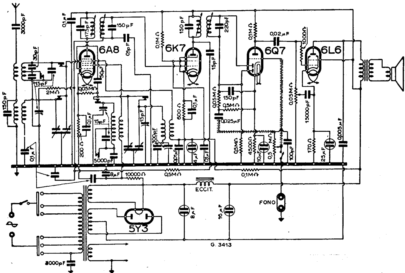
RADIO SUPERLA - MODD. « 531 » « 1531 »
