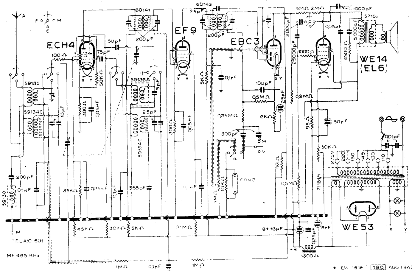
Il mod. « V. d. P. 571 Fono ».
