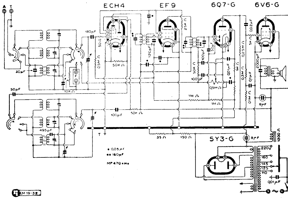
MINERVA - MOD. « 475/4 »
