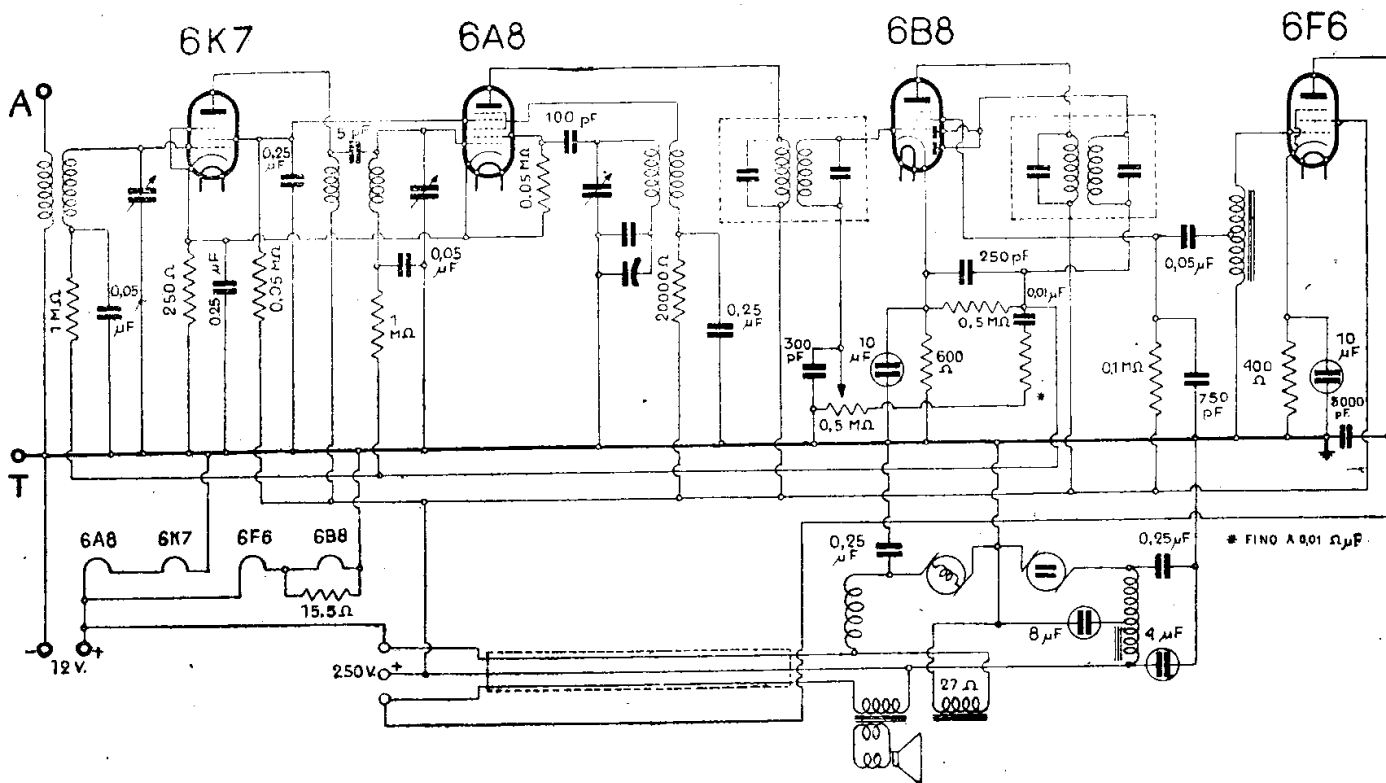
IRRADIO - MOD. « A 43 » - « AA 43 » AUTORADIO
