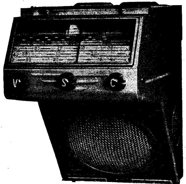
Il Condor « Cyclone Six » autoradio.
