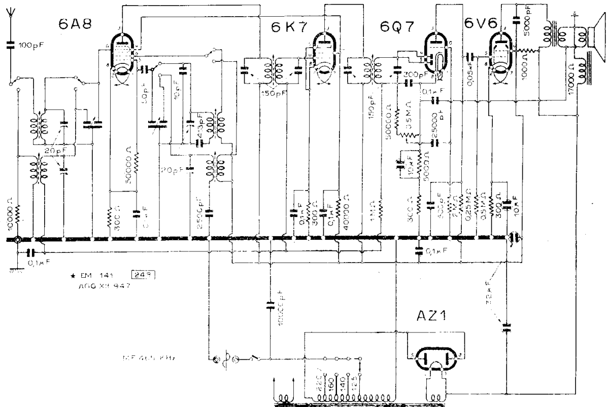
ALLOCCIO, BACCHINI &amp; C. - MOD. « 514 »
