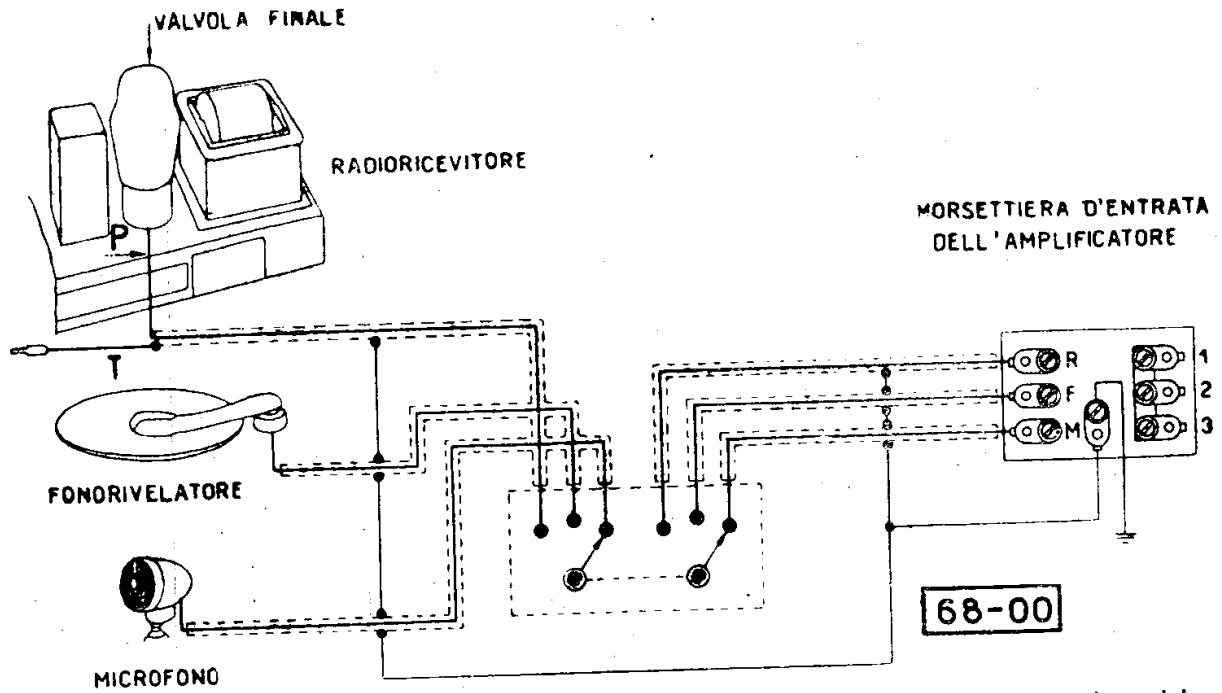
Il collegamento negli amplificatori Magneti Marelli descritti in questo paragrafo, della « Radio », del « Microfono » e del « Fonorivelatore ». Un invertitore a doppio contatto e tre posizioni provvede alla commutazione dei tre elementi.
