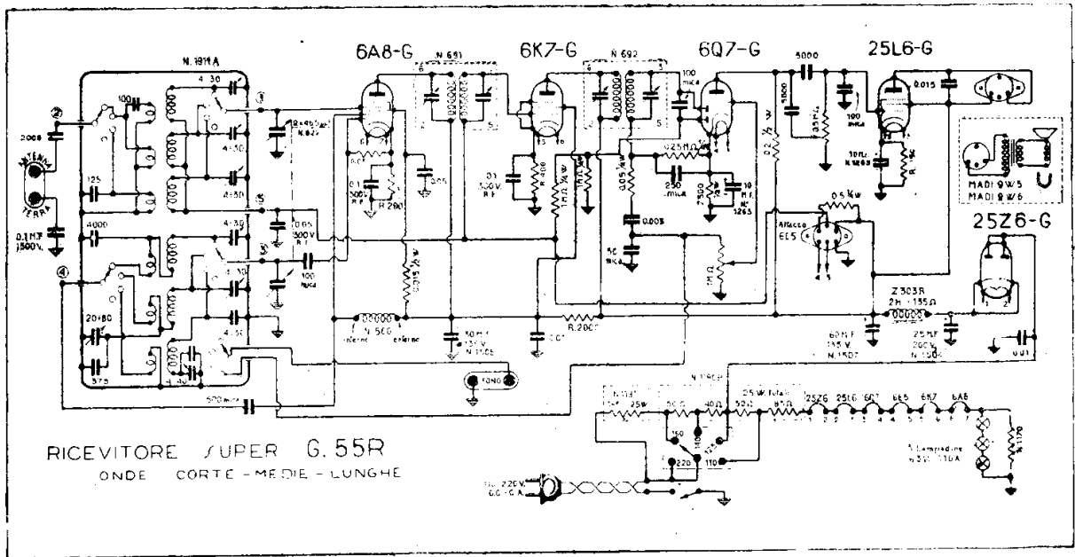
GELOSO (SOC.) - MOD. SUPER « G 55 R »
