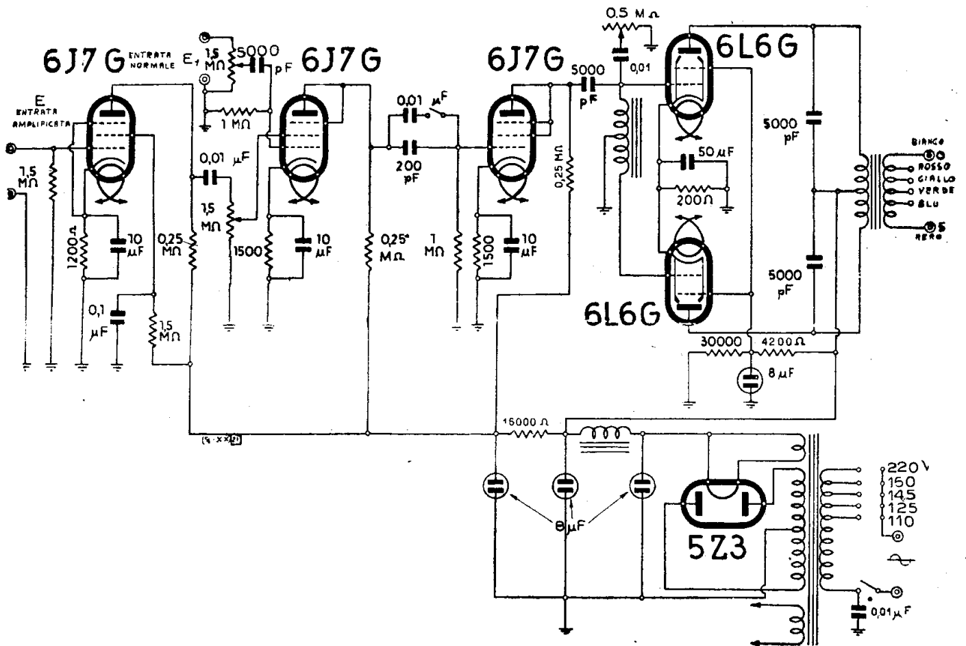
NOVA - AMPLIFICATORE MOD. « 32 W »
