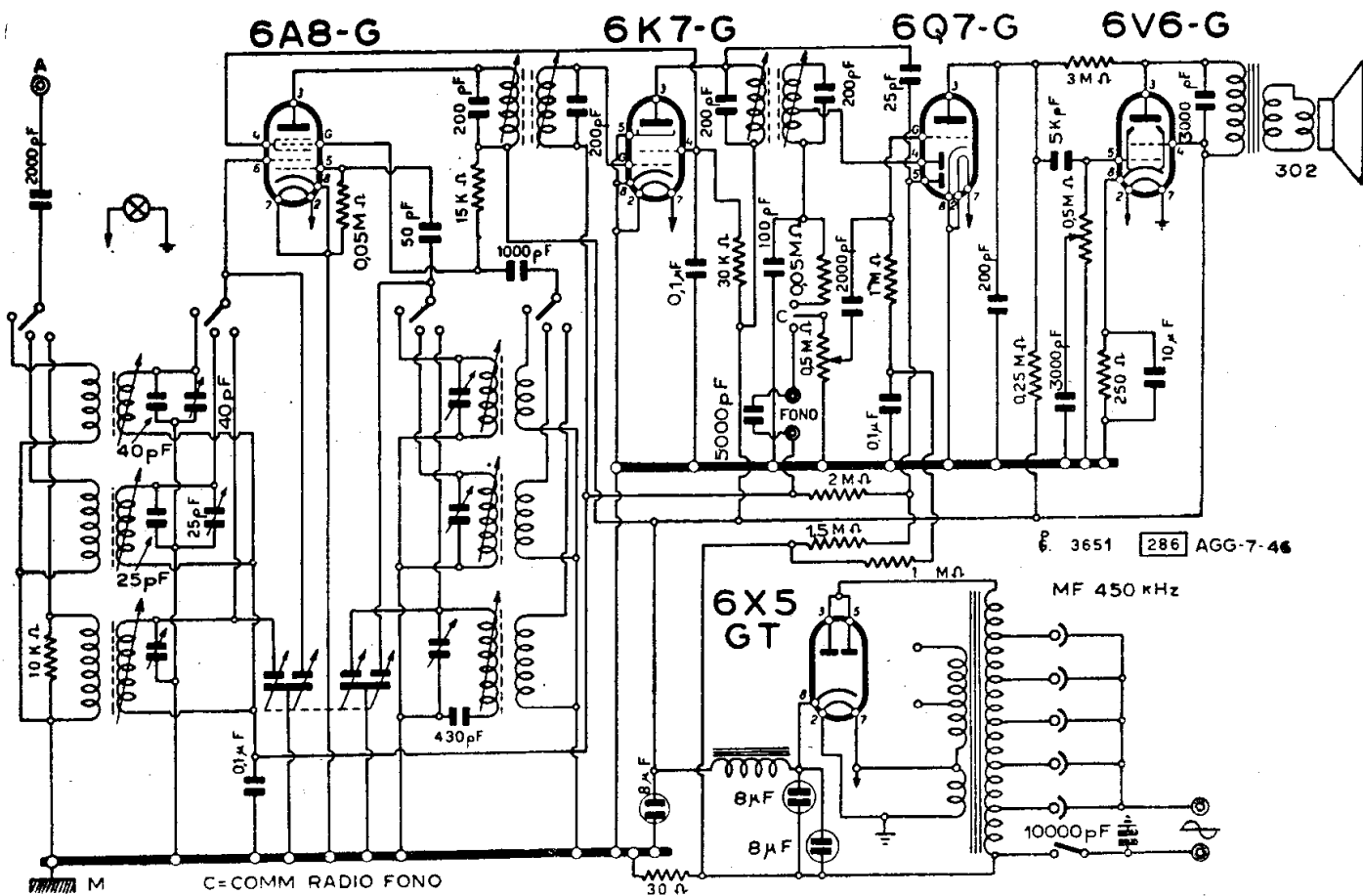
UNDA RADIO - MOD. « TRI UNDA R 53/4 »
