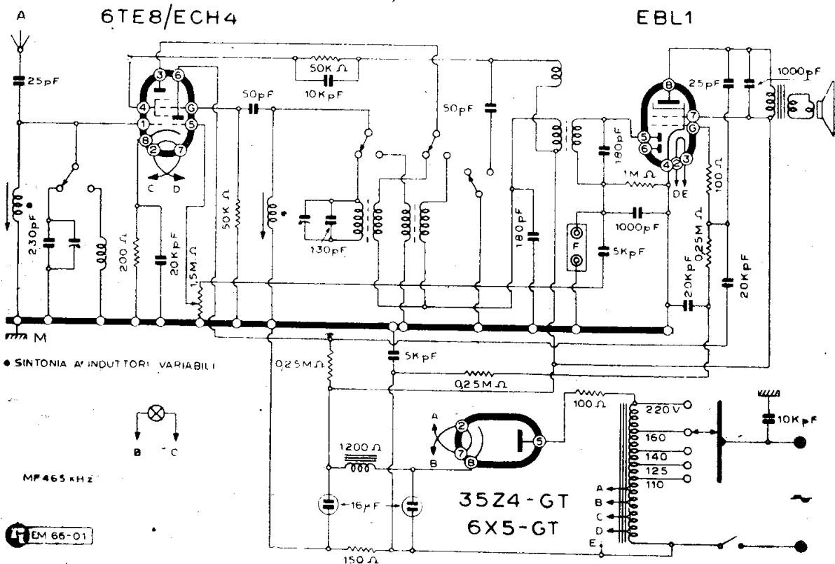
A.B.C. RADIO COSTRUZIONI - MOD. « R 731 »
