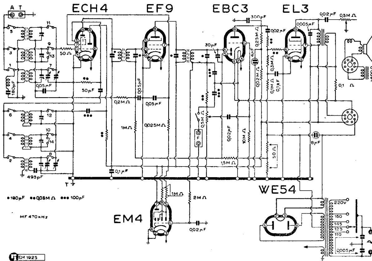
MINERVA - MOD. « 455/3 »
