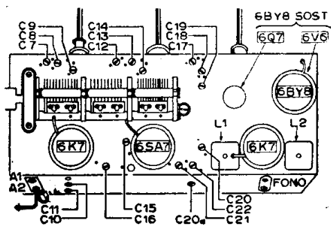
Il mod. « Nilo Bianco »: Il telaio con la posizione dei compensatori.
