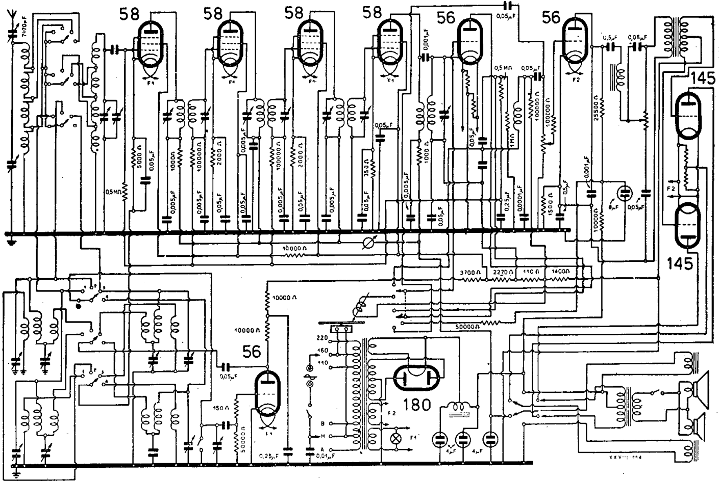
RADIOMARELLI - MODD. « ARGESTE » « FONARGESTE »
