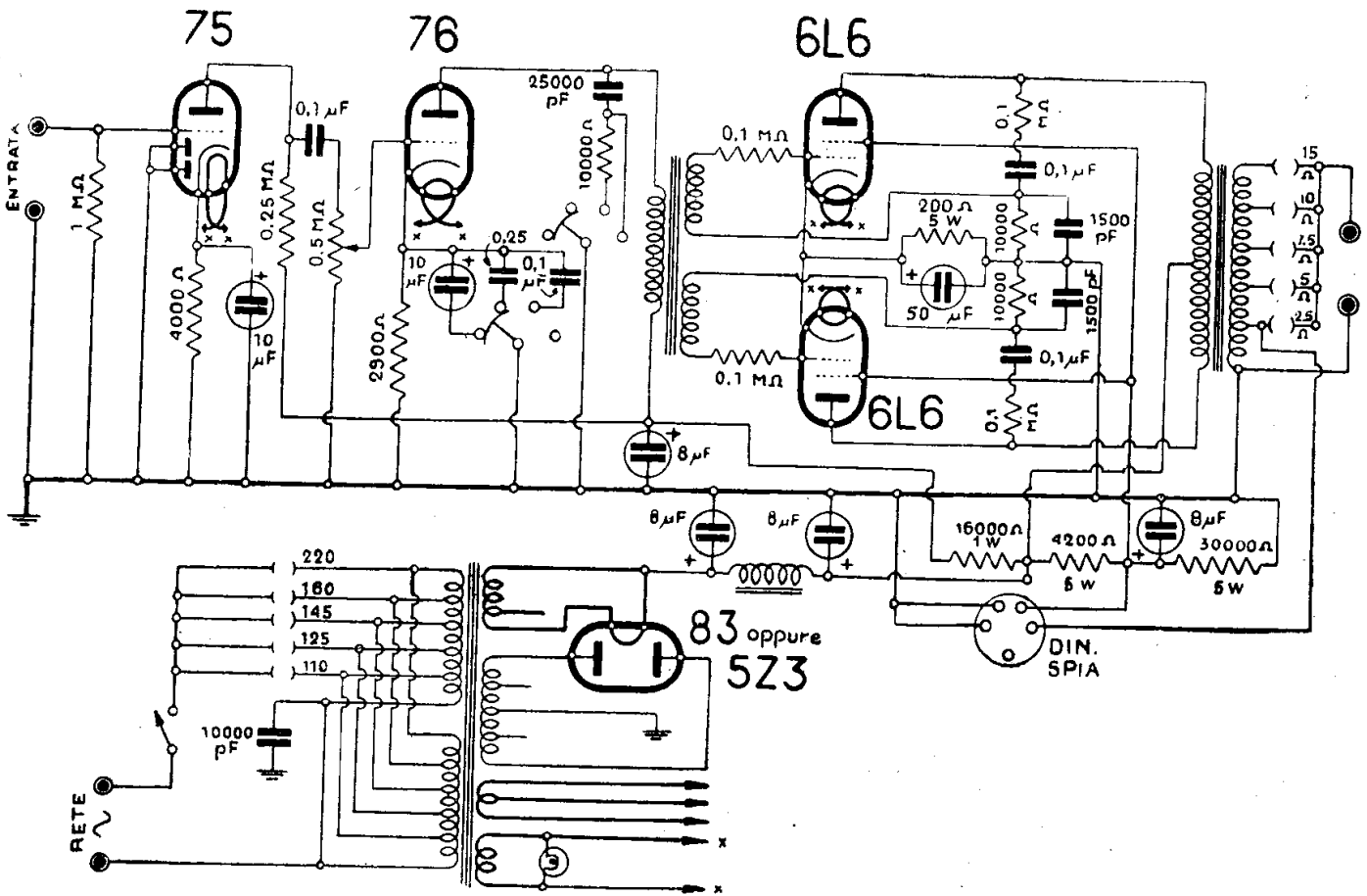
NOVA - AMPLIFICATORE MOD. « 24-30 W »
