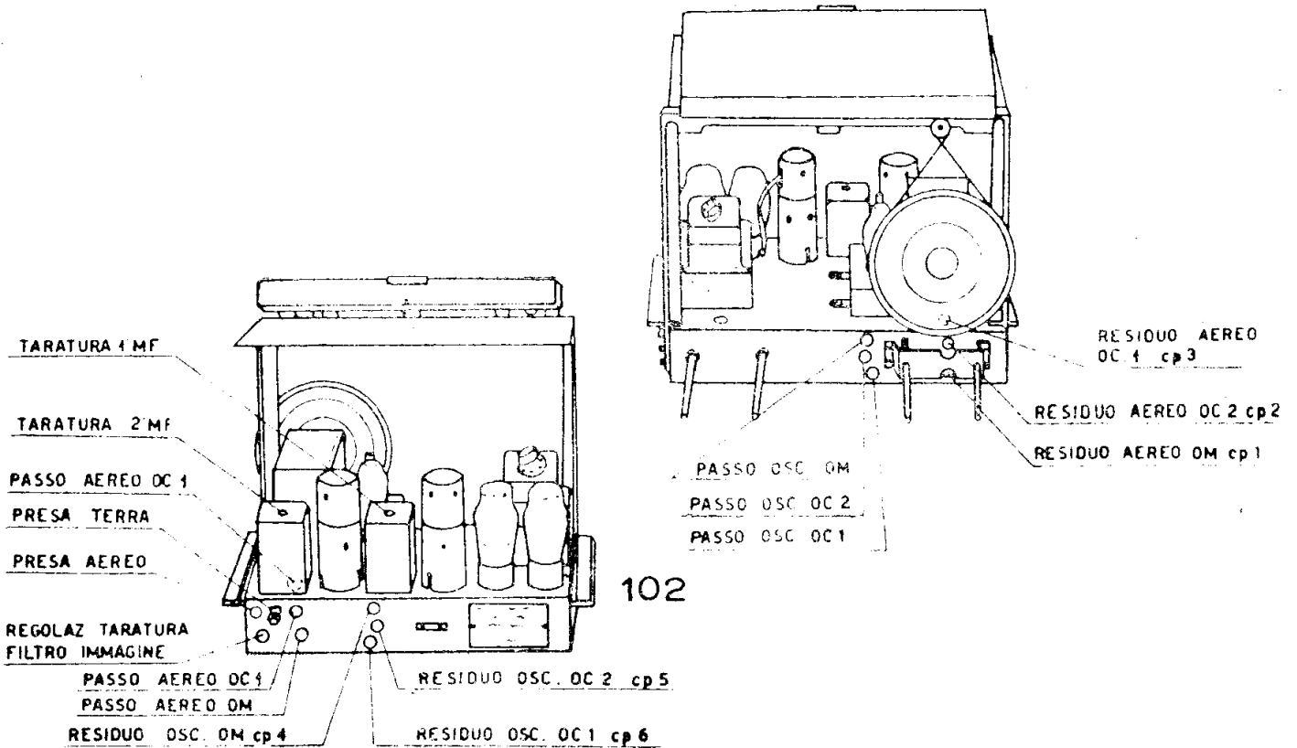
Disposizione dei compensatori per la taratura sull'AF e la MF del « 520 ».
