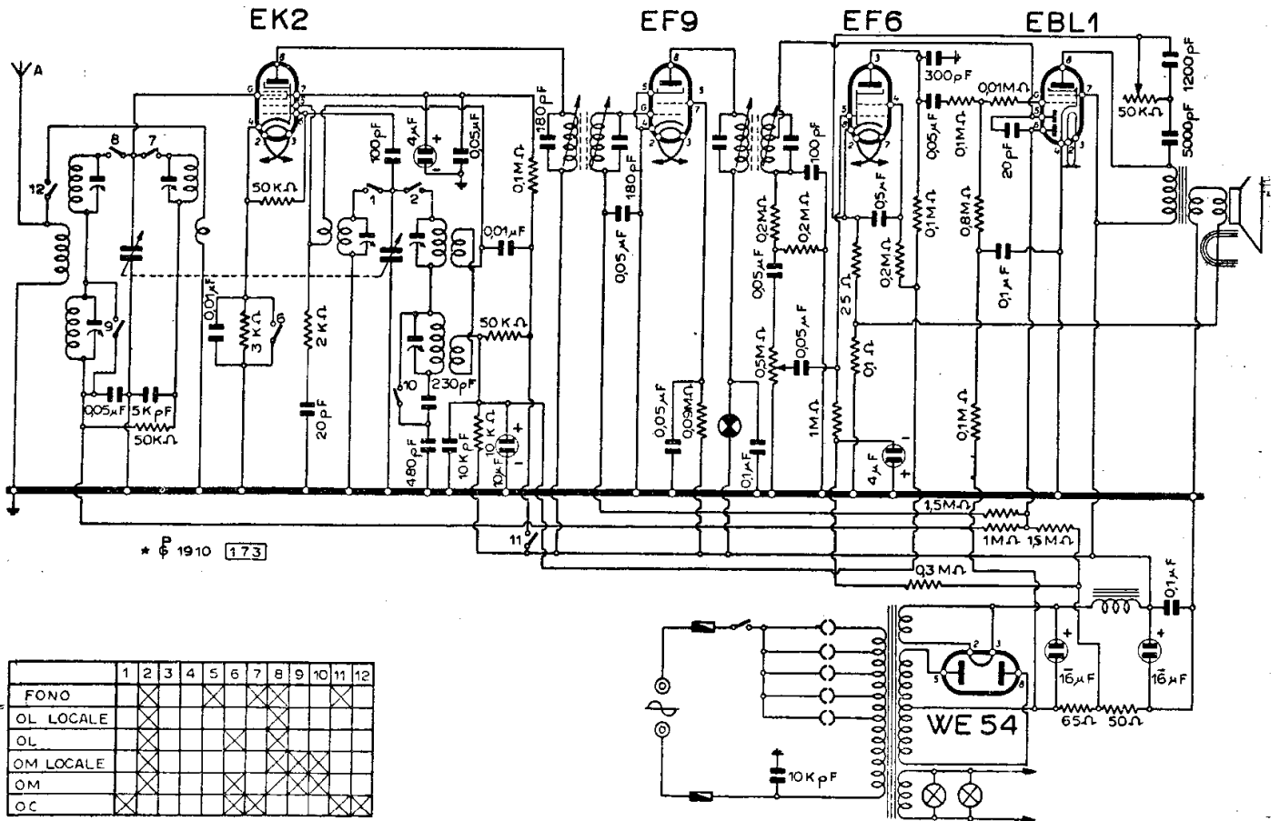
MINERVA - MOD. « 385 »
