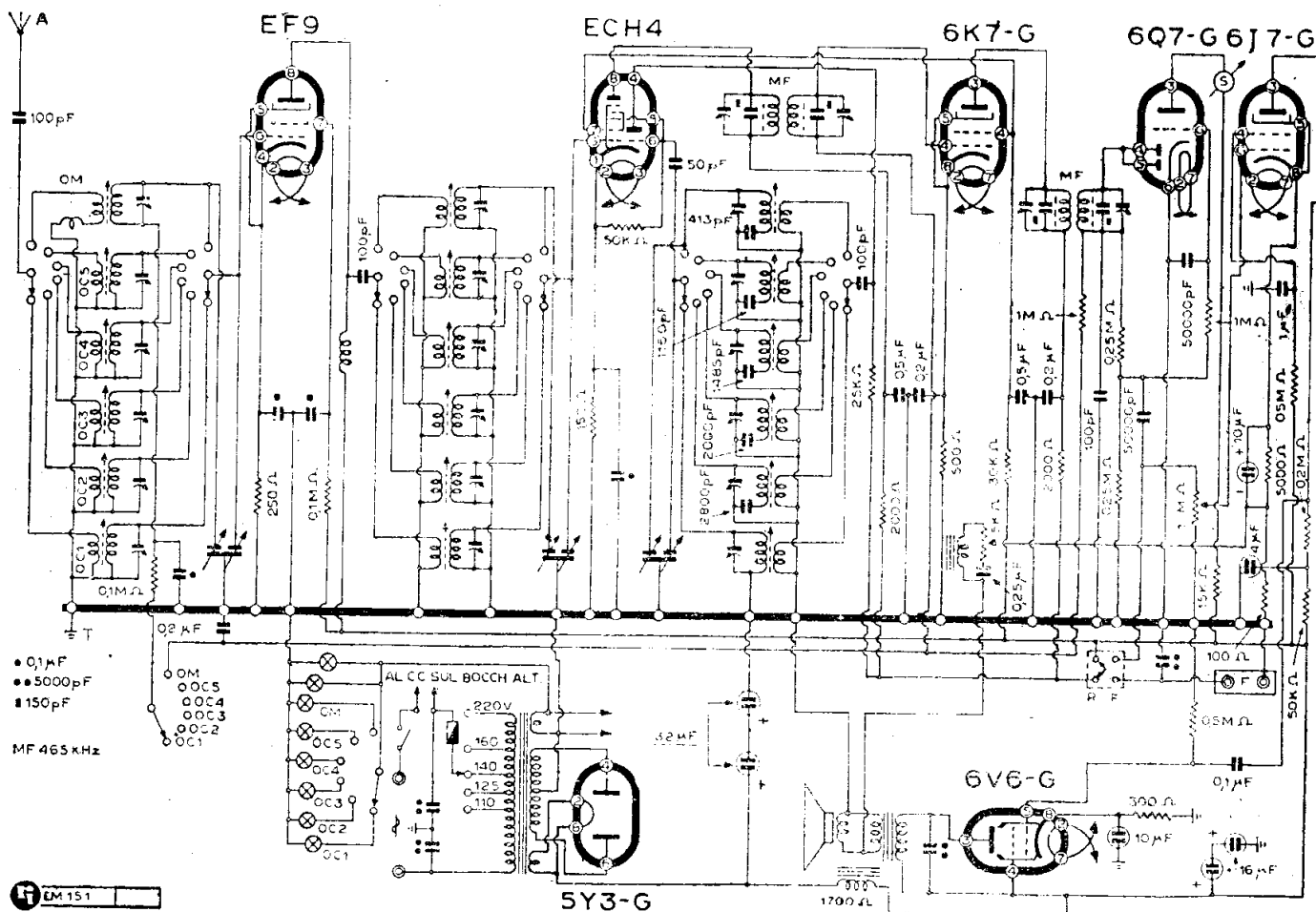
ALLOCCIO, BACCHINI & C. - MOD. « 716 »
