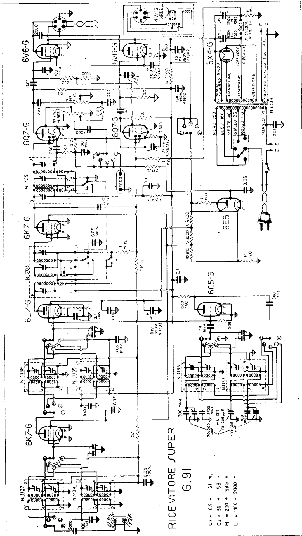
GELOSO (SOC.) - MOD. SUPER (G.91)
