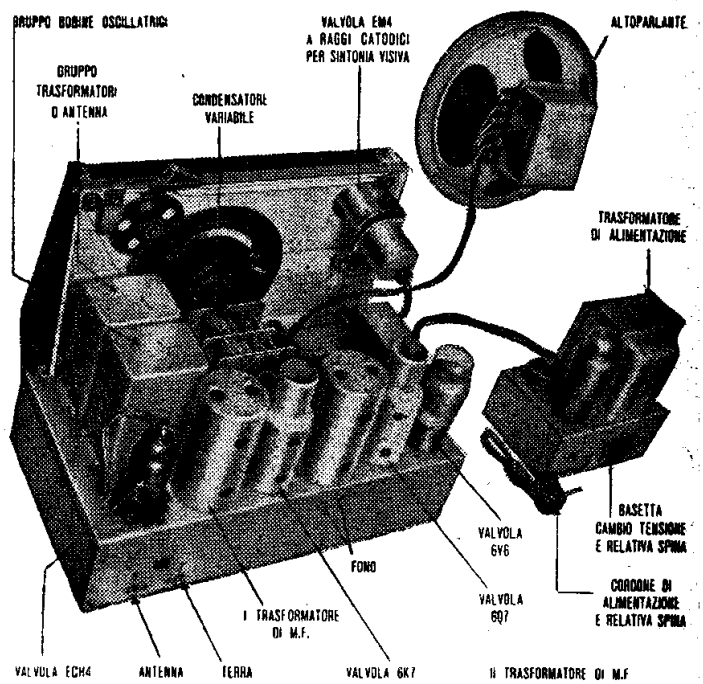
Il telaio del mod. « 315 » visto posteriormente.
