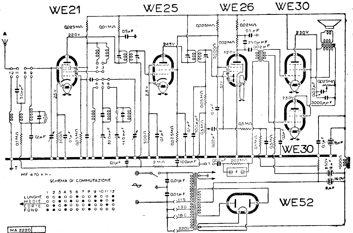
RADIO LAMBDA - MOD. « E 646 »
