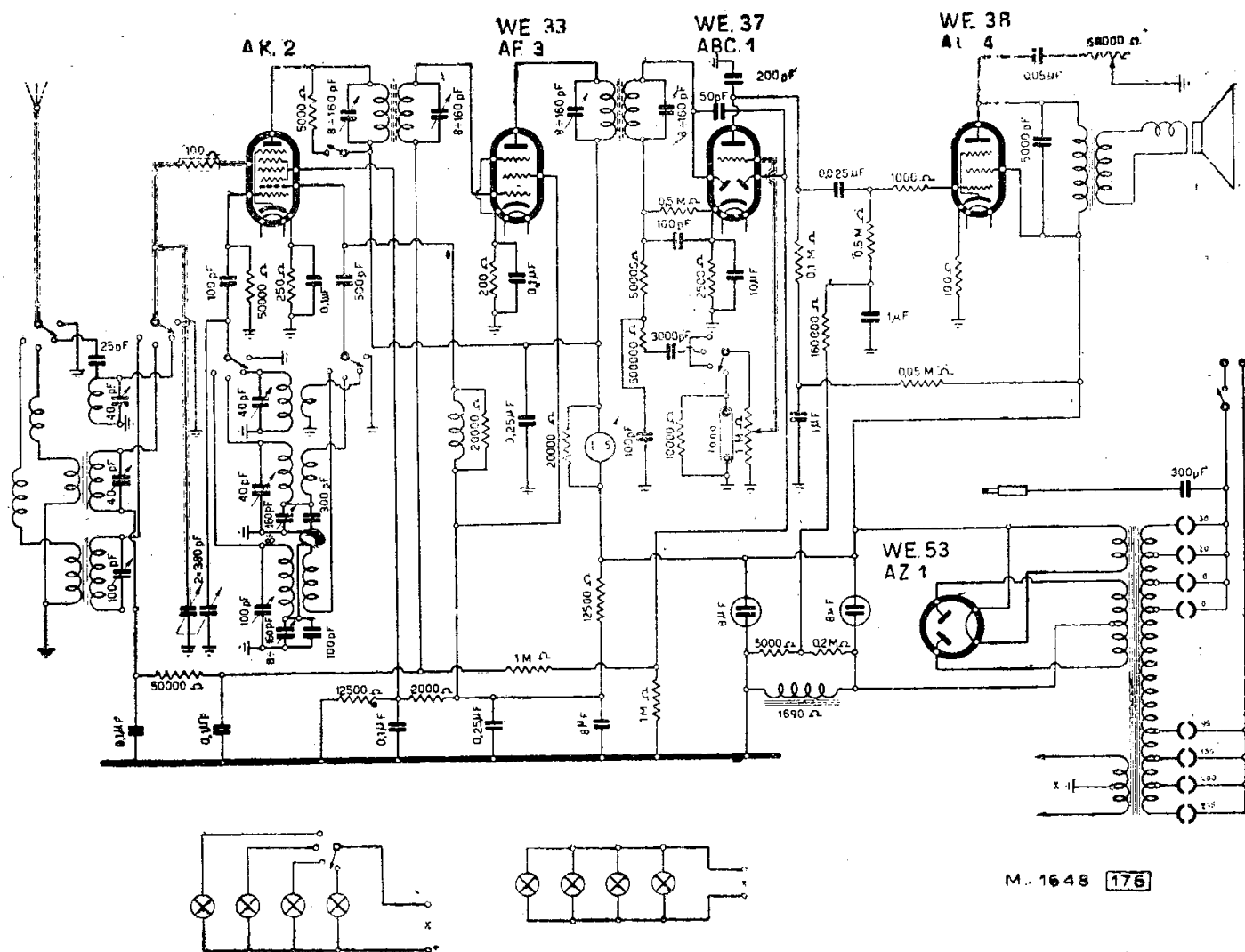
LA VOCE DEL PADRONE - COLUMBIA - MARCONIPHONE MODD. « V. d. P. 514 » e « 516 FONO »
