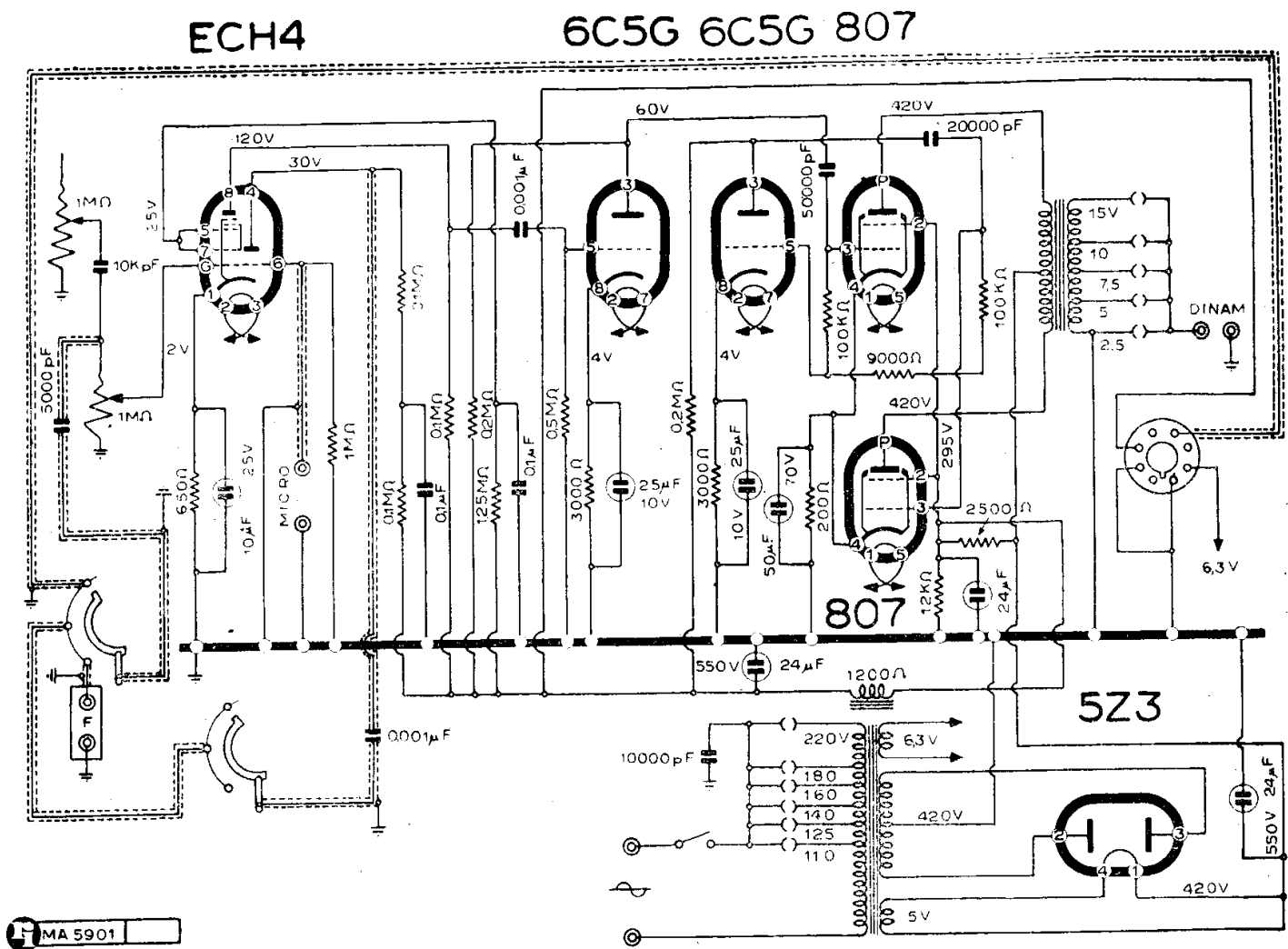
L.I.A.R. - AMPLIFICATORE MOD. « 25 A 5 »
