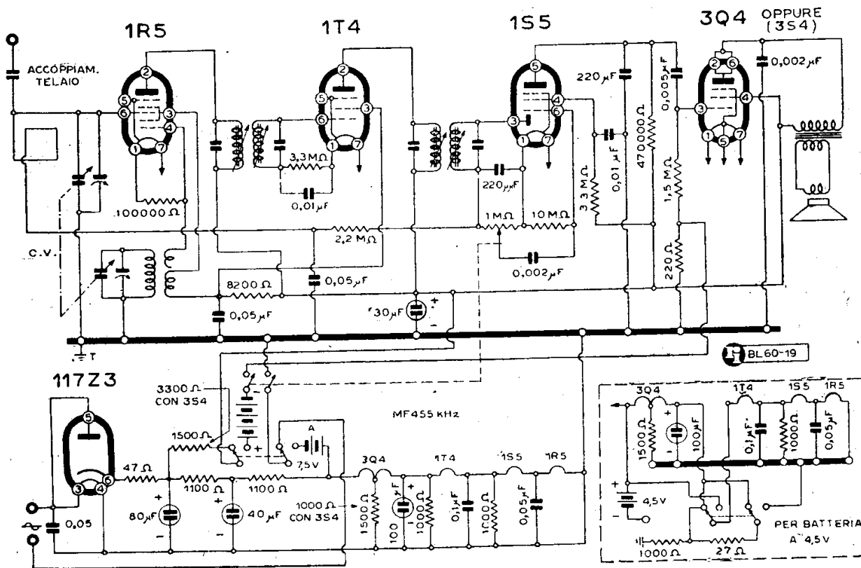
EMERSON - MOD. « 559 »
