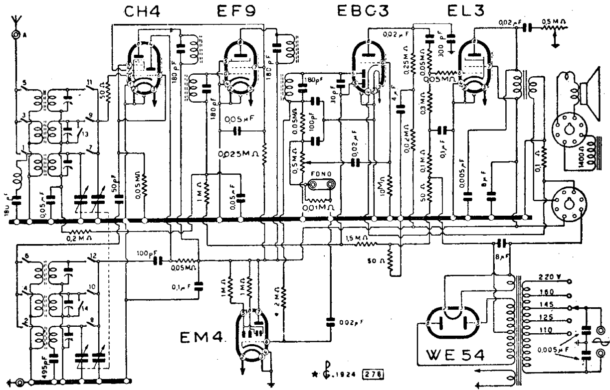
MINERVA - MODD. « 445/3 » « 1455/3 RF »
