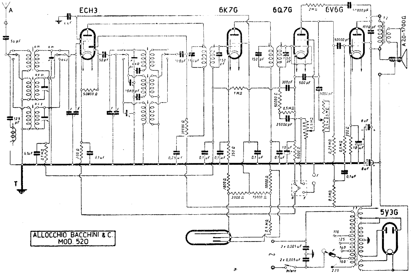
ALLOCCIO, BACCHINI & C. - MOD. « 520 »
