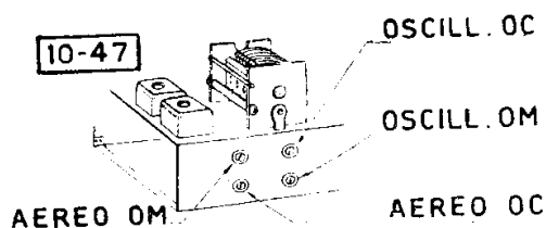
La posizione dei compensatori per i modd. « 407 » e « 407-A ».
