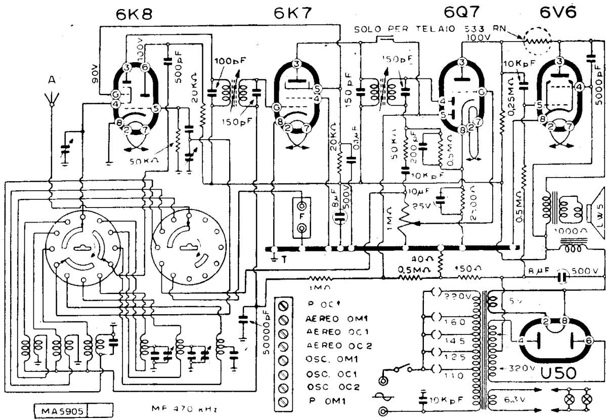
L.I.A.R. - MOD. « 535 »
