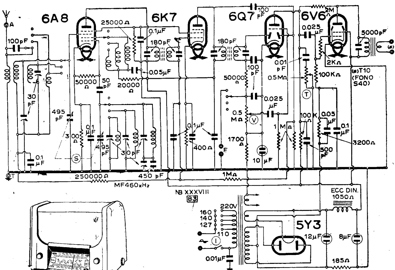
WATT RADIO - MOD. « SUPER STELLA II »
