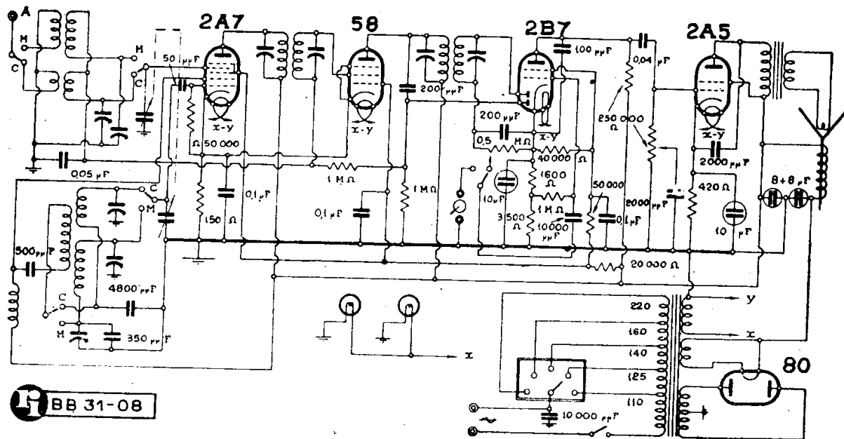
S.I.A.R.E. CROSLY - MOD. « 154 »
