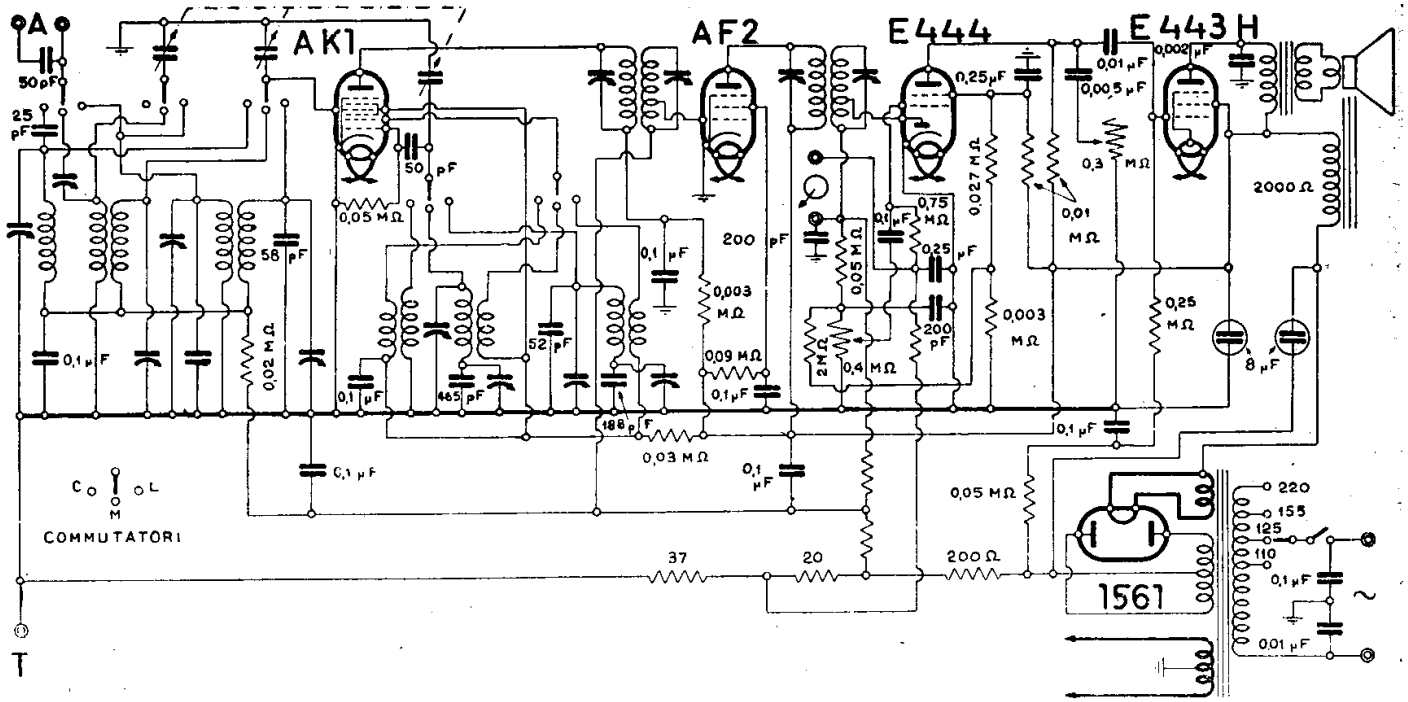
MAGNADYNE - MOD. « S 53 »
