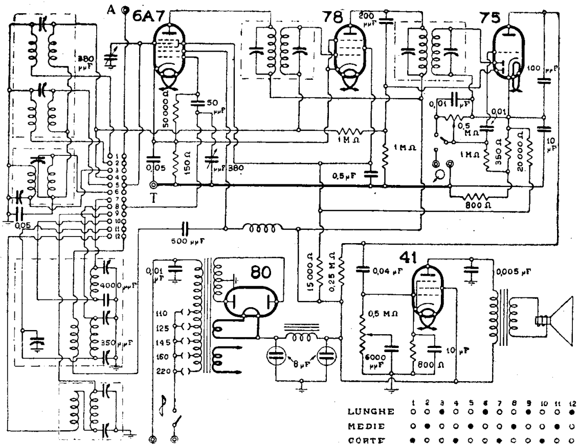
OFFICINE DI SAVIGLIANO - MOD. « 73 »
