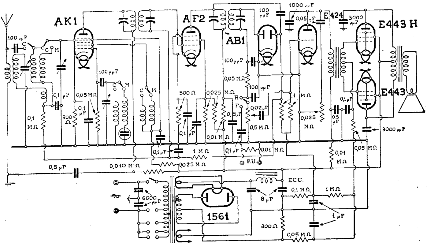
RADIO LAMBDA - MOD. « E 427-C.M. »
