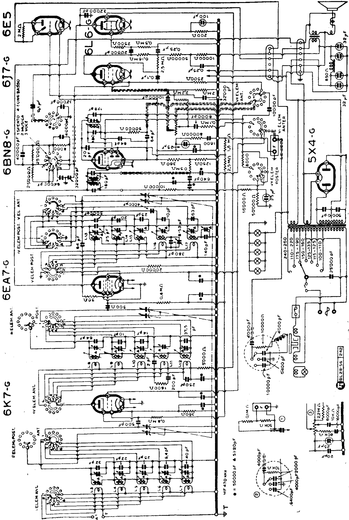
RADIOMARELLI - MOD. « 9F36 »
