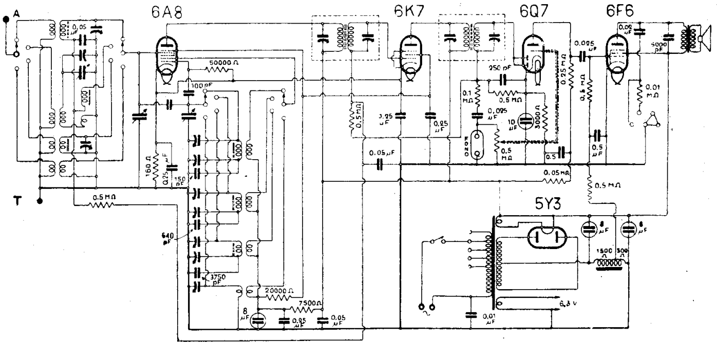
IRRADIO - MOD. « D 57 » « D 557 »
