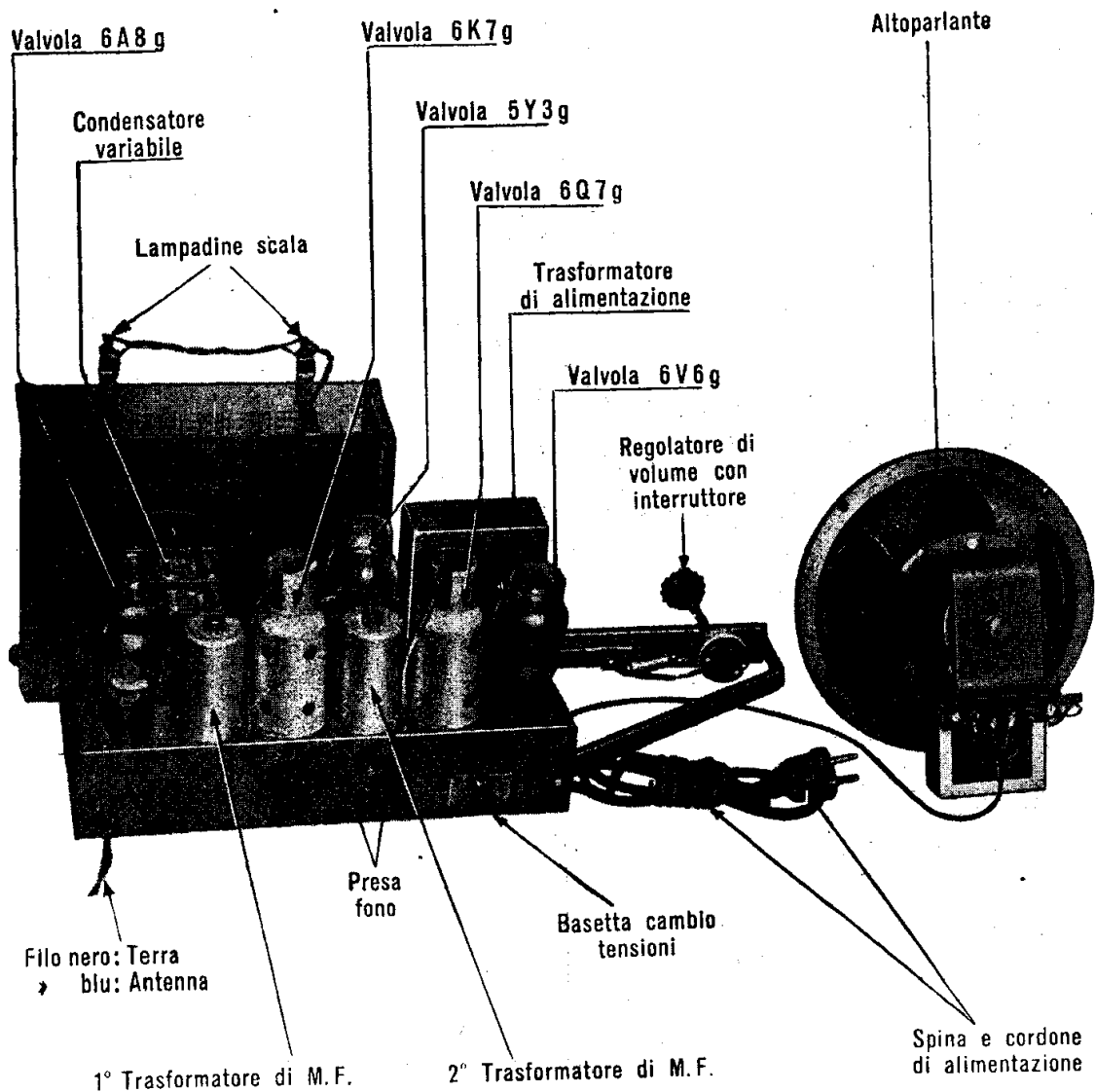
Il mod. « 865 » radiofonografo: vista posteriore.
