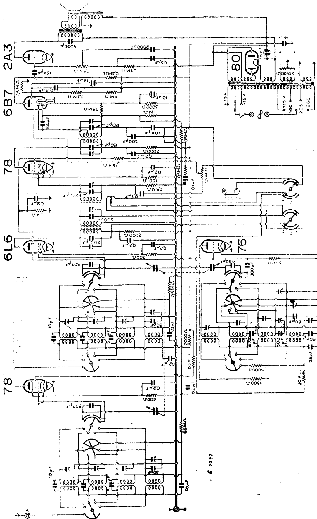
S.A.F.A.R. - MOD. - « 748 »
