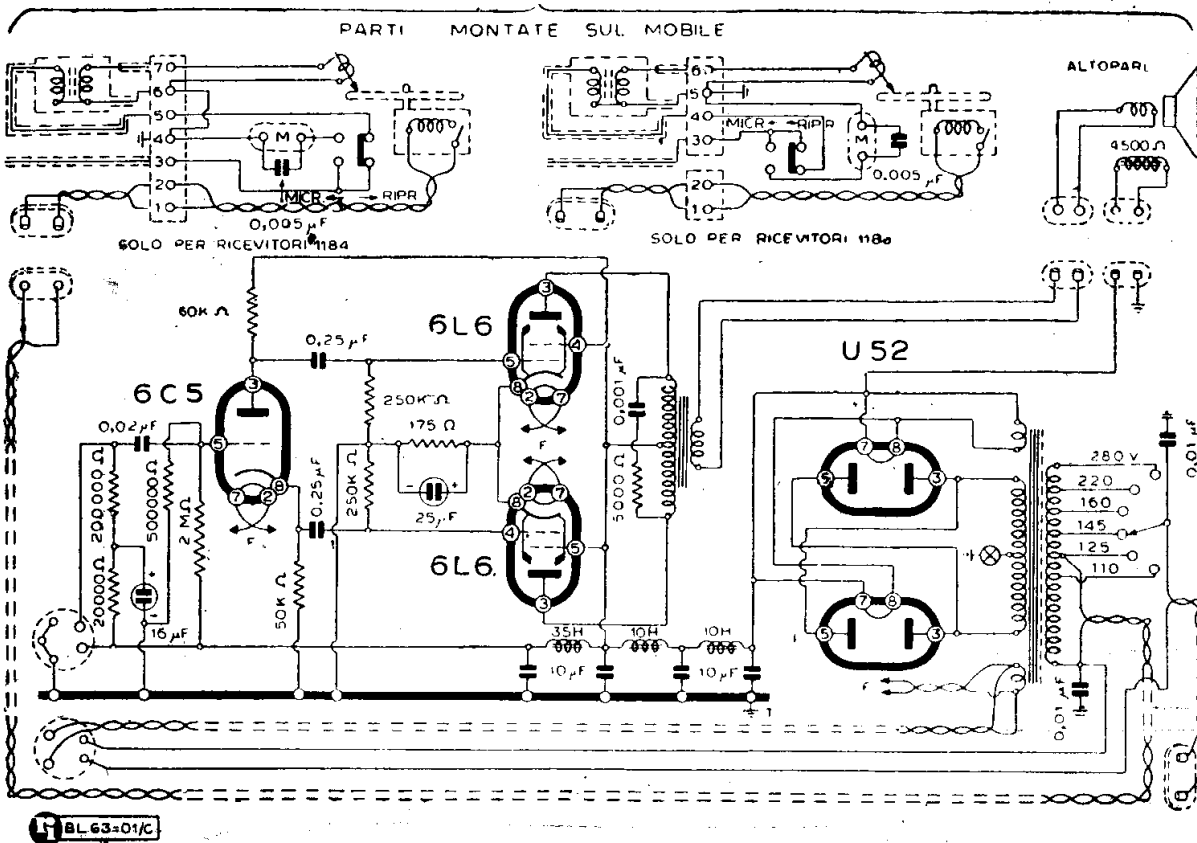
COMP. IT. MARCONI - MODD. « 1183 » « 1184 » PARTI BF E ALIM.
