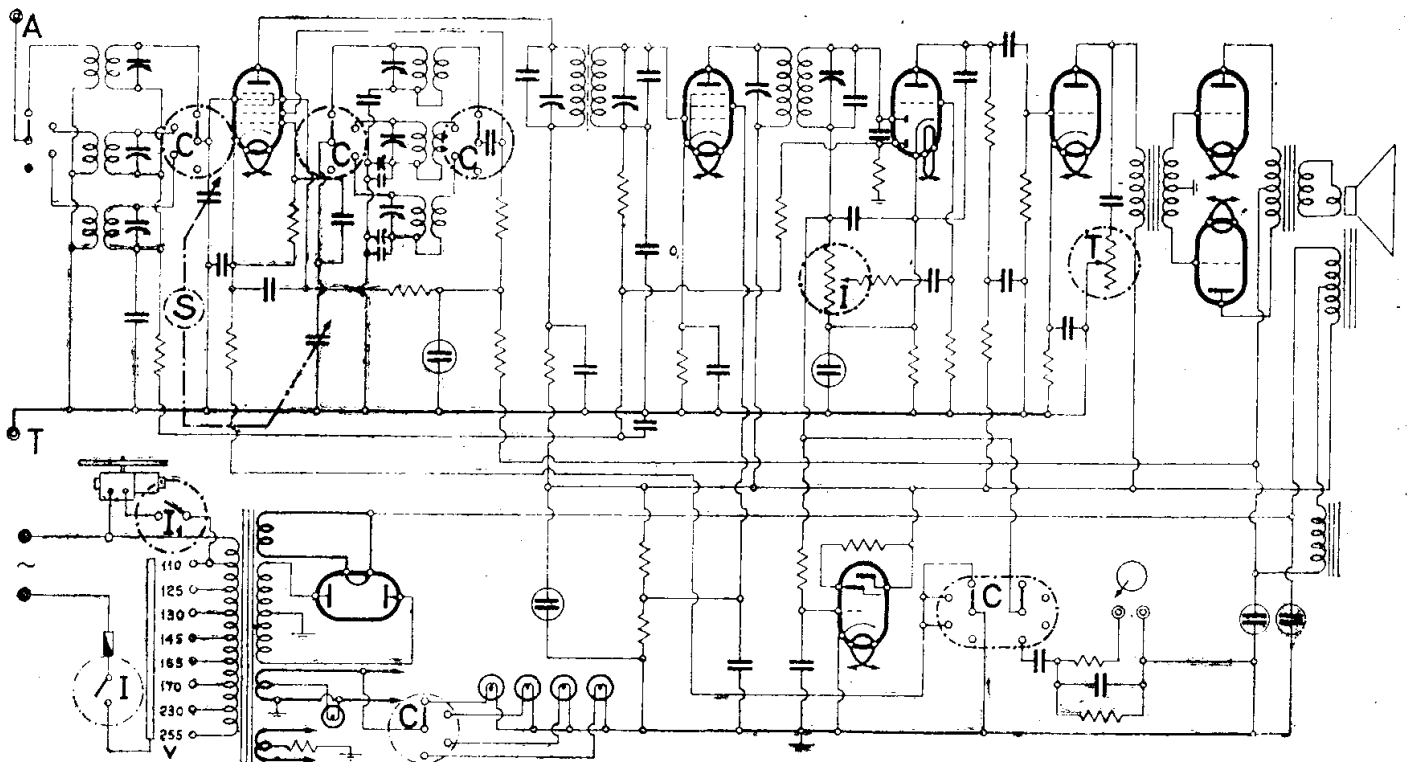
COMPAGNIA GENERALE DI ELETTRICITA' - MODD. « 252 » « 253 » « 263 »
