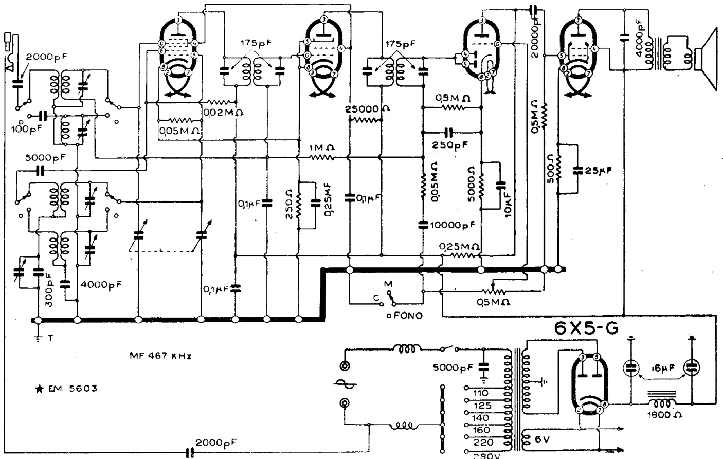
OREM - MOD. « 522 »
