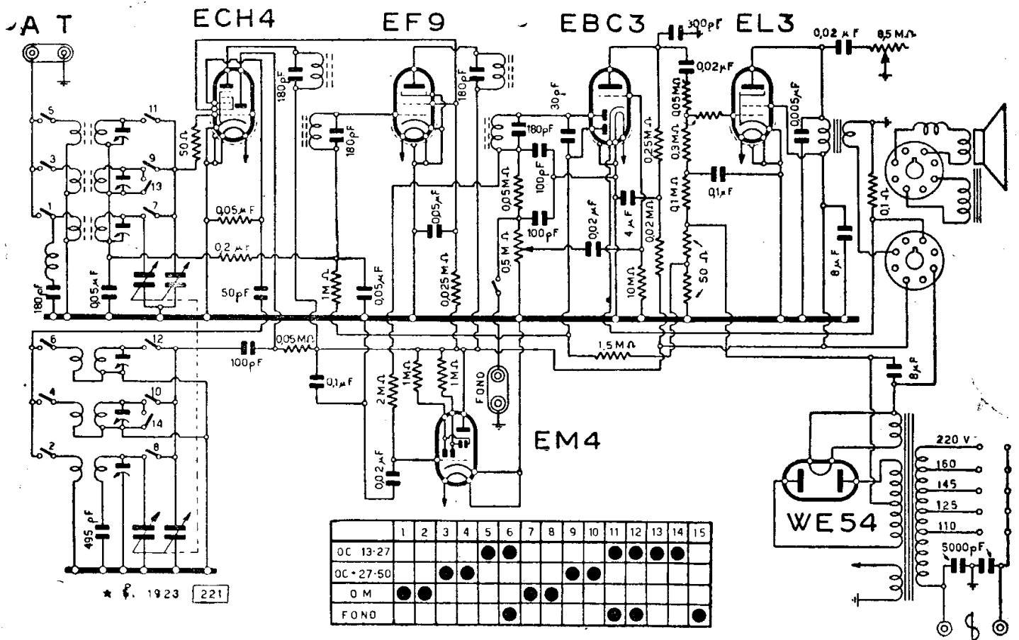
MINERVA - MOD. « 4451 »
