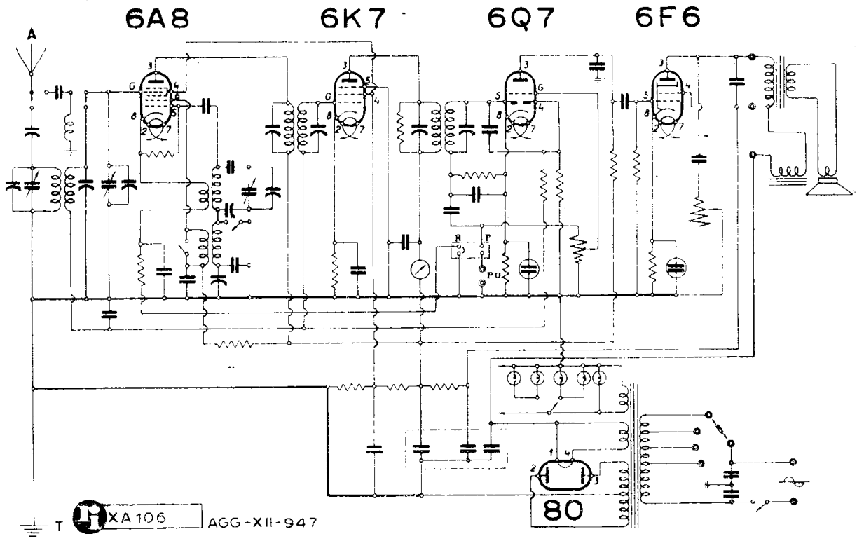
ALLOCCHIO, BACCHINI & C. - MOD. « 55 »
