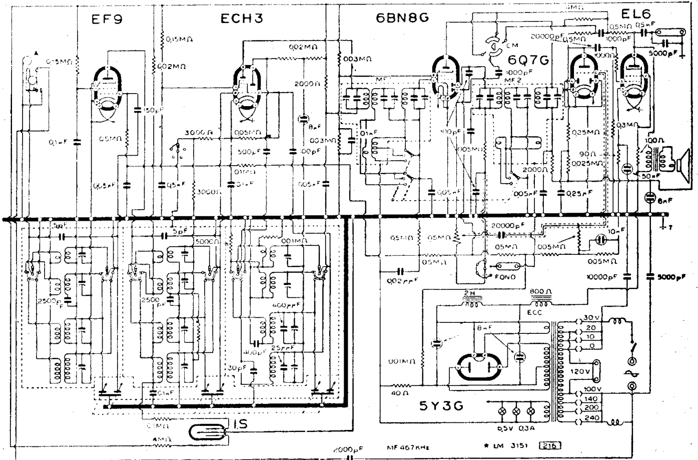
S.I.A.R.E. - MOD. « 461 A »
