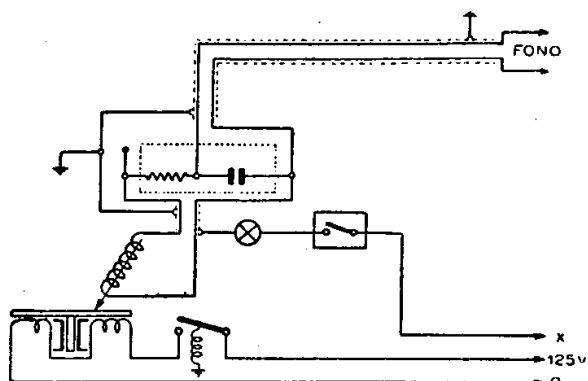
Il tipico collegamento per le varianti Fono (pik-up elettromagnetico).
