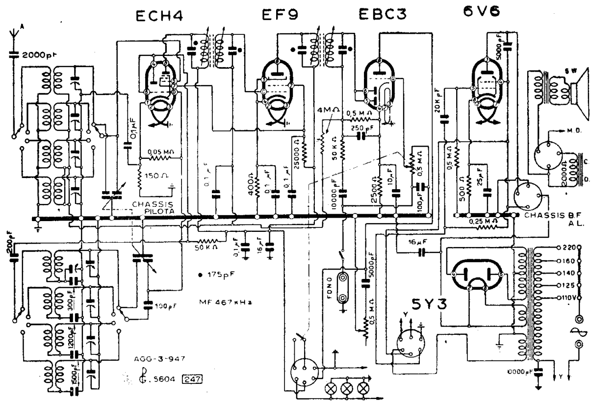
OREM - MOD. « 543 »
