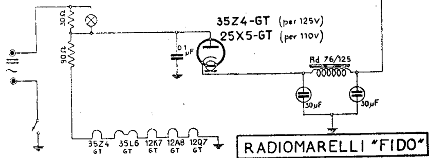
RADIOMARELLI - MOD. « FIDO »
