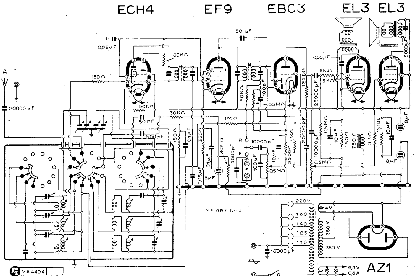
INCAR - MOD. « LV 52 »
