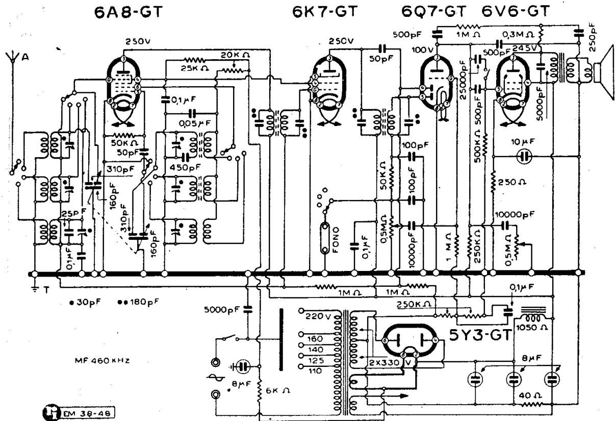
WATT RADIO - MOD. «TAURUS ORO III»
