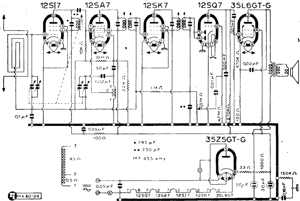
MANTOLA - MODD. « 92505 » « 92506 »
