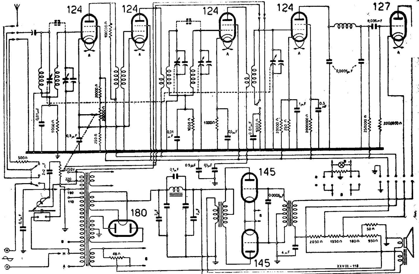
RADIOMARELLI - MOD. « CHILIOFONO I »
