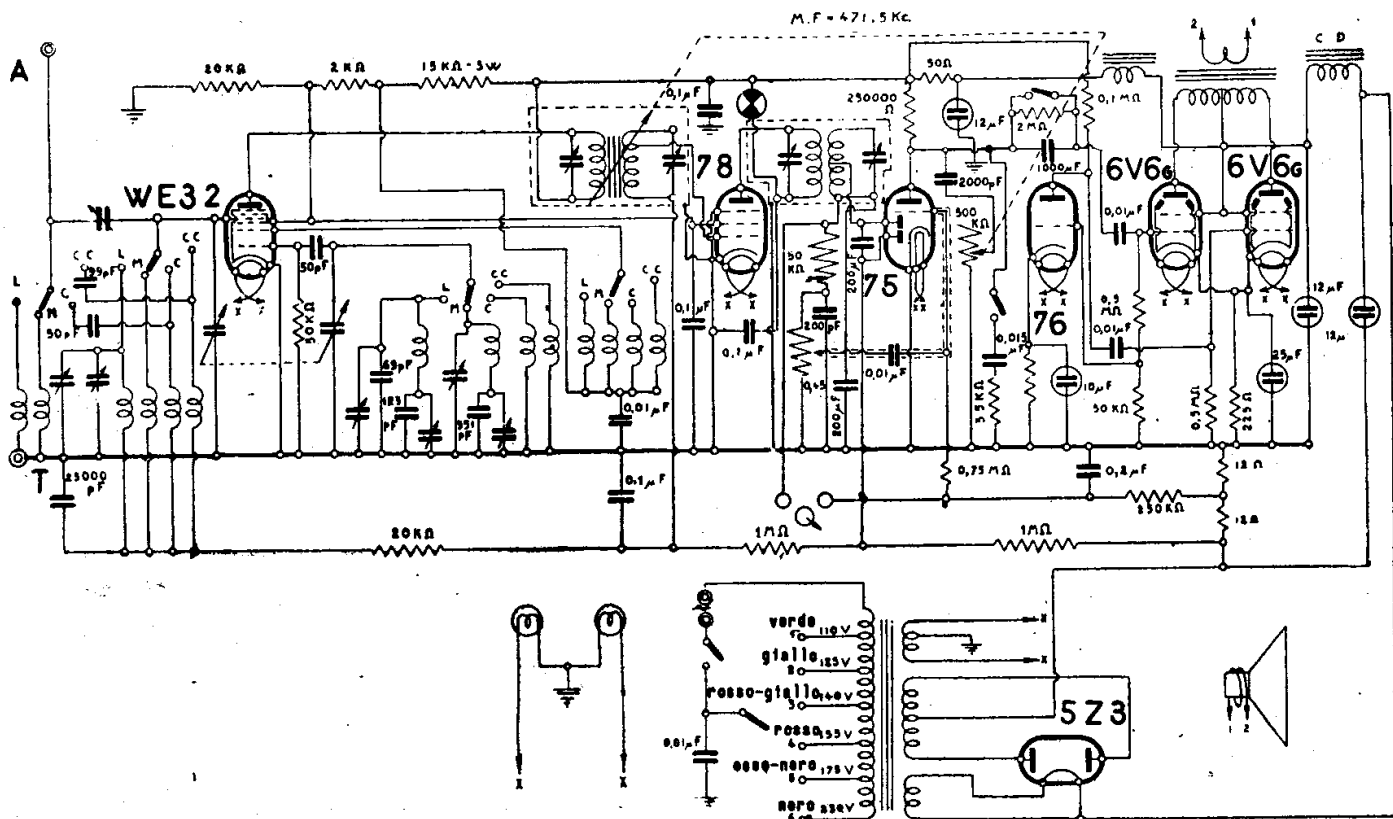
MAGNADYNE - MOD. « SV 74 » « SV 174 »
