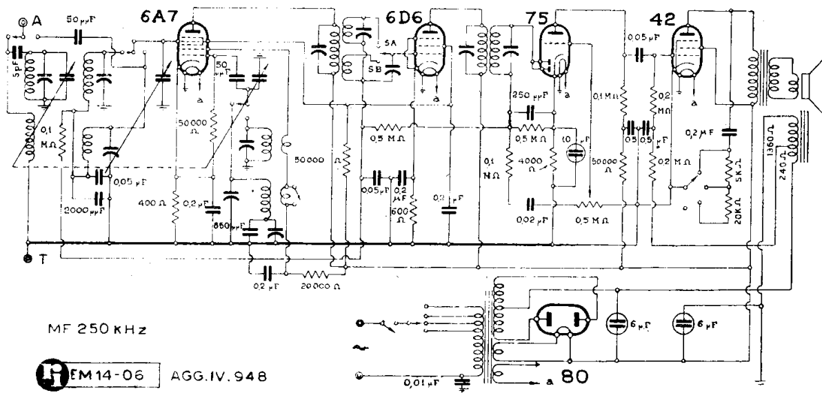
IRRADIO - MOD. « B 50 »
