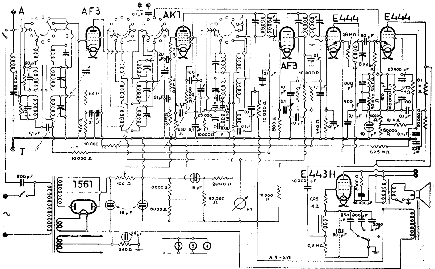
PHILIPS RADIO - MOD. « 532 A » — POPE RADIO - MOD. « P. 67 »
