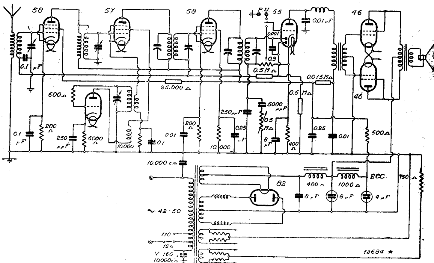
CRESA RADIO - MOD. « SUPERLA 8 CA »
