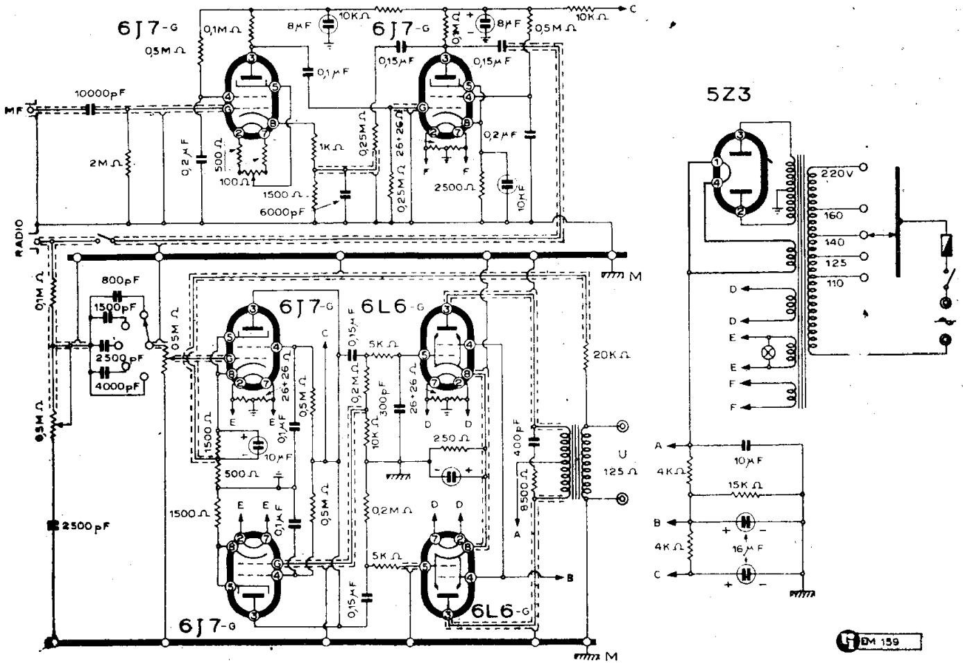
ALLOCCIO, BACCHINI &amp; C. - AMPLIFICATORE MOD. « 2516 »
