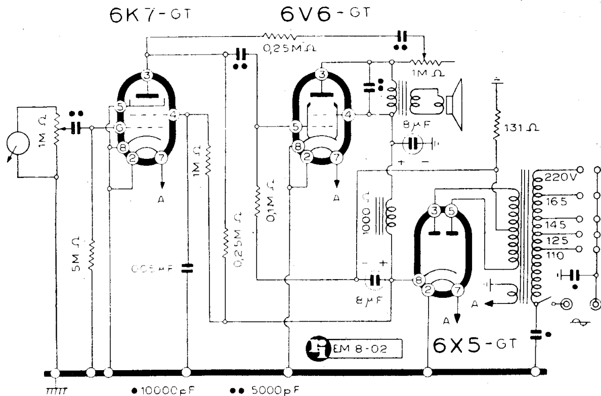
DURIUM S. A. - MOD. « DURIOLA 480 »
