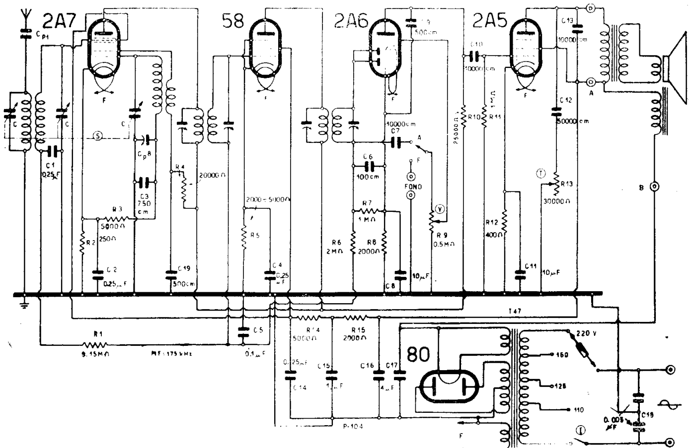
ALLOCCIO, BACCHINI & C. - MOD. « 53 c.a. »
