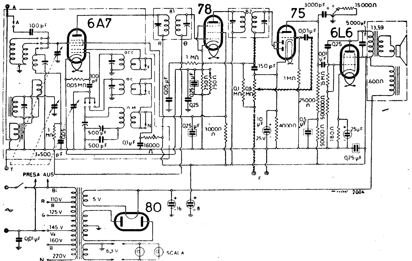
NOVA - MOD. « 501 »
