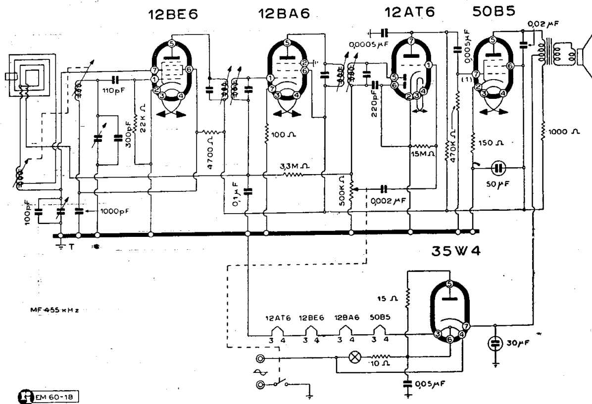
EMERSON - MODD. « 540 » « 564 » « 572 »
