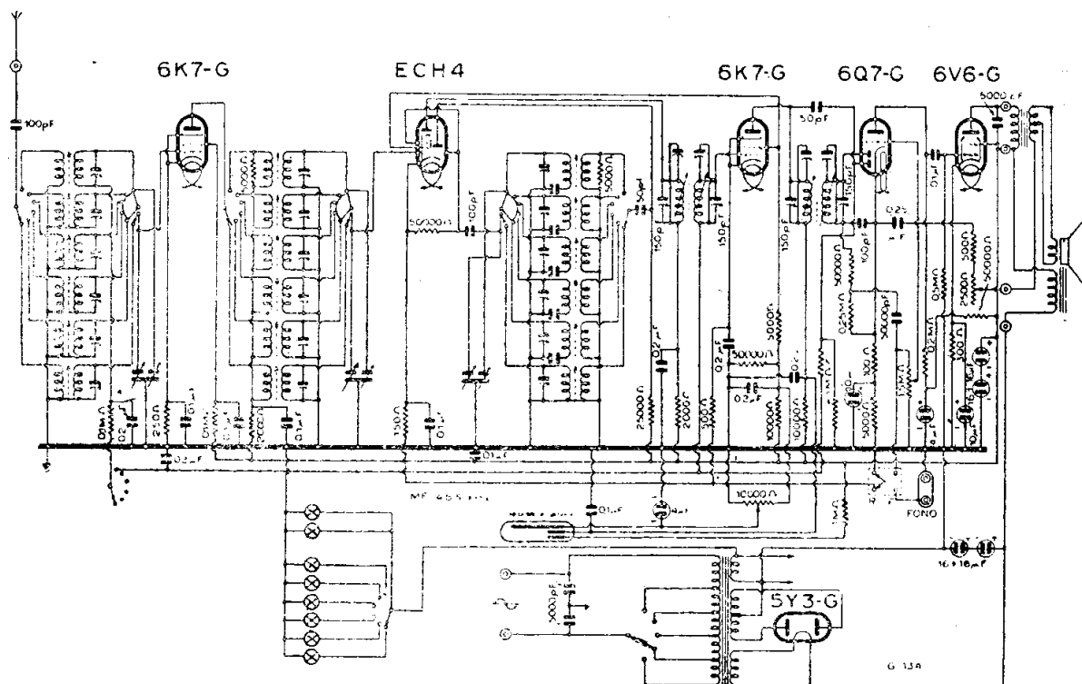
ALLOCCIO, BACCHINI &amp; C. MOD. « 612 »
