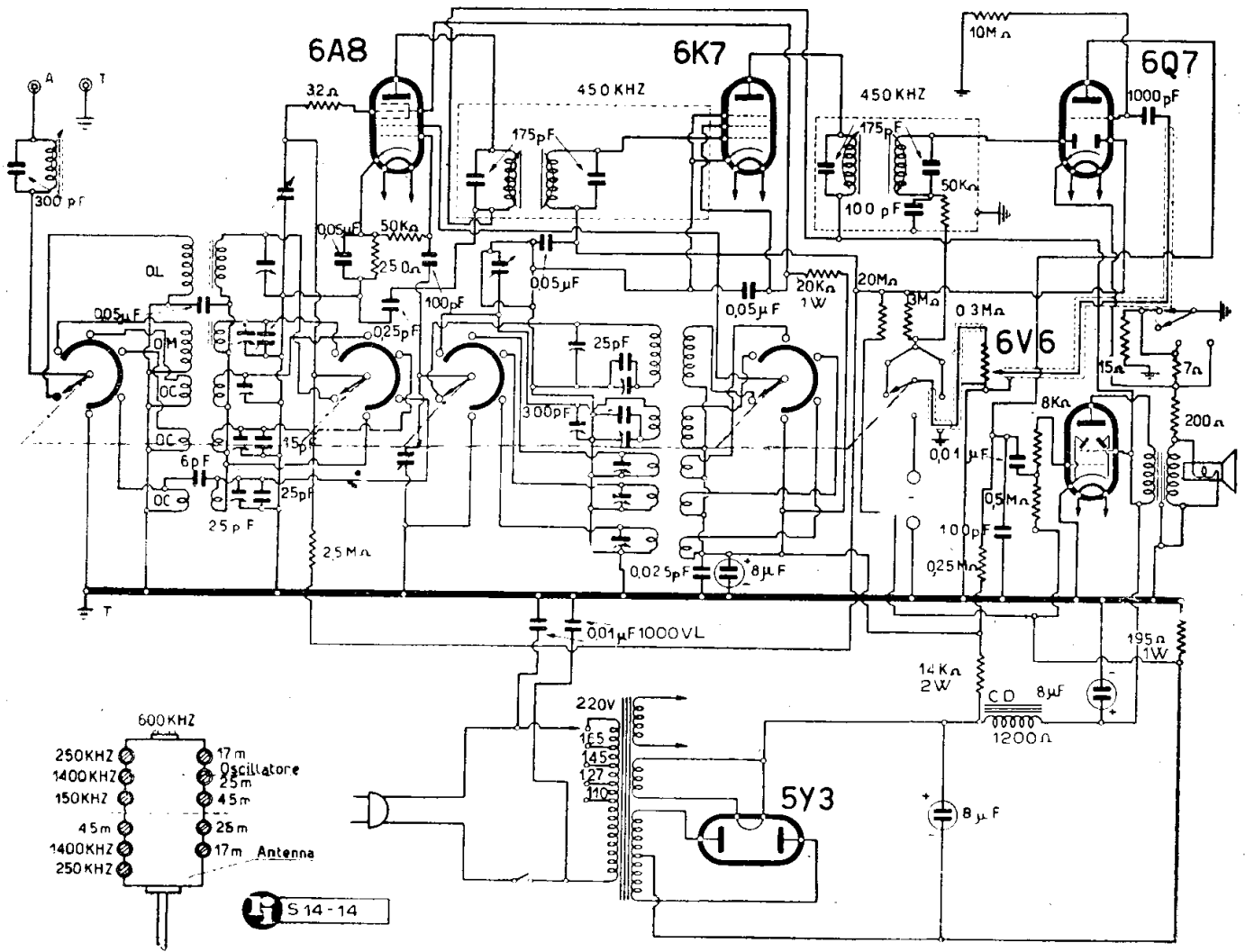
DURIUM S. A. - MOD. « D 1625 FONO »
