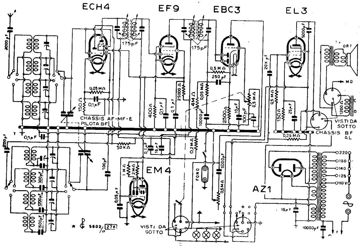
OREM - MOD. « 642-R »
