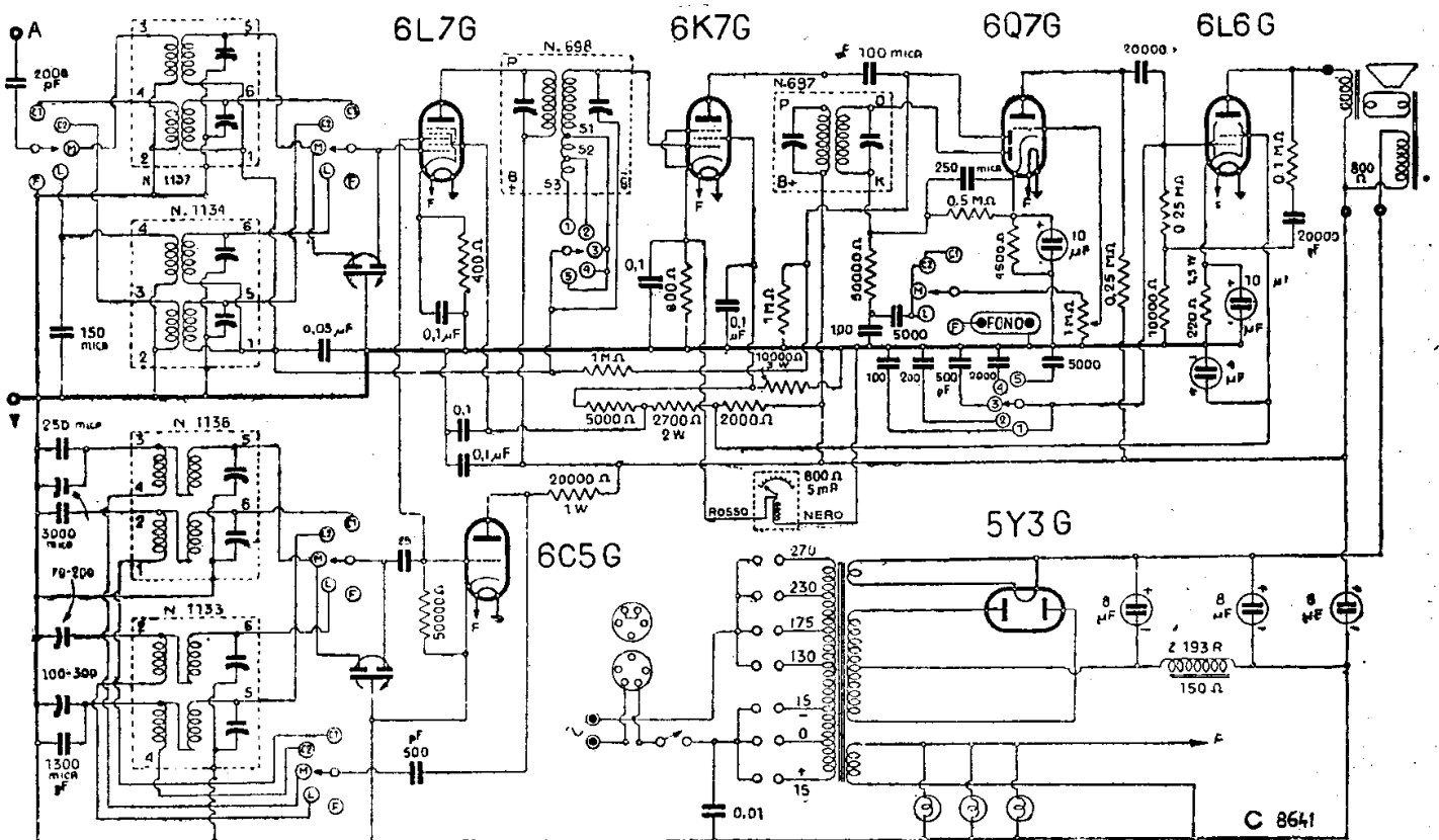
S.I.A.R.E. - MOD. « 468 »
