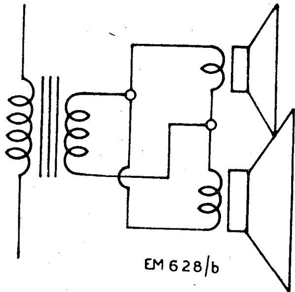
Il mod. « 405 » differisce dal mod. « 115 » per l'adozione di due altoparlanti. Ecco lo schema di inserzione.
