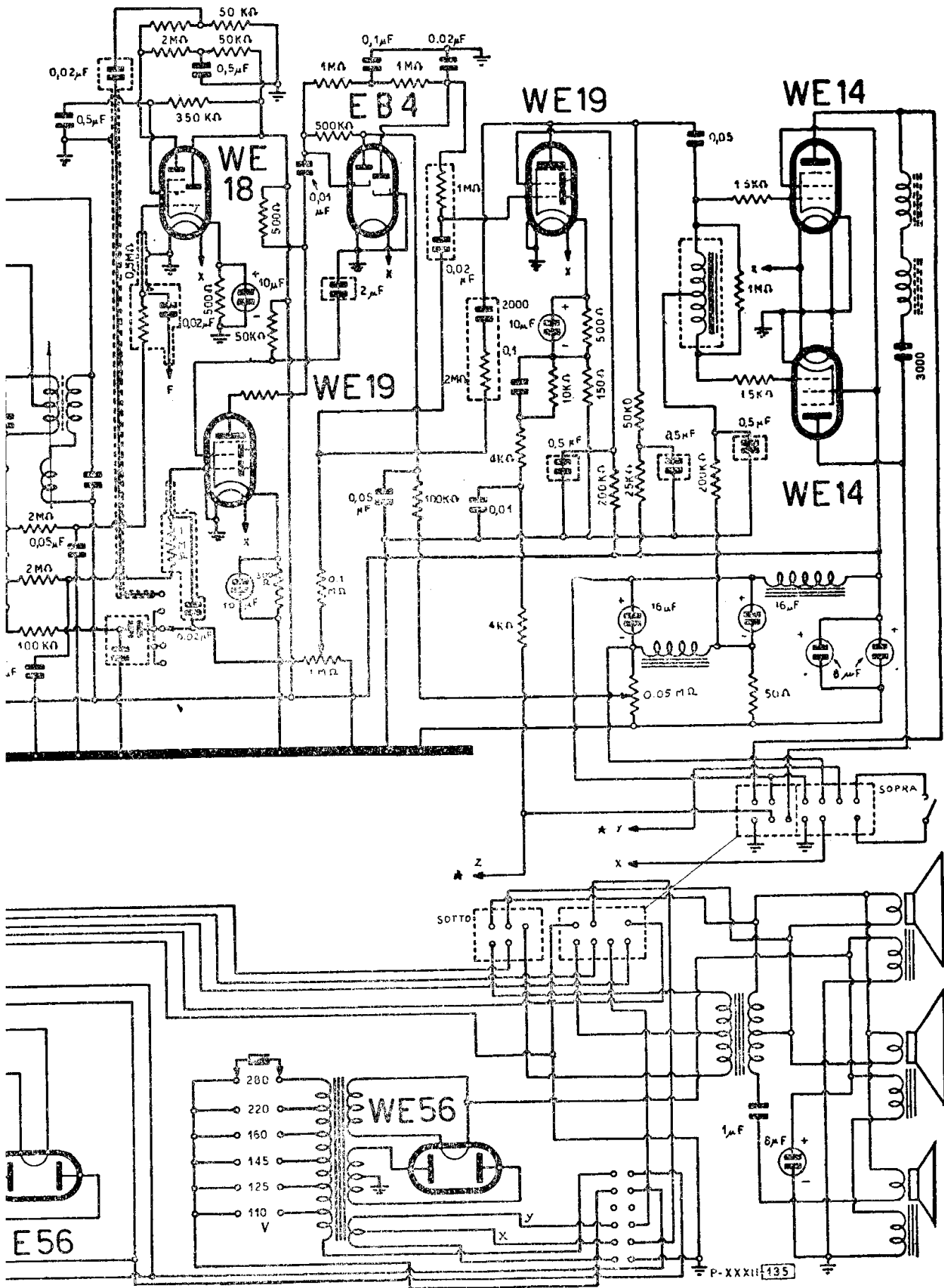
1246 „ RADIOFONOGRARO
