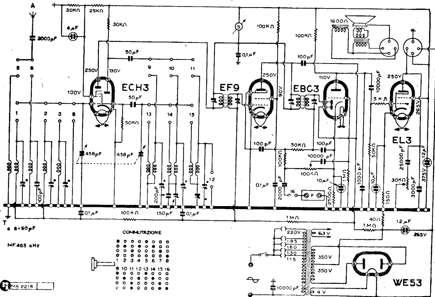
RADIO LAMBDA - MOD. « R 365 M »
