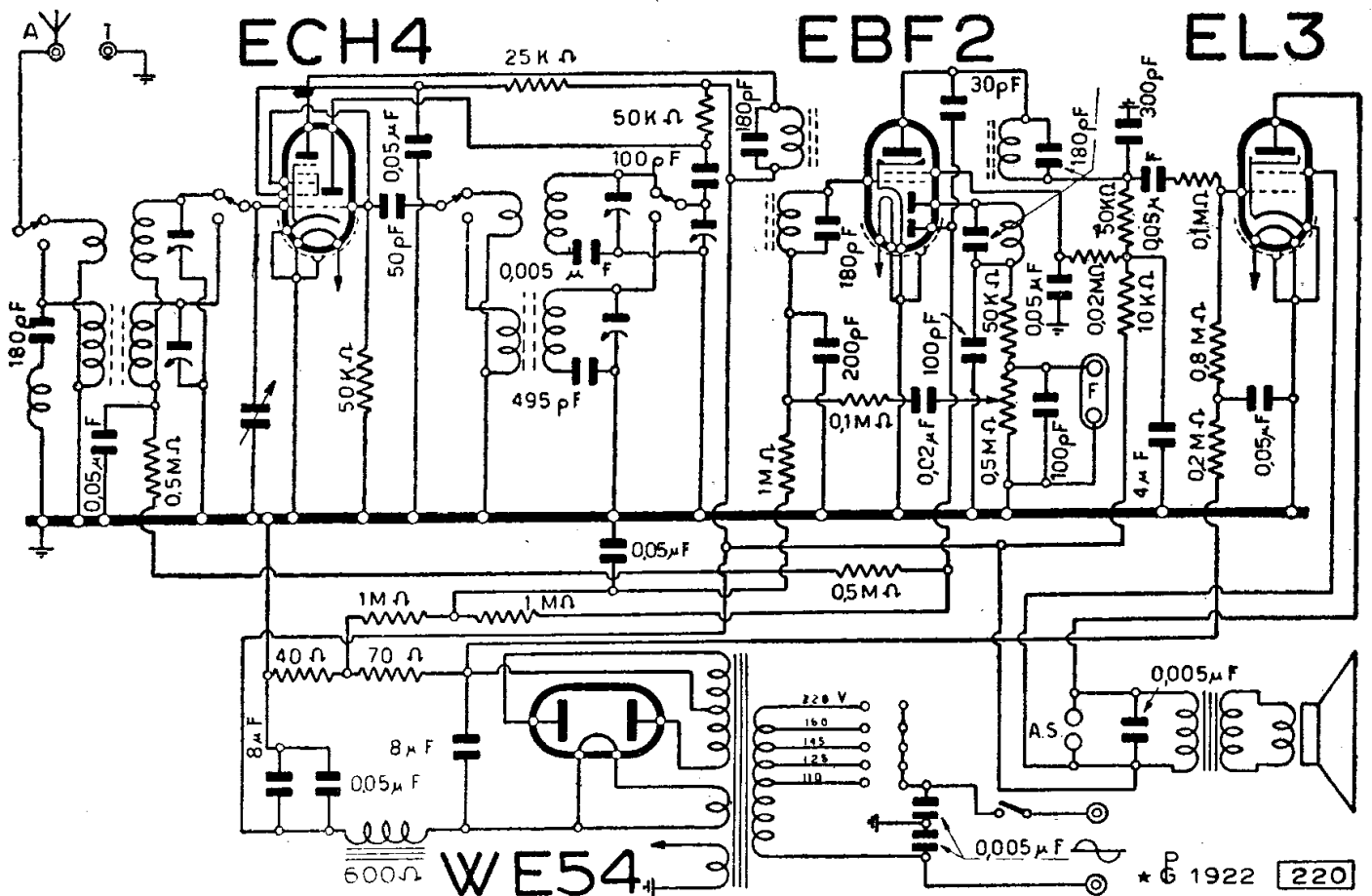
MINERVA - MOD. « 4441 »
