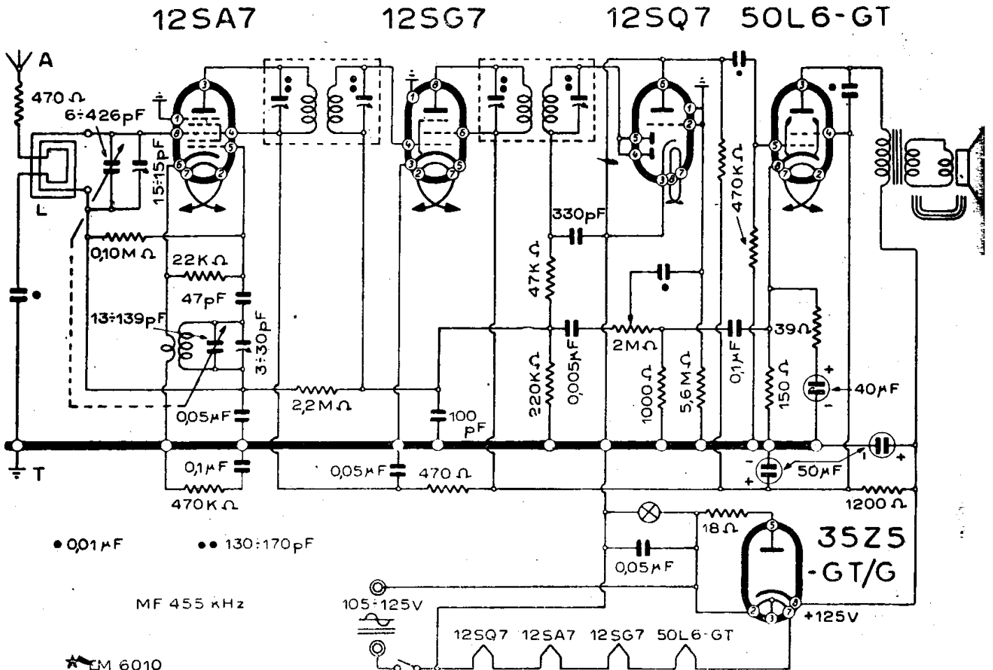
GENERAL ELECTRIC - MODD. « 100 » « 101 » « 103 » « 105 »
