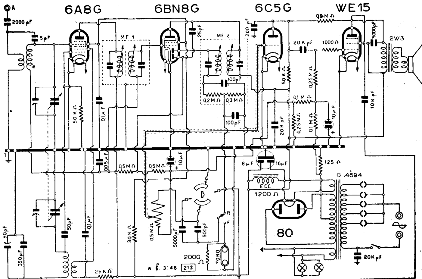
S.I.A.R.E. - MOD. « 438 »
