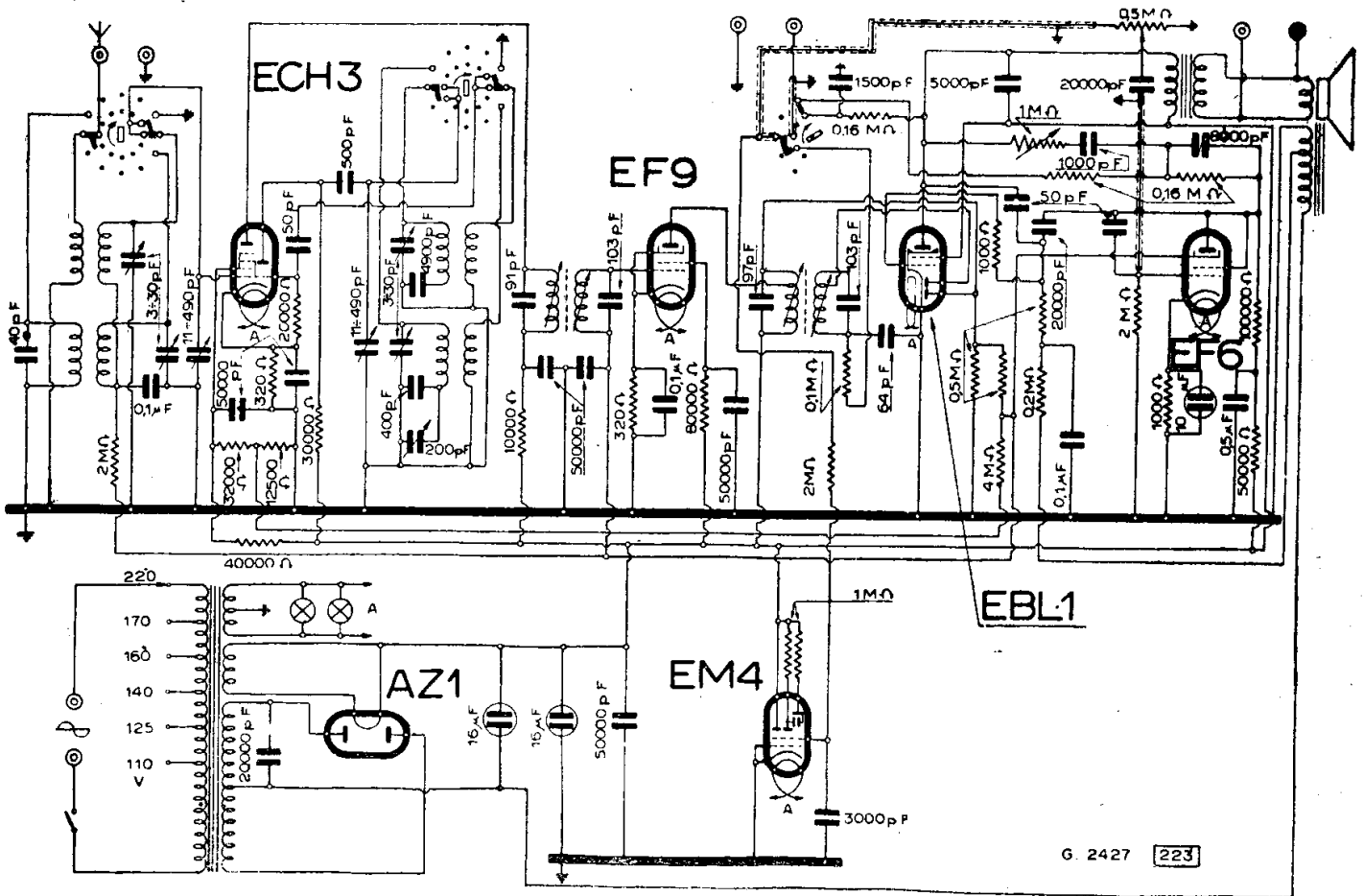
PHILIPS RADIO - MOD. « 466 »
