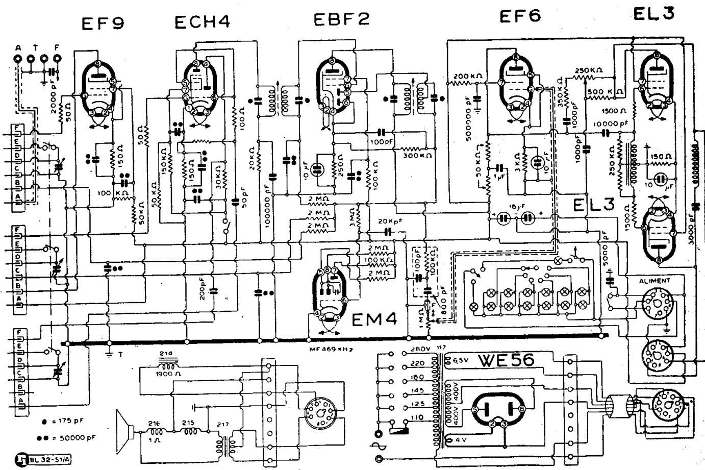
SIEMENS S. A. - MOD. « S 8108 »
