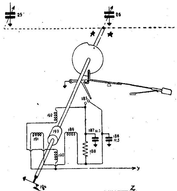
Il dispositivo di comando automatico (a motore, del Siemens mod. « S 1246 » (fig. 4).
