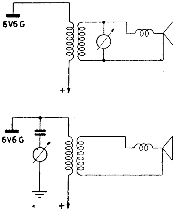
Come si collega un misuratore di uscita durante le operazioni di taratura. Sopra: uno strumento a bassa impedenza; sotto a impedenza elevata.
