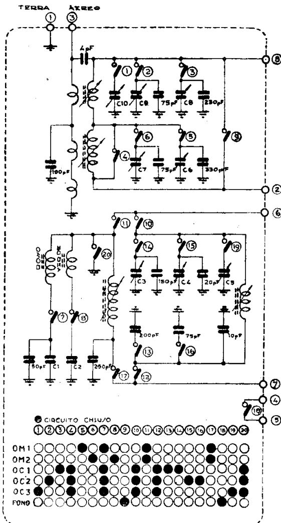
Lo schema elettrico del gruppo P1 Nova.
