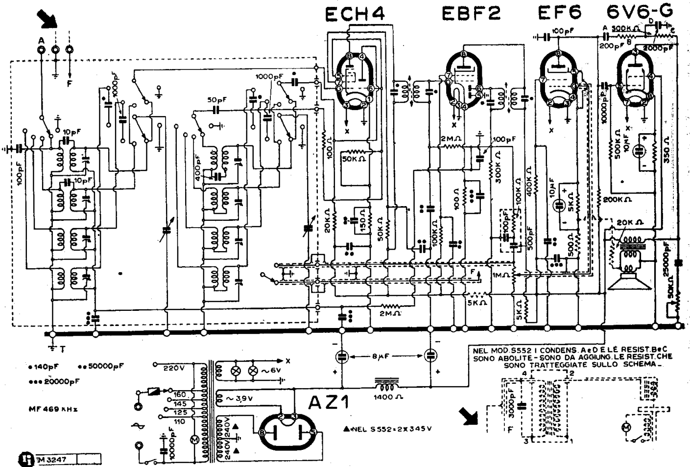
SIEMENS S. A. - MODD. « S 547 » « S 552 FONO »
