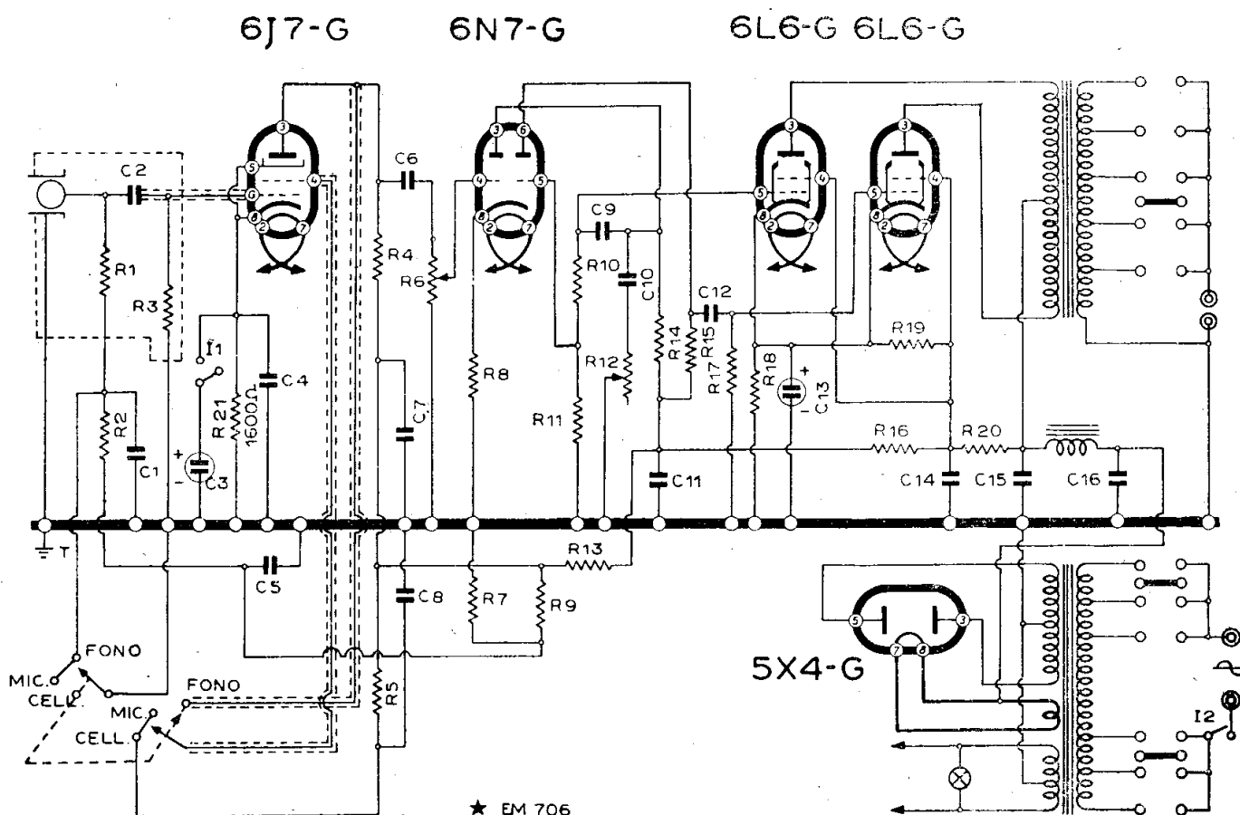
DUCATI - AMPLIF. MOD. « RG 2501/1 »
