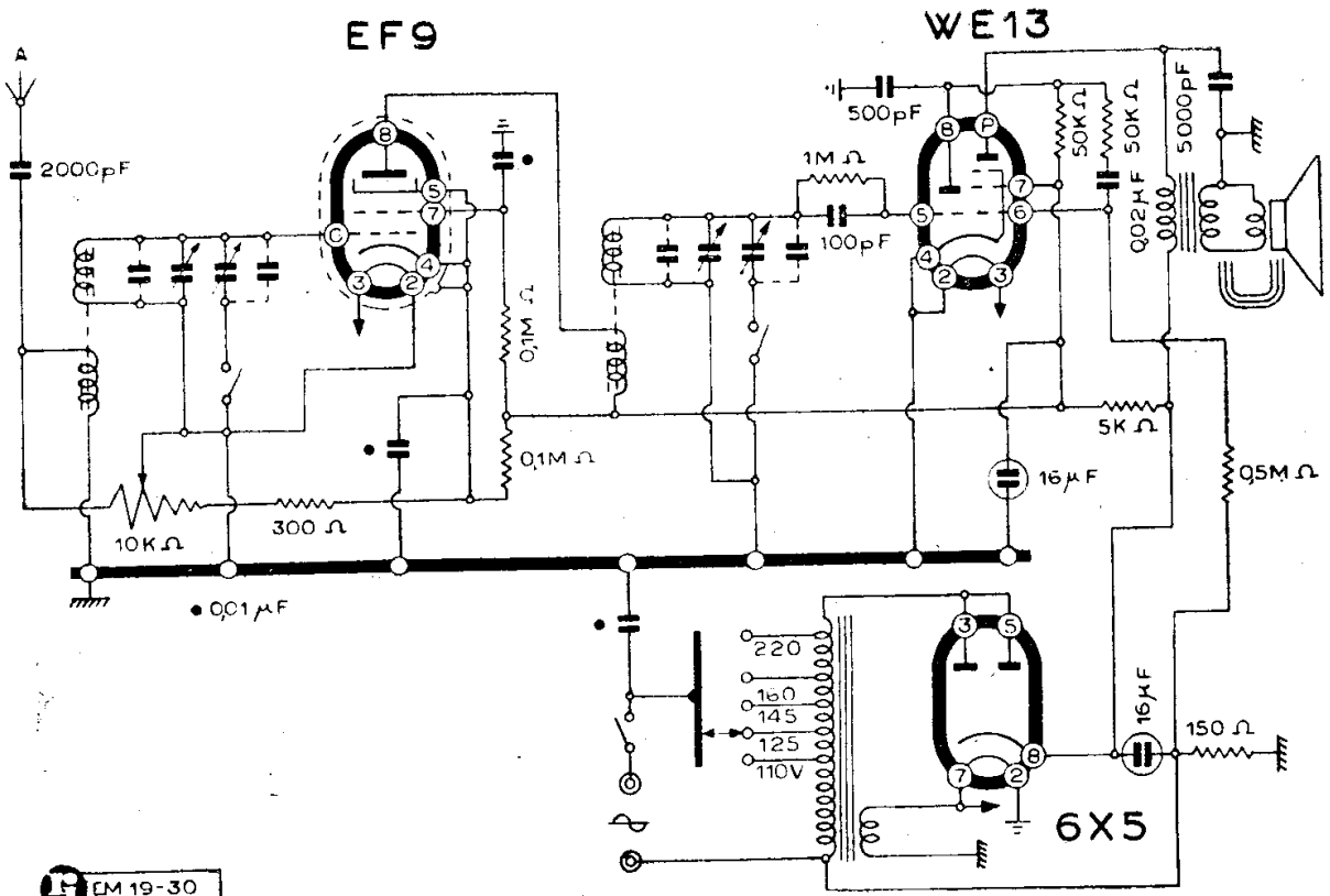
MINERVA - MOD. « 473/1 »
