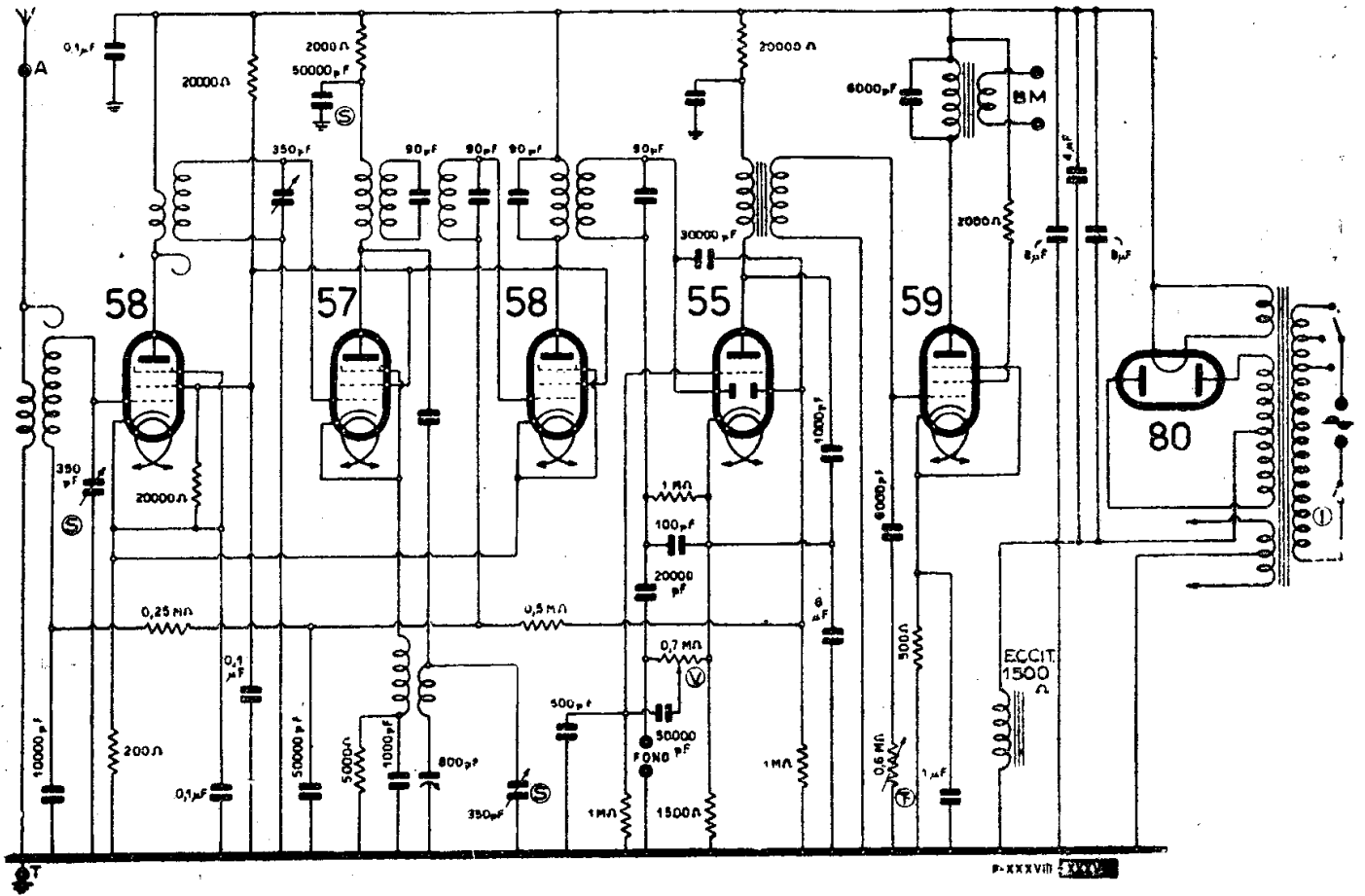
WATT RADIO - MOD. « 900 »
