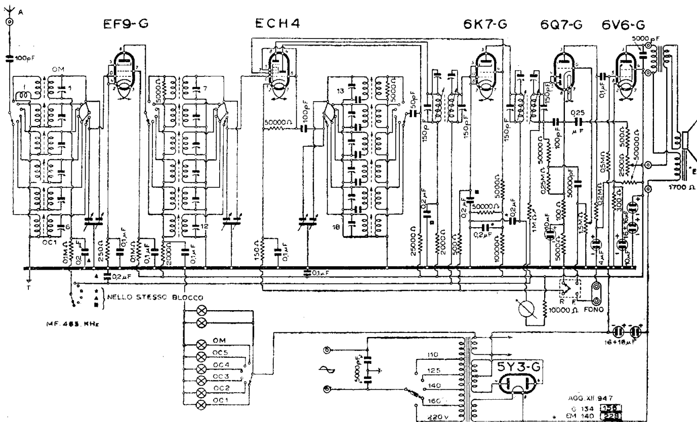
ALLOCCIO, BACCHINI & C. - MOD. « 615 »
