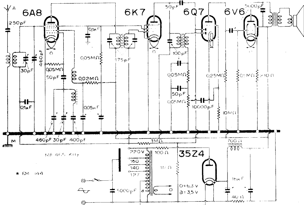
ALLOCCIO, BACCHINI & C. - MOD. « 514 »
