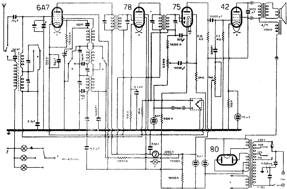
ALLOCCIO, BACCHINI & C. - MOD. « 51 F. »
