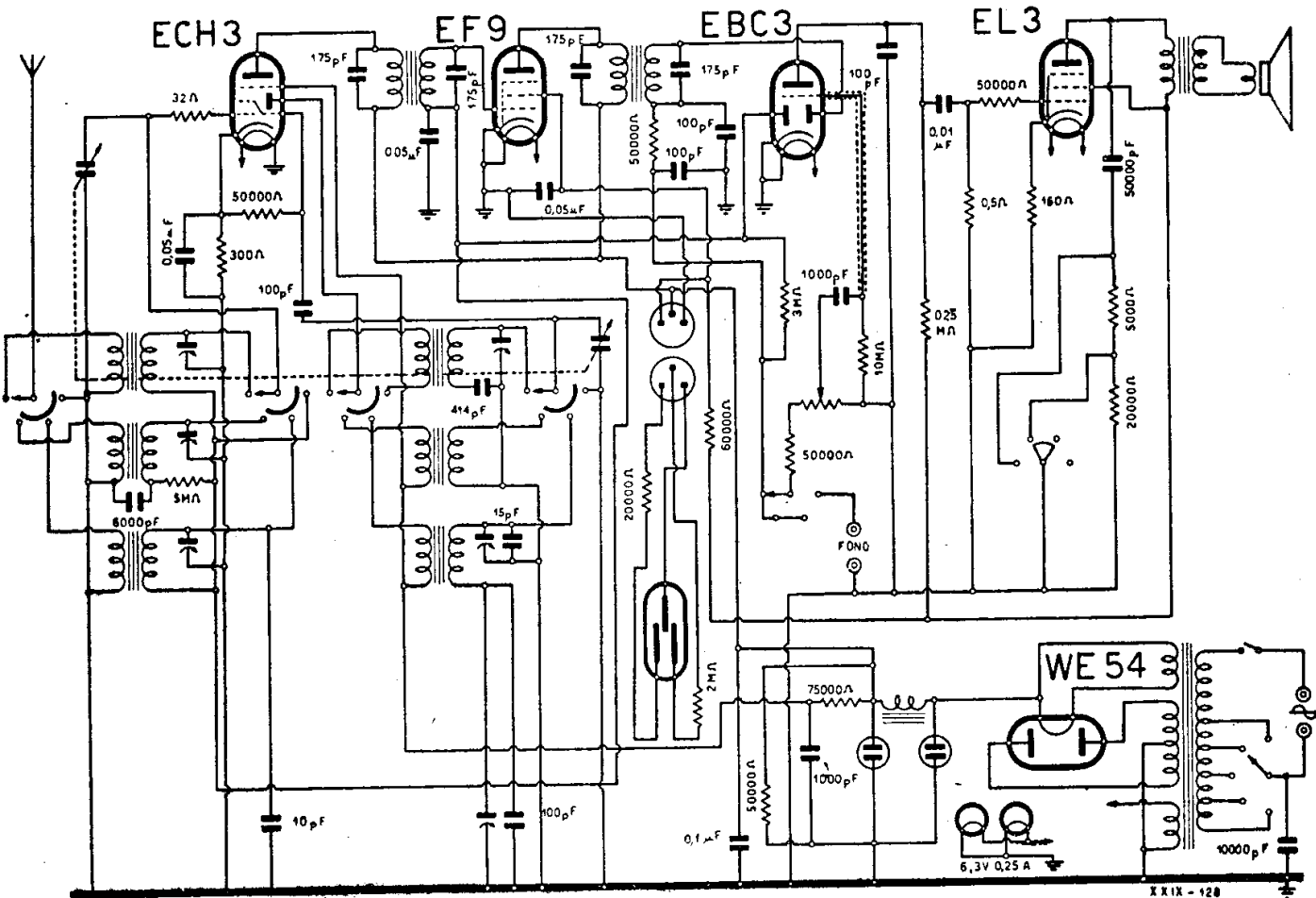
S.A.F.A.R. - MOD. « 535 »
