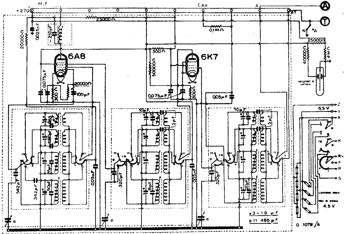
F.I.M.I. - MOD. PHONOLA « 880 » - PARTE AF
