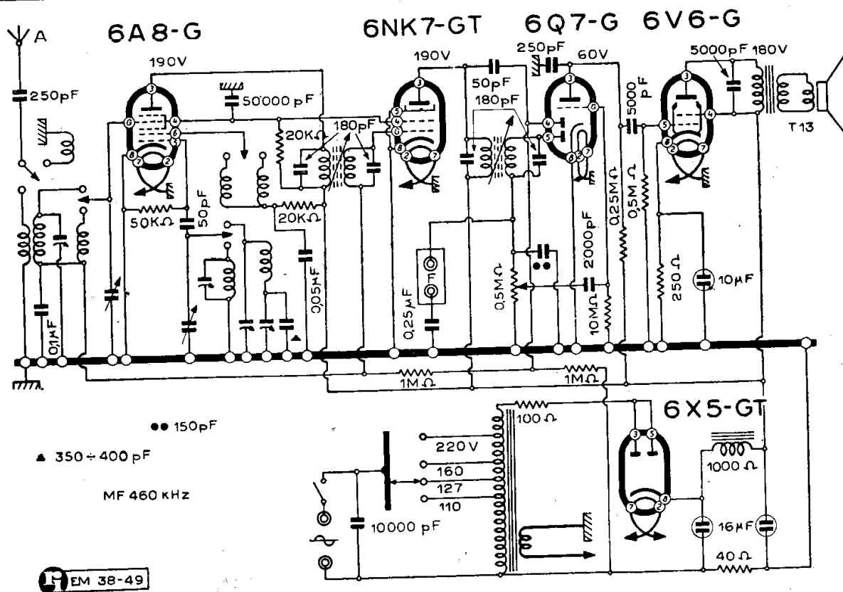
WATT RADIO - MOD. « 48 »
