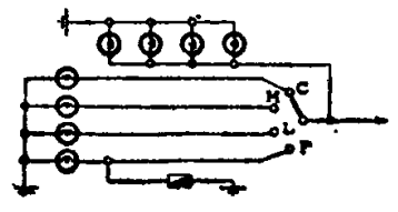
S.I.A.R.E. - MOD. « 496 C » - CROSLY - MOD. « 289 C » (I PARTE)
