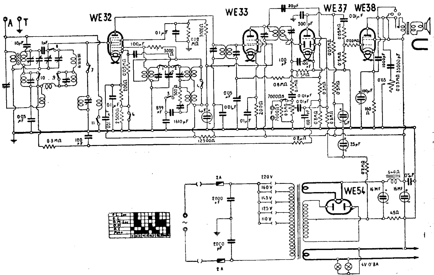
MINERVA - MOD. « 375 . 1 PH »
