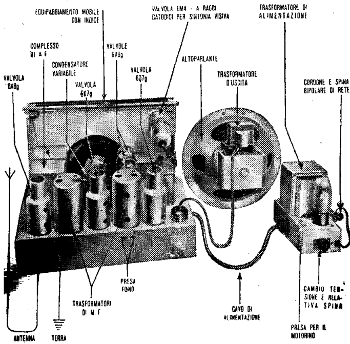
Il telaio del mod. « 716 » visto posteriormente.
