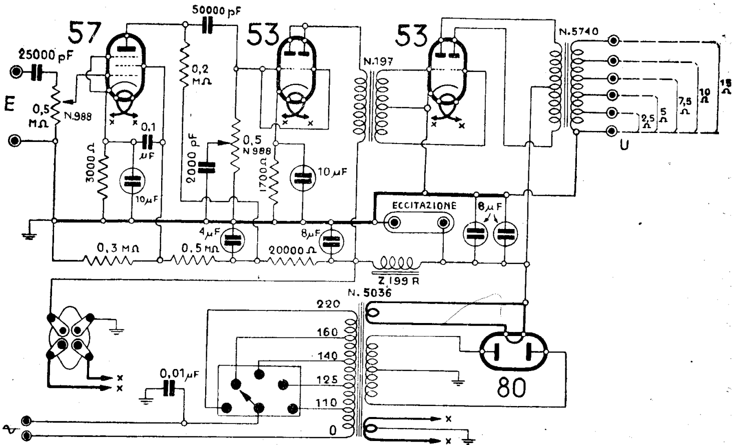
GELOSO (SGC) - AMPLIFICATORE MOD. « G 17 A »
