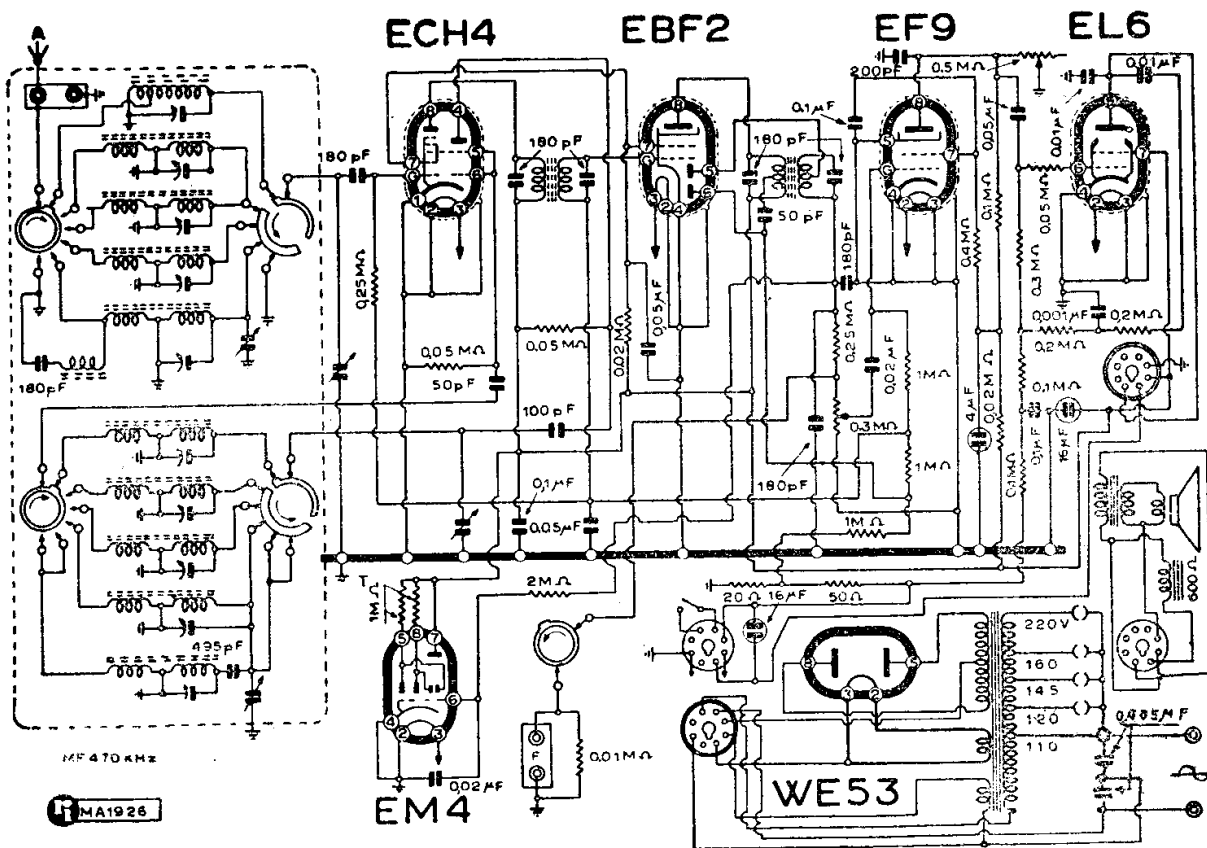
MINERVA - MOD. « 465/1 »
