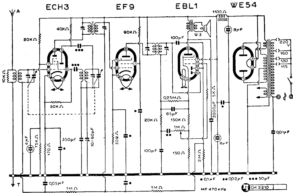
RADIO LAMBDA - MOD. « GL 141-M »
