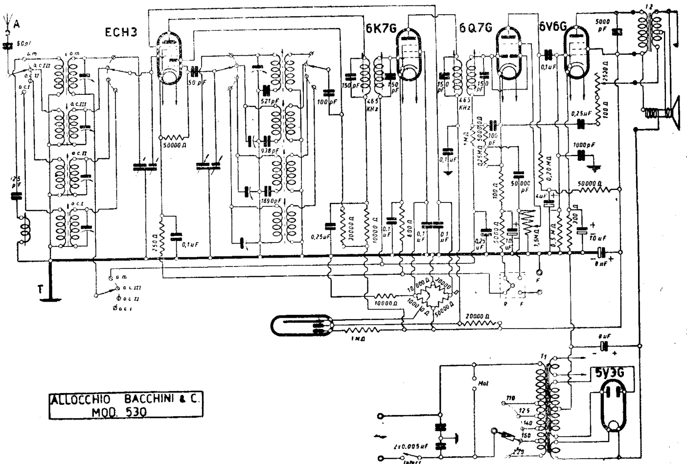
ALLOCCIO, BACCHINI & C. - MOD. « 530 »
