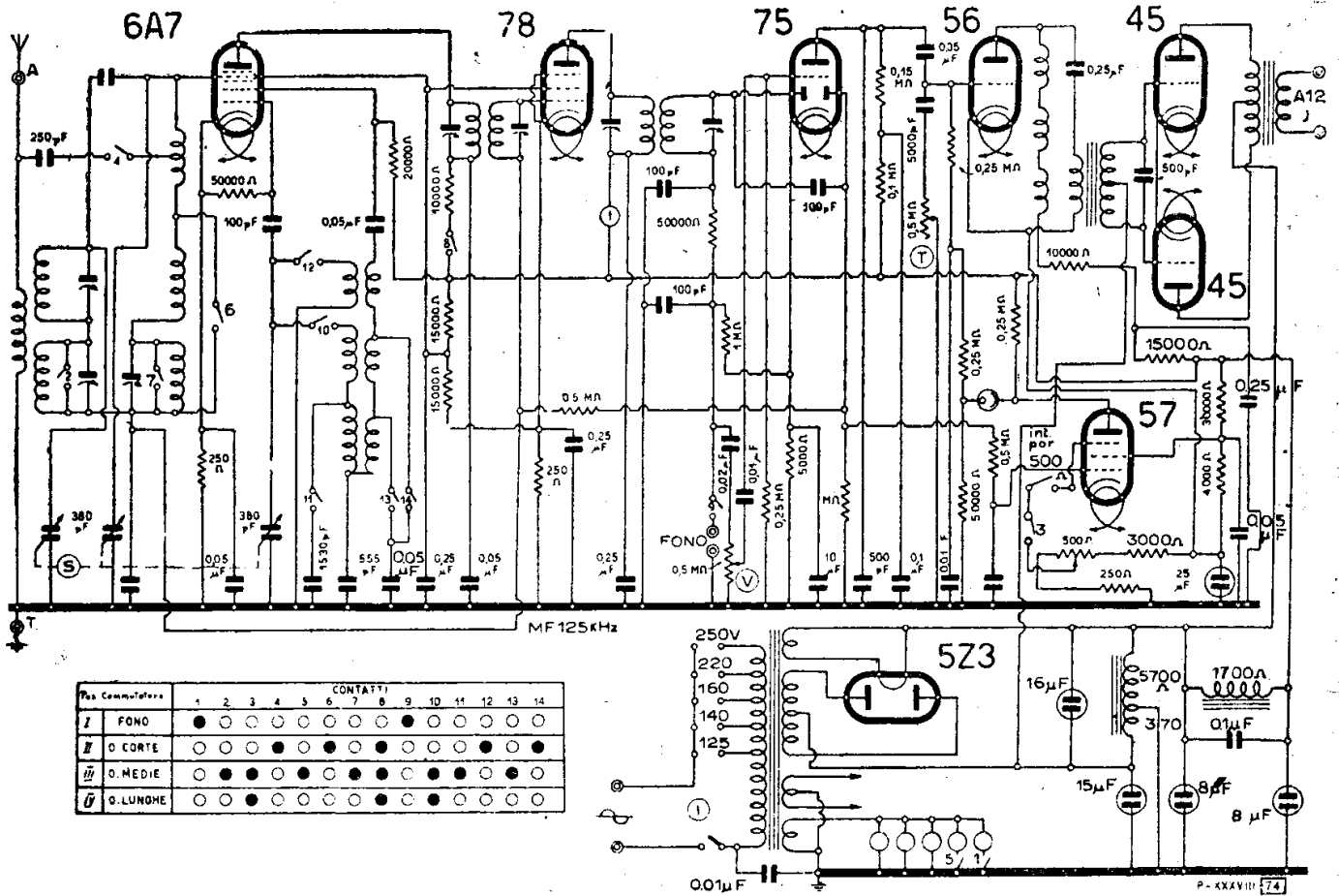
WATT RADIO - MOD. « SUPER IMPERIALE »
