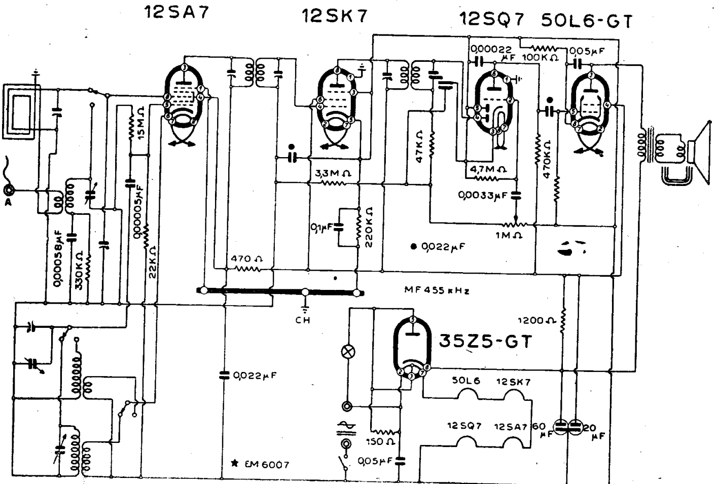
CROSLY - MOD. « 56 TX »
