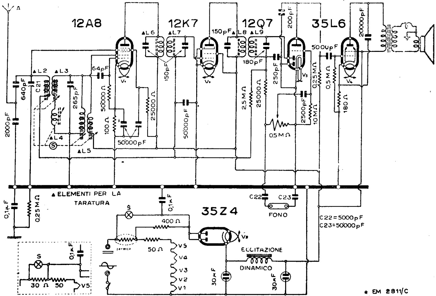
RADIOMARELLI - MOD. « FIDO II »
