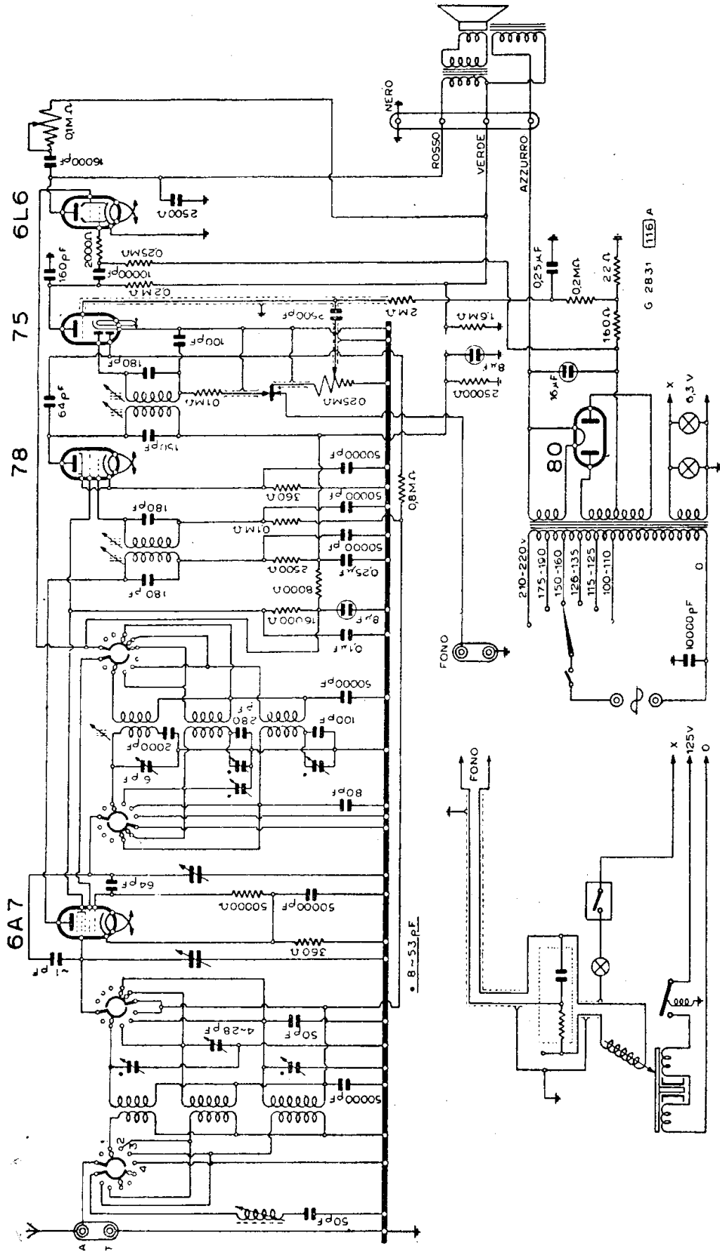
RADIOMARELLI - MOD. « AXUM II »
