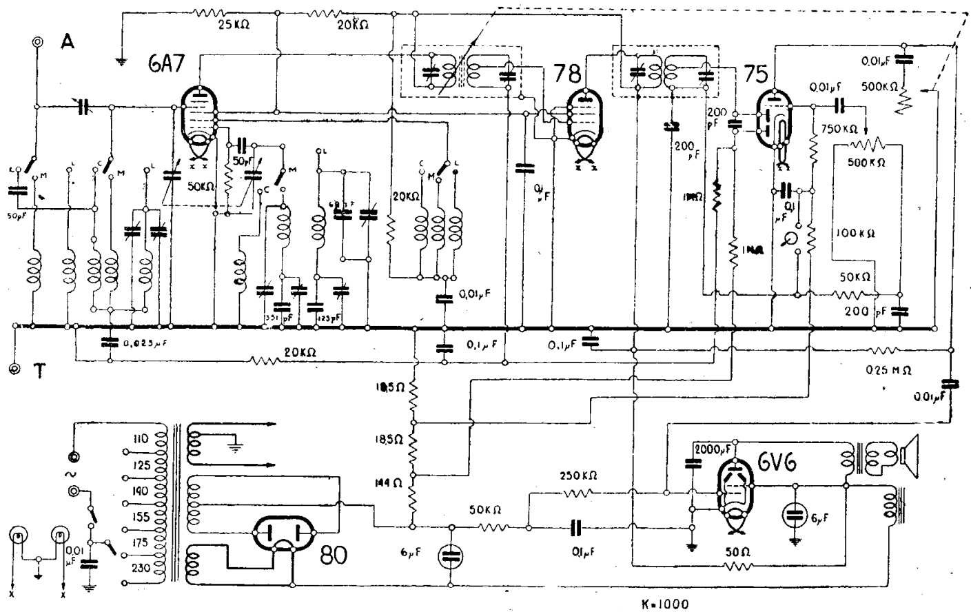
MAGNADYNE - MOD. « SV 12 » - « SV 14 » (REALIZZA I MOD. « SV 112 » - « SV 114 »)
