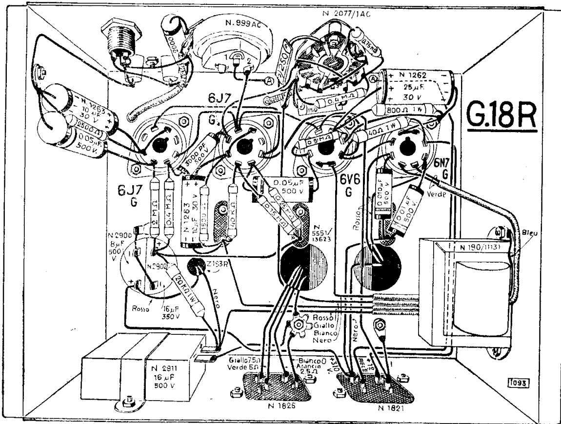
Il piano costruttivo dell'ampificatore « G18 R »
