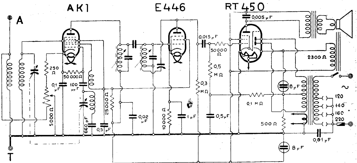
F.I.M.I. - MOD. PHONOLA « 670 M »
