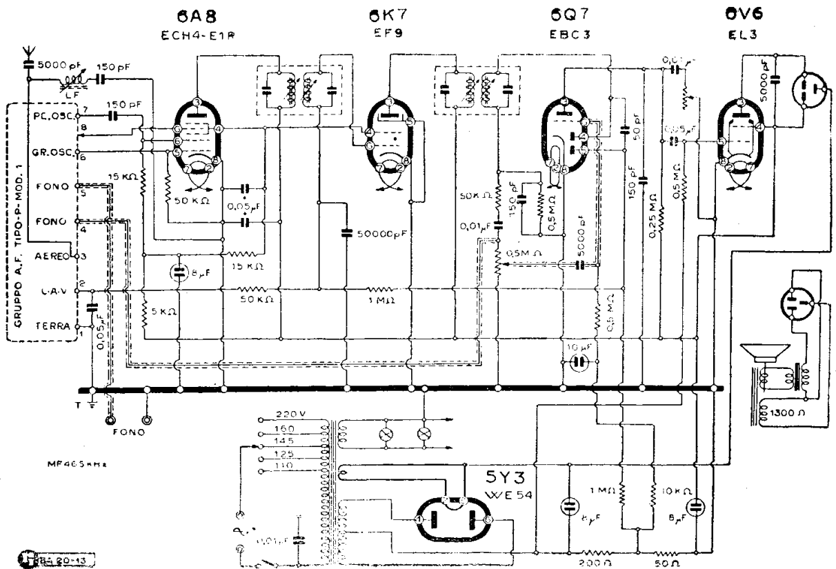
NOVA - MOD. « 503-A 1 »
