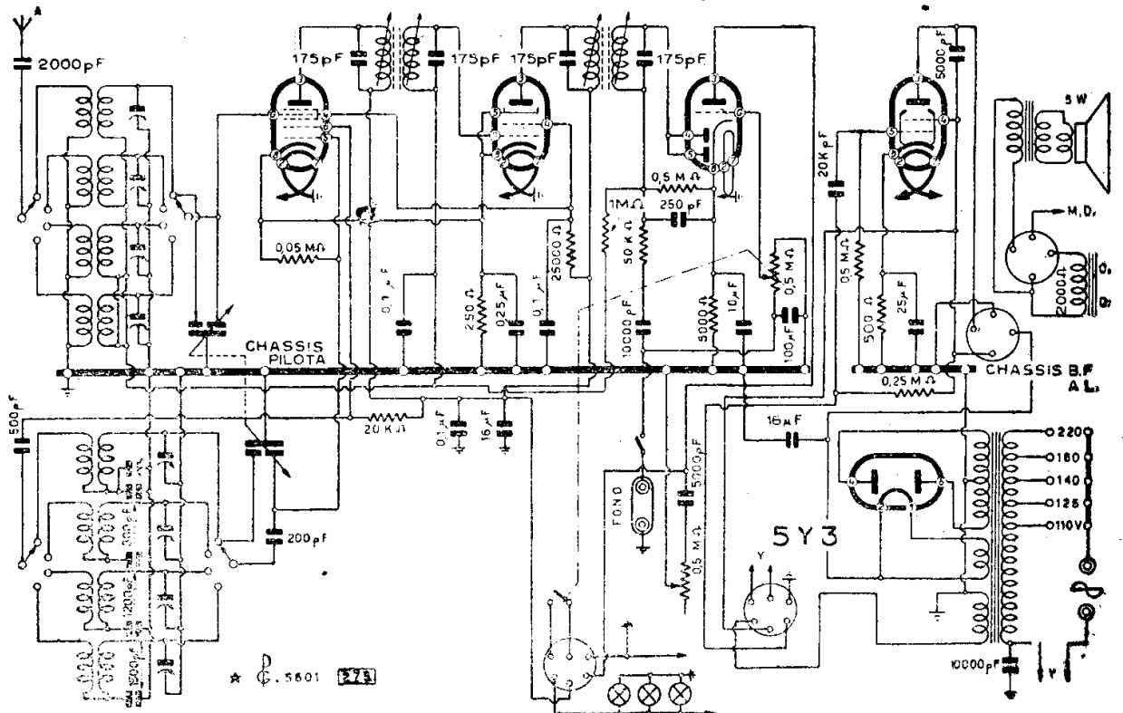
OREM - MOD. « 542 »
