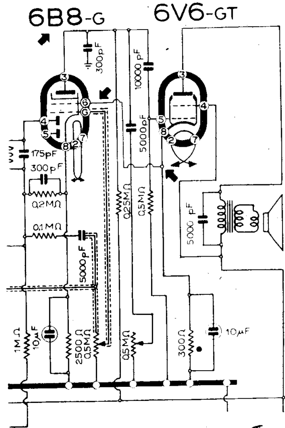
Una variante del circuito dei modd. «1256» - «2256» per l'impiego della 6B8-G in luogo della 6Q7-G.
