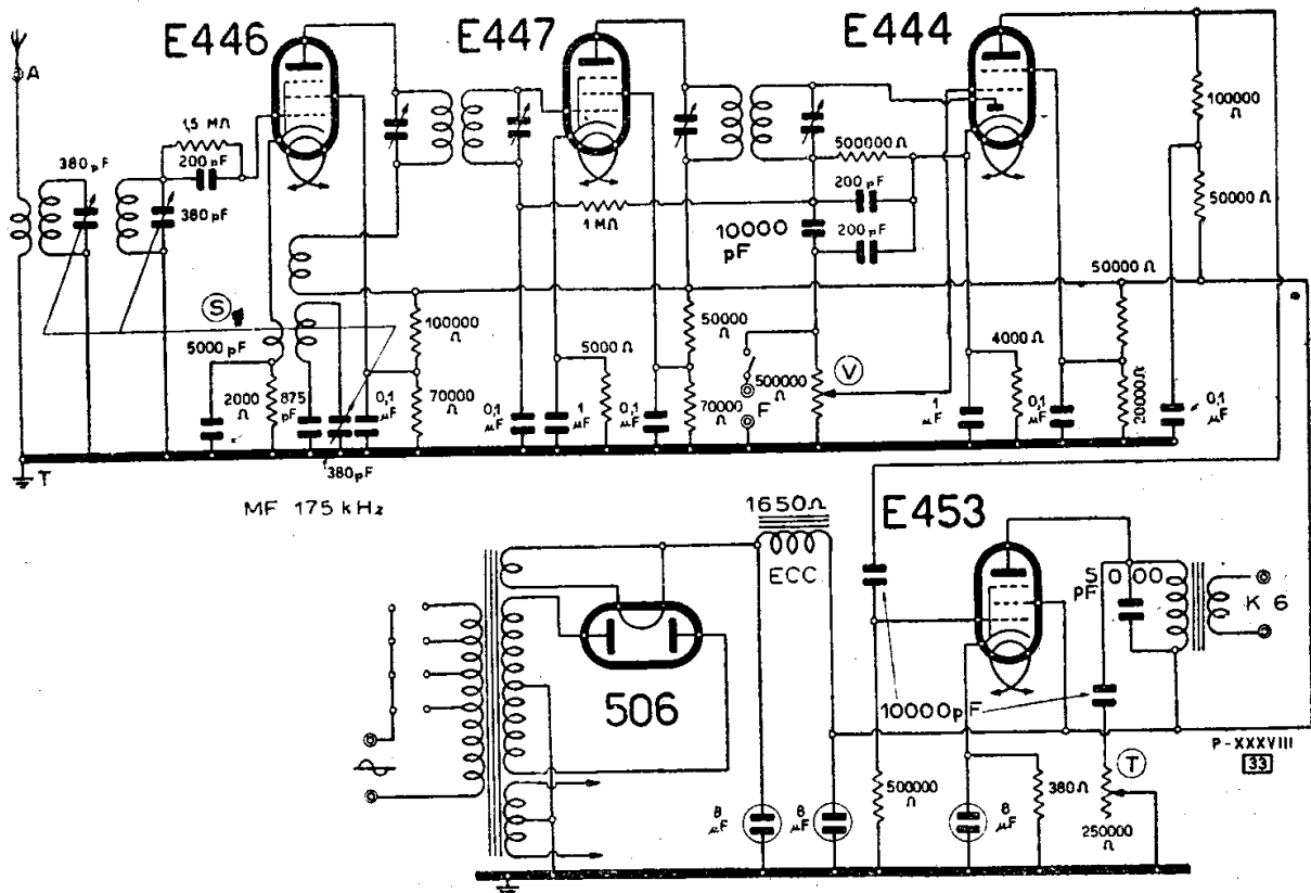
WATT RADIO - MOD. « APOLLO »
