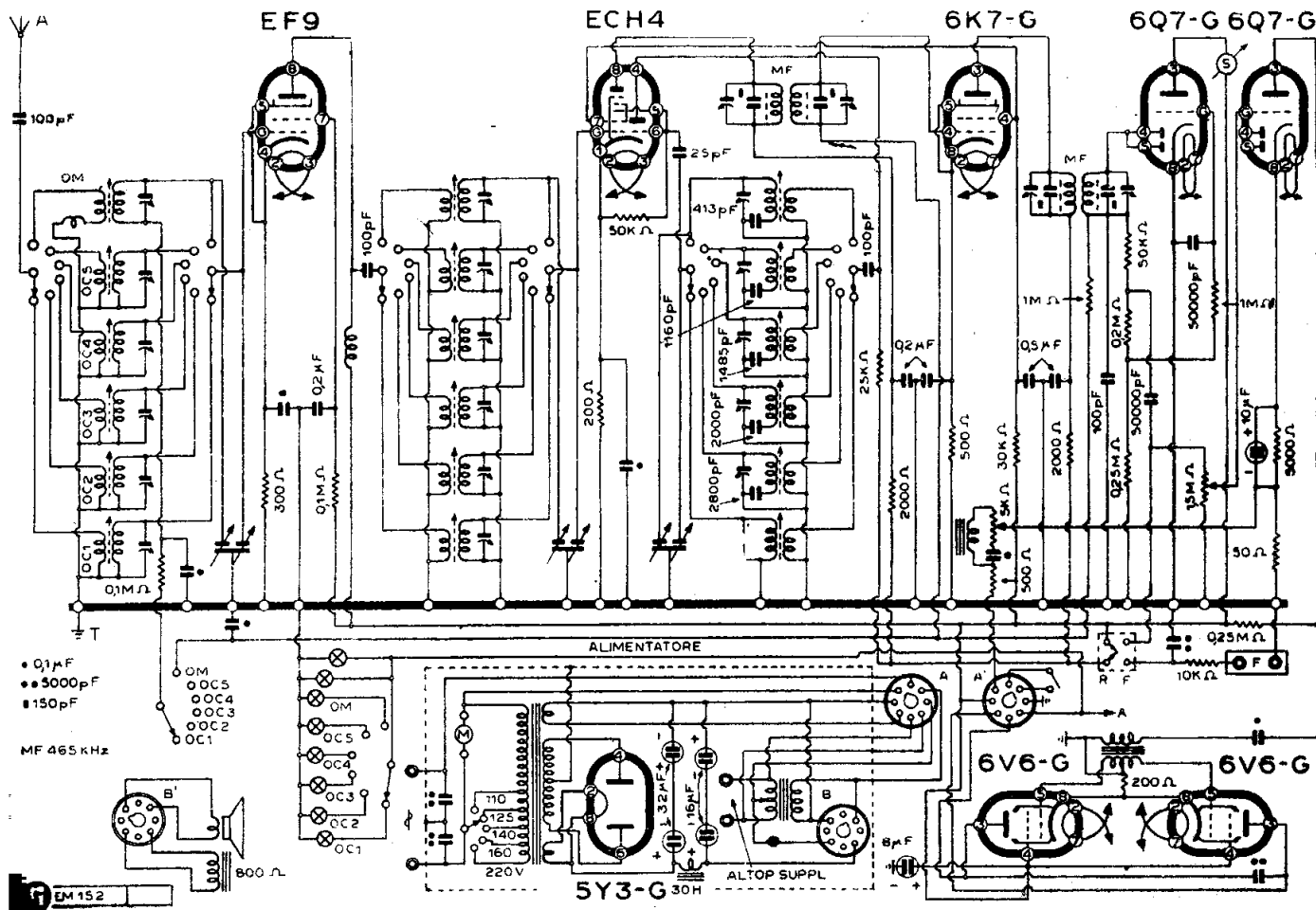
ALOCCHIO, BACCHINI & C. - MOD. ( 816 )
