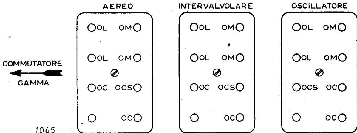
La disposizione dei compensatori nel Phonola « 622 » - « 715 » - « 716 » - « 717 » - « 718 » - « 1010 ».
