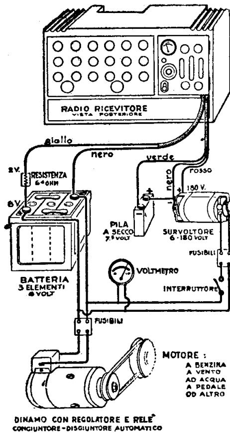
L'impianto di manutenzione del radiorecettore coloniale « Dubat » con batteria e survolto.
