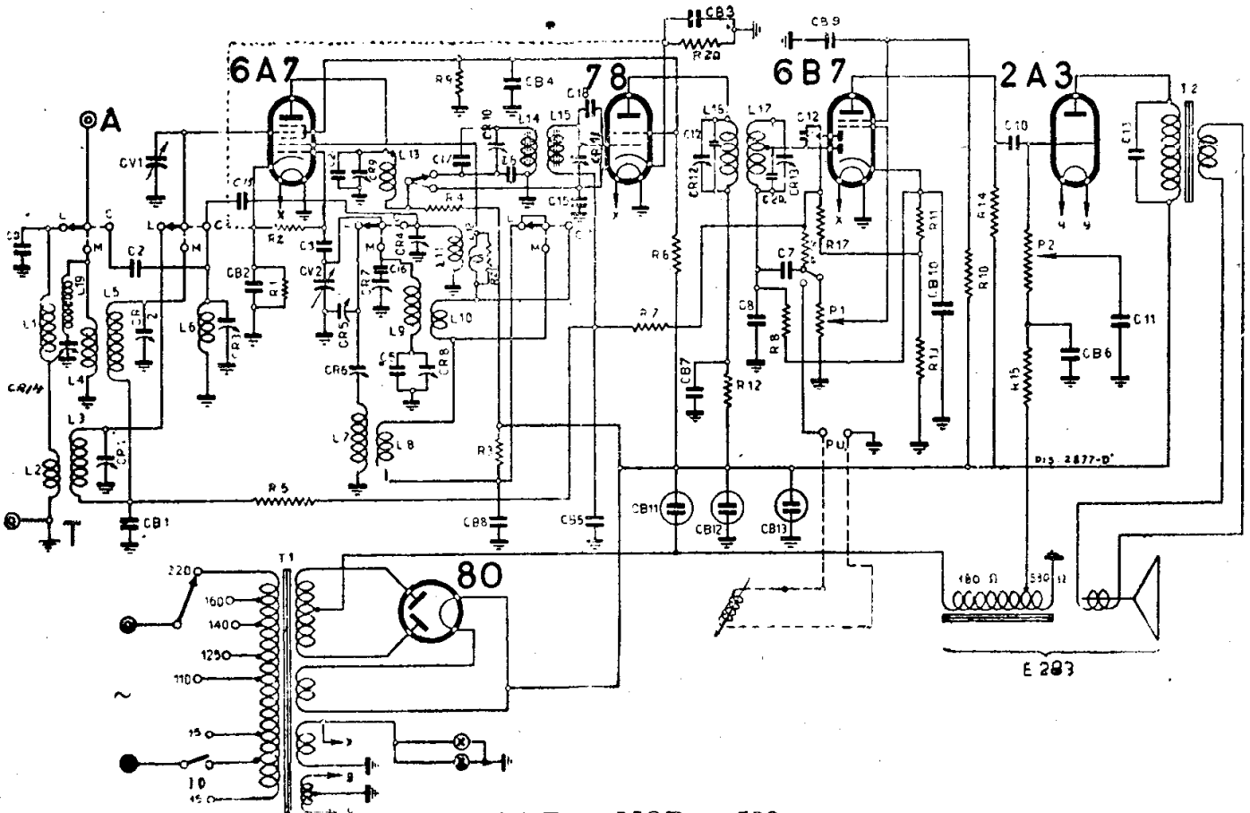
S.A.F.A.R. - MOD. « 533 »
