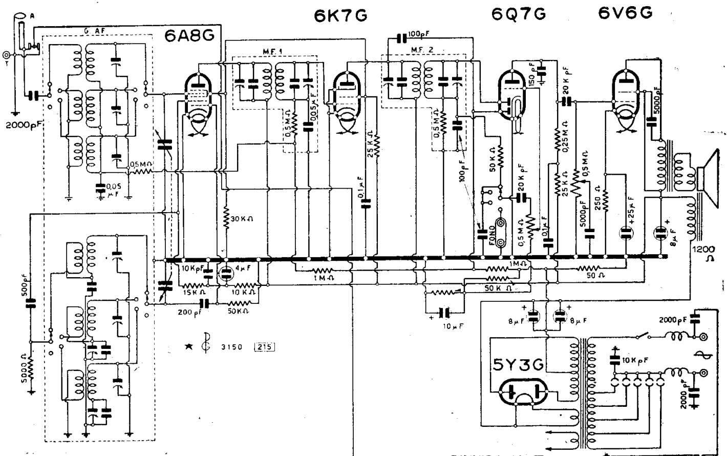
S.I.A.R.E. - MOD. « 445 »
