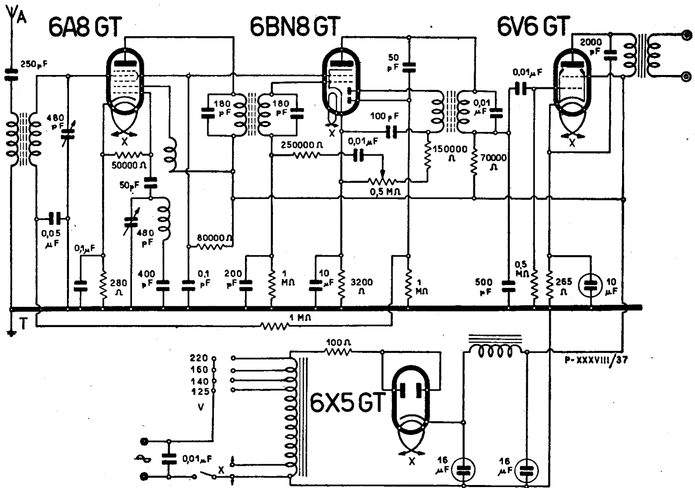
WATT RADIO . MOD. « CUCCIOLO »
