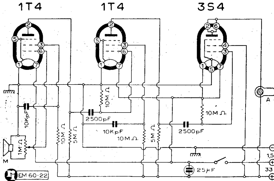
ZENITH - AMPLIFICATORE PER SORDITA' MOD. « HP9/AS1 »
