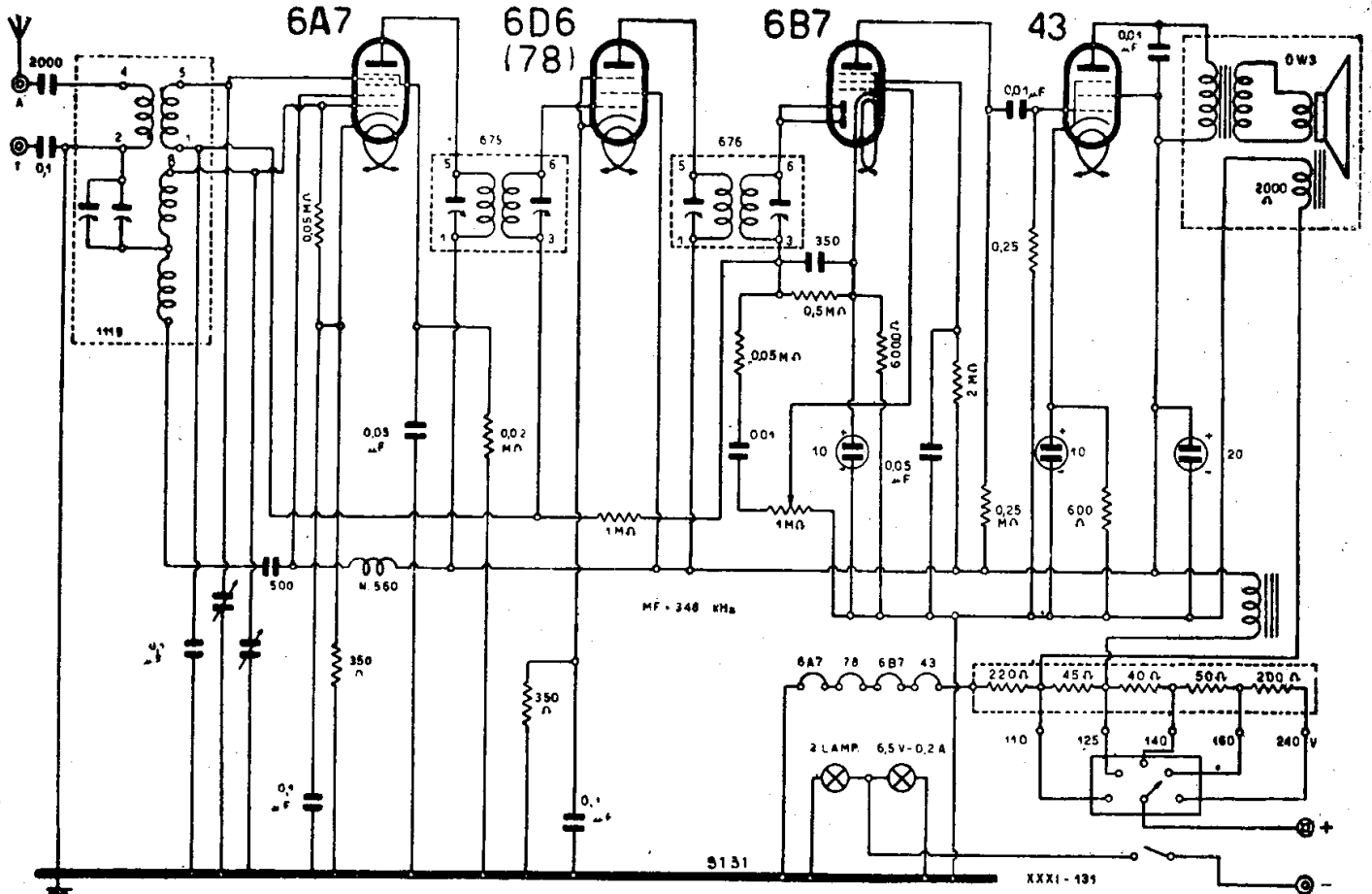
S.I.A.R.E. CROSLY - MOD. « 7411 D.C. »
