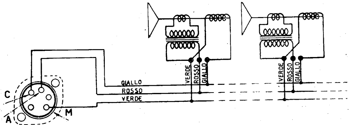
Negli amplificatori Magneti Marelli il collegamento di uno o più altoparlanti in uscita è semplice. Tenere presente che A = sorgente a corrente microfonica per la bobina mobile; C = massimo positivo per la corrente di eccitazione. I due circuiti confluiscono a una massa in comune = M.
