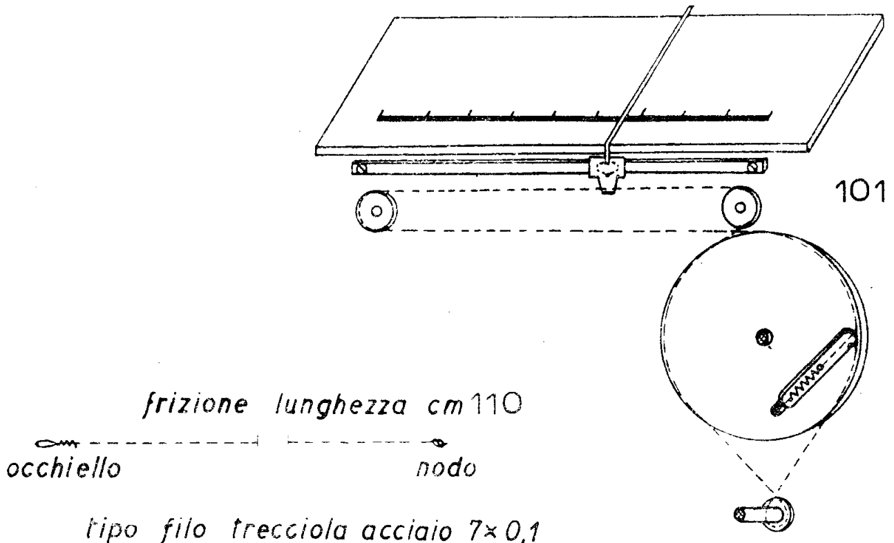
Qui sotto: schema della disposizione della funcella di comando dell'indice.
