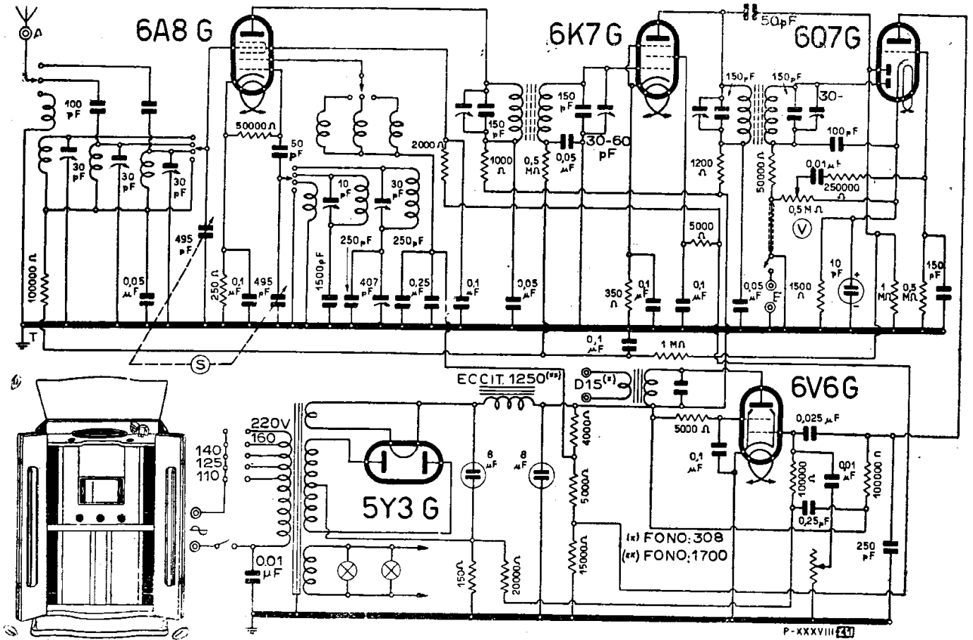
WATT RADIO - MOD. « FRECCIA »
