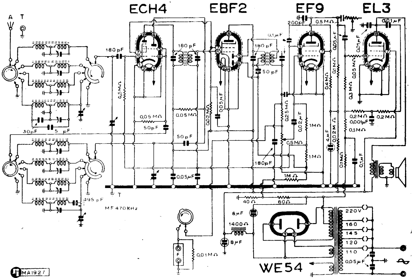
MINERVA - MOD. « 465/2 » « 475/2 »
