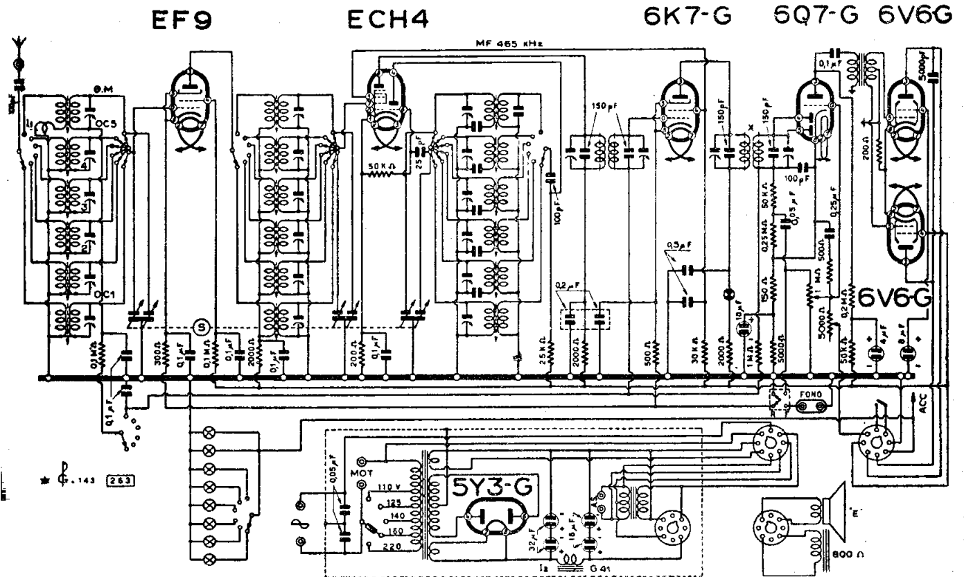
ALLOCCIO, BACCHINI & C. - MOD. « 715 »
