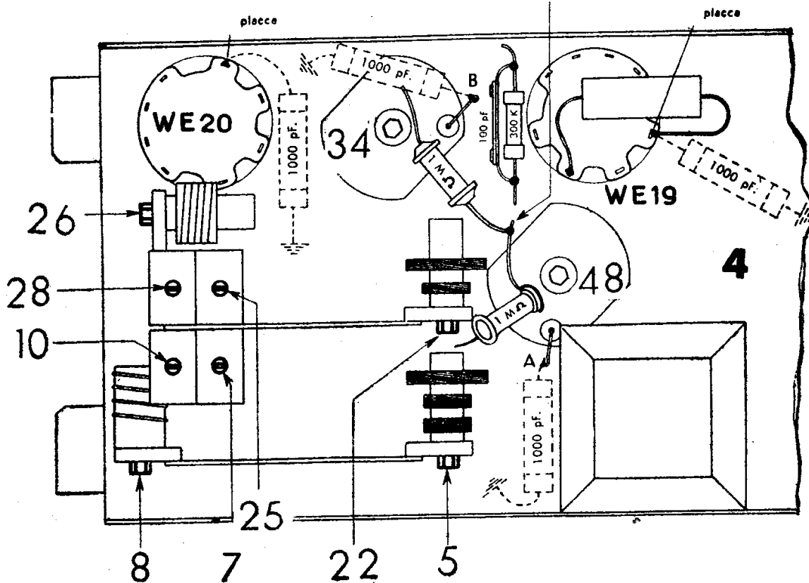
Il piano costruttivo del Siemens mod. « S 422 » con la posizione dei compensatori di taratura (4). In alto: particolare del circuito durante l'allineamento (3).
