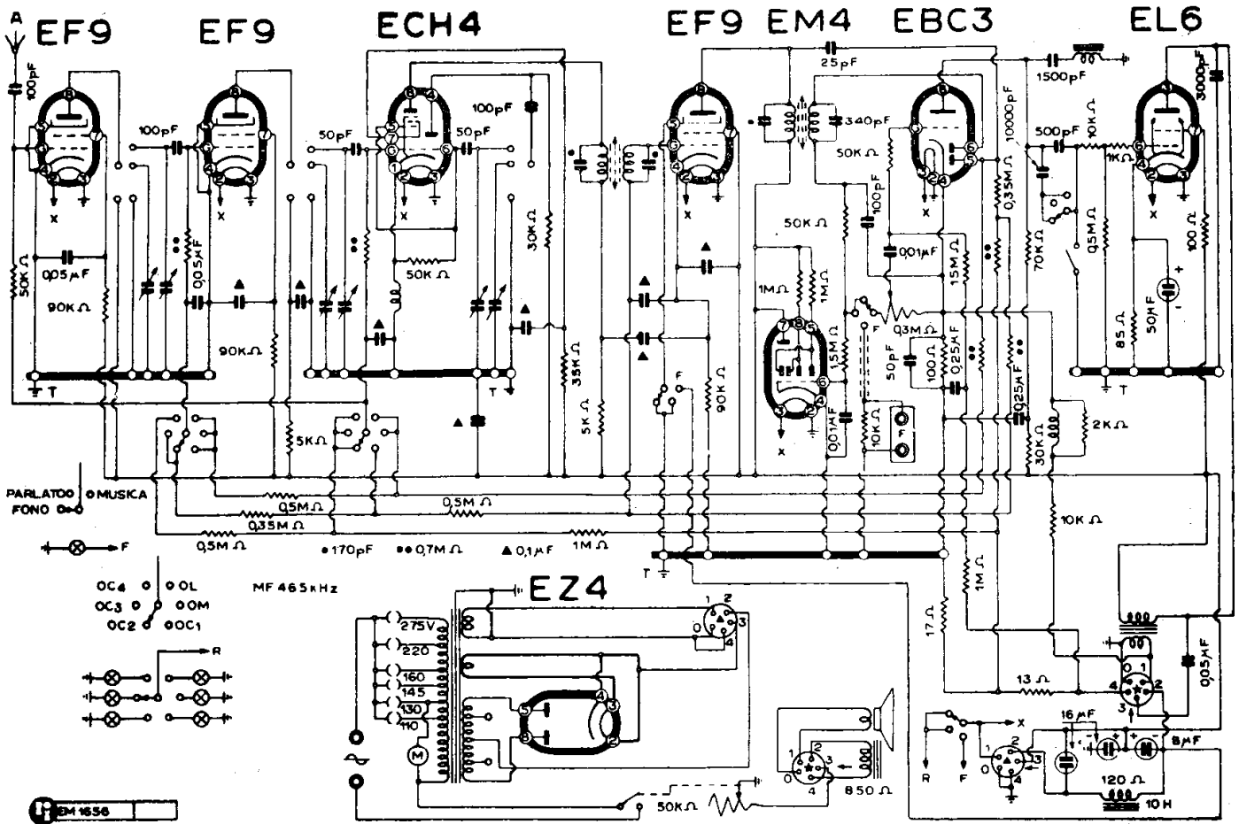
LA VOCE DEL PADRONE - COLUMBIA - MARCONIPHONE MODD. « MARCONI 1706 » « 1707 » « 1716 »
