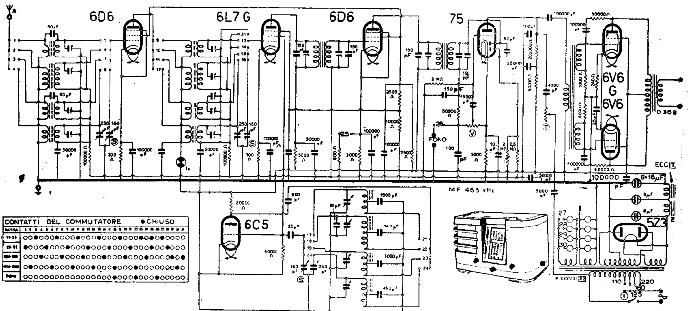
WATT RADIO - MOD. « FREJUS »
