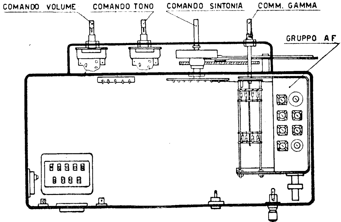
Schizzo del telaio « 530 » con l'ubicazione dei comandi e del gruppo AF.
