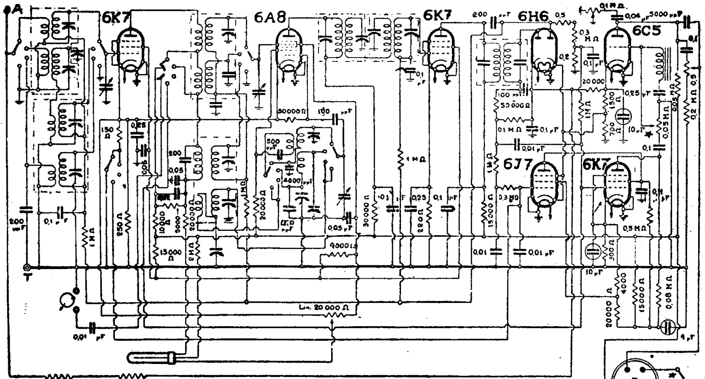
S.I.A.R.E. - MOD. « 472 C »
