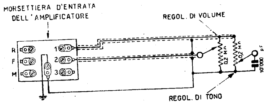
L'inserzione di un regolatore di volume e di un correttore di tono, entrambi manuali in ingresso negli amplificatori Magneti Marelli.
