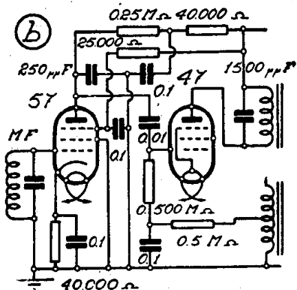
Varianti per i modelli Watt in (a) il « 659 », in (b) e (c) il mod. « Ardito ».
