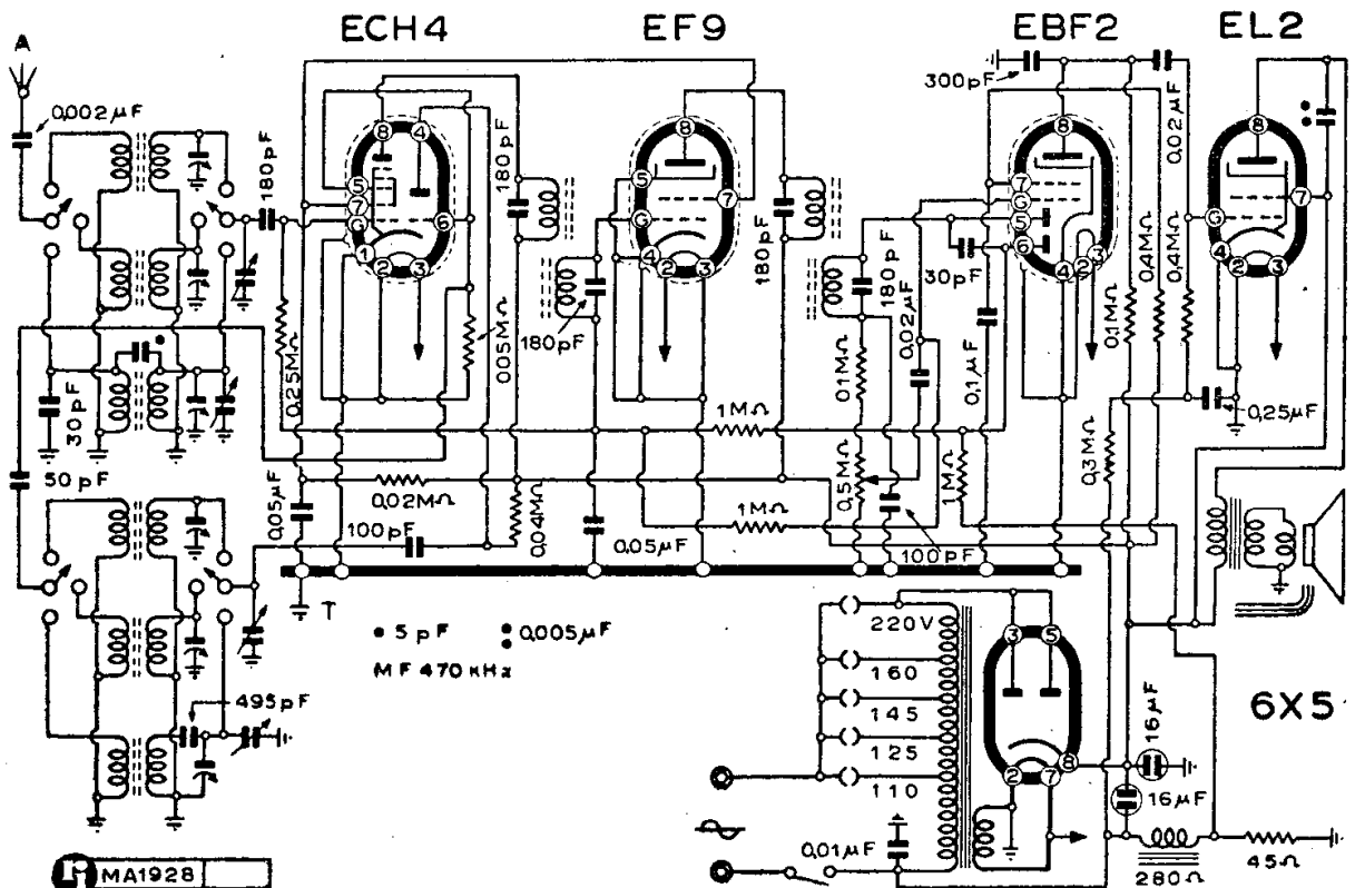
MINERVA - MOD. « 465/3 »
