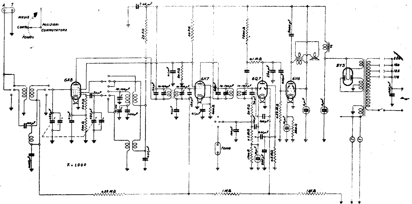
WATT RADIO - MOD. « ALFIERE »
