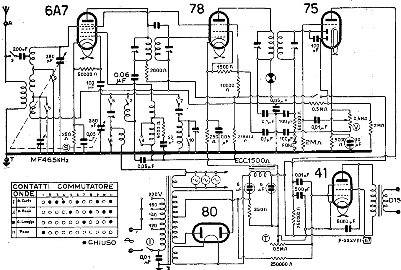
WATT RADIO . MOD. « SIDERODINA »
