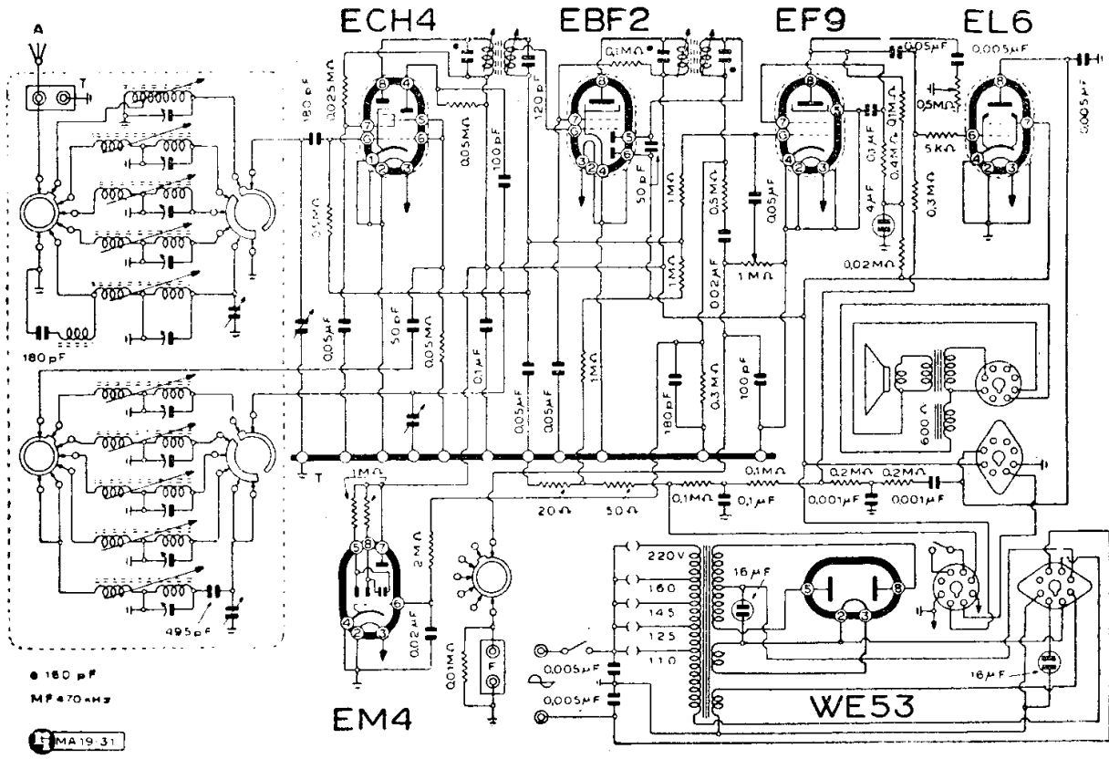
MINERVA - MOD. « 475/1 » « FLORIDA »
