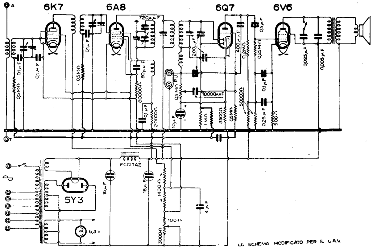
LO SCHEMA MODIFICATO PER IL 6.3V
