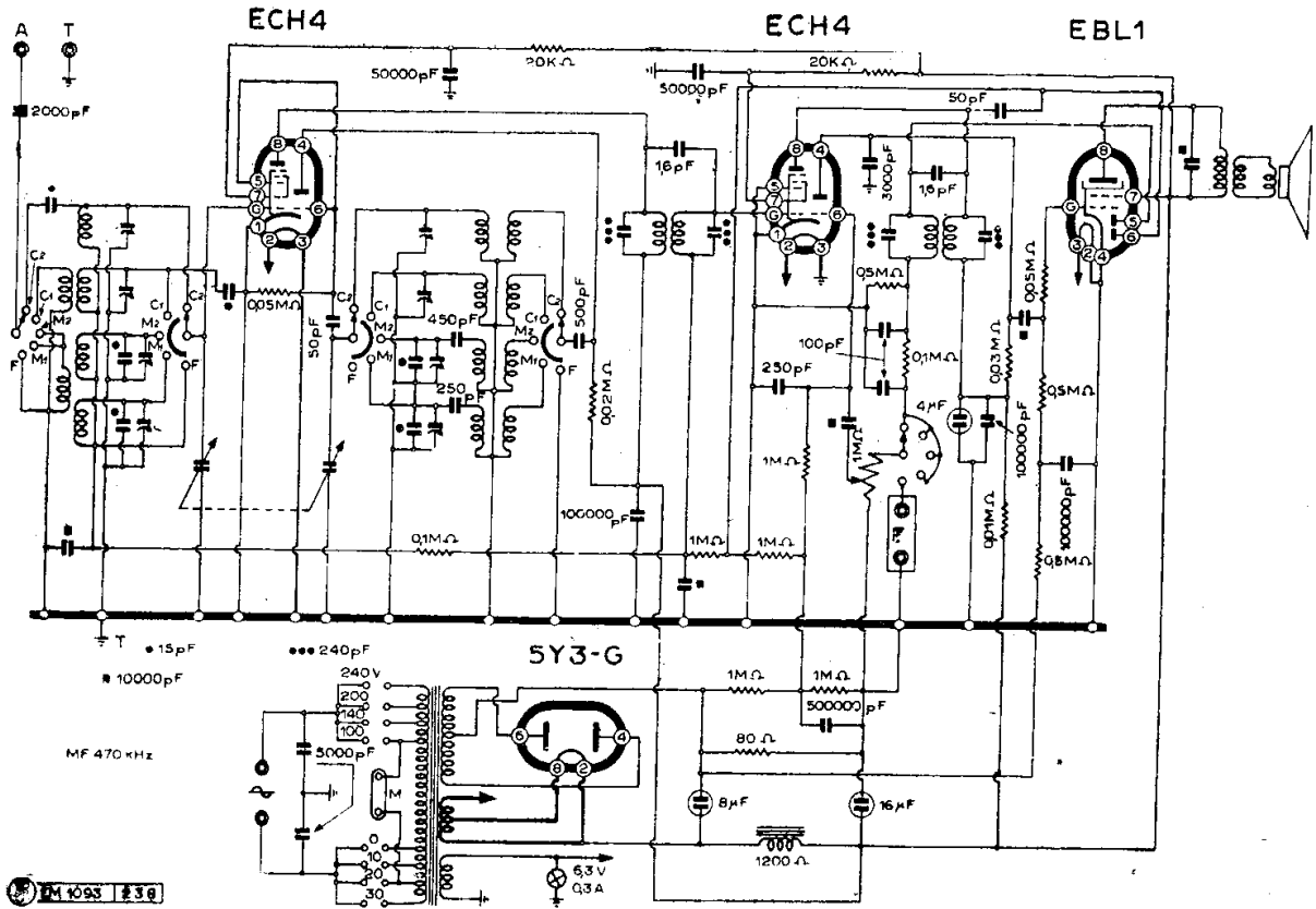
F.I.M.I. - MOD. PHONOLA « 417 »
