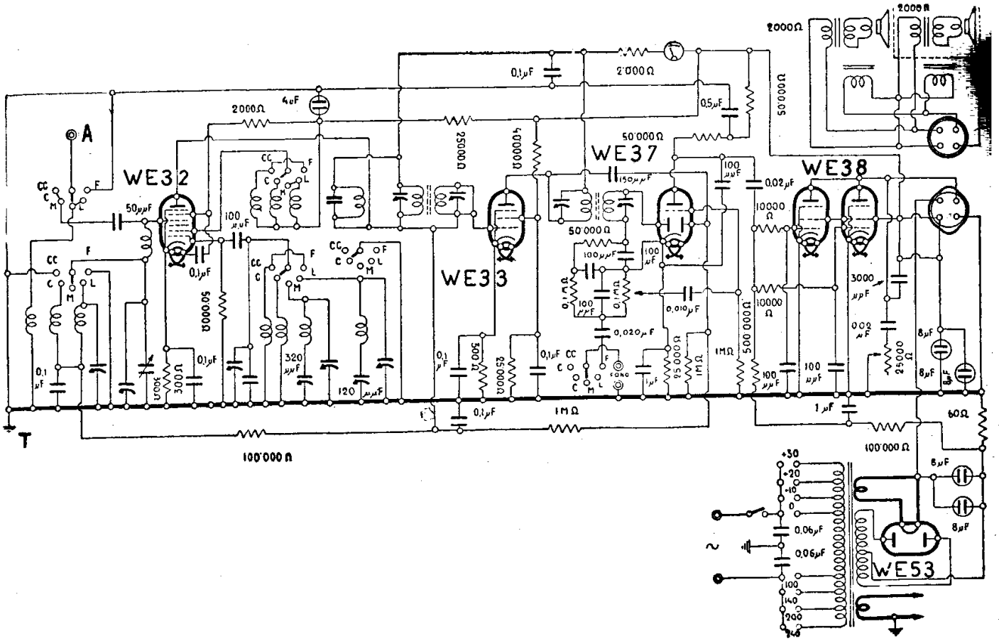
RADIO LAMBDA - MOD. « E 846 »
