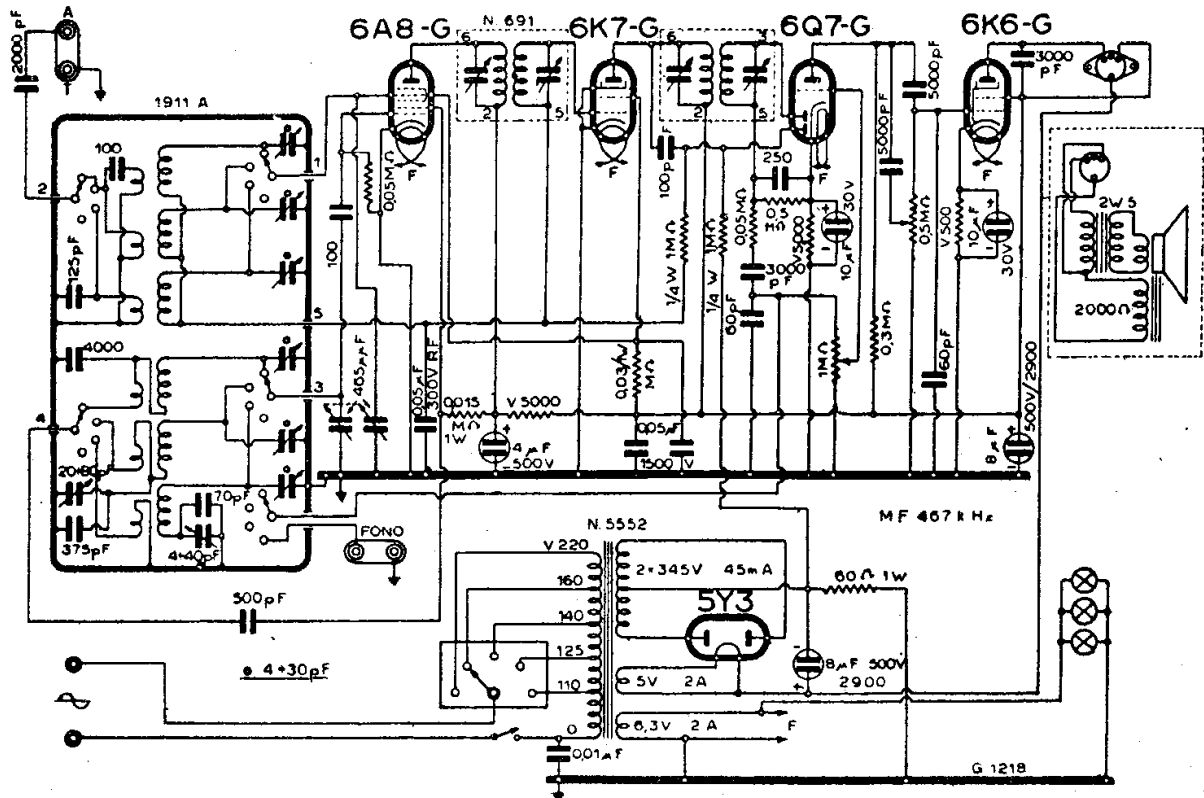
GELOSO (SOC.) - MOD. SUPER « G 50 R »
