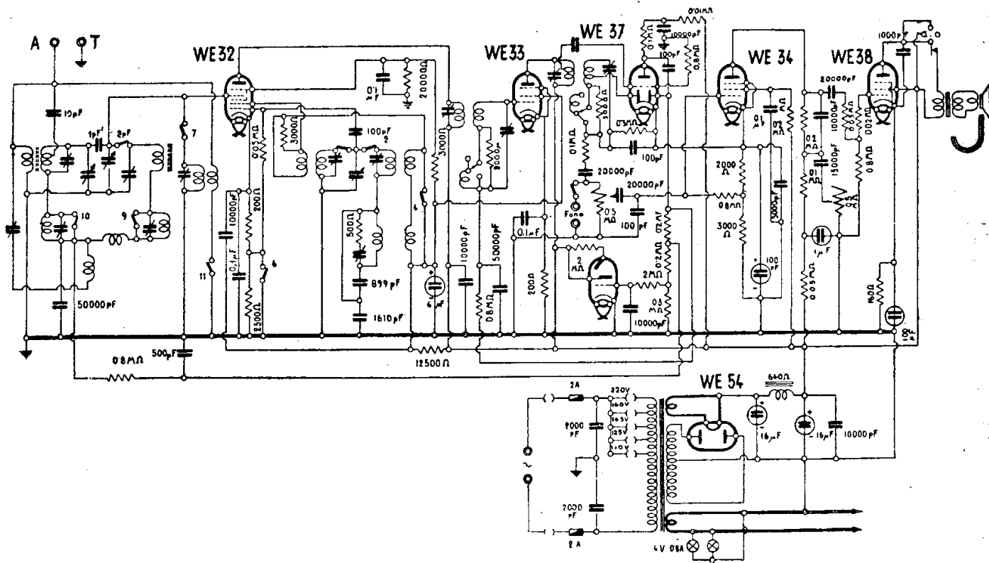
MINERVA - MOD. « 376 - 1 PH »
