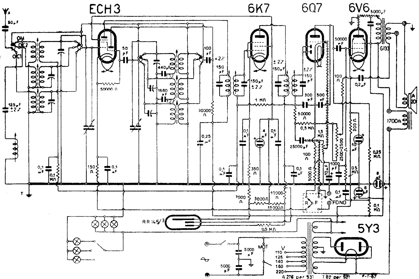
ALLOCCIO, BACCHINI & C. - MODD. « 521 », « 531 », « 534 »
