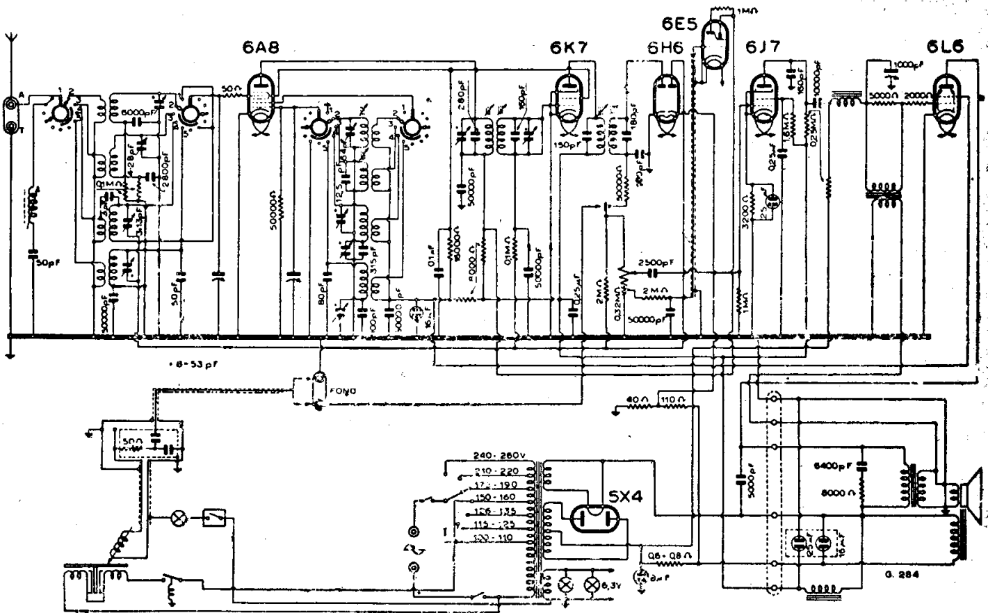
RADIOMARELLI - MOD. « ASSAB » FONDO
