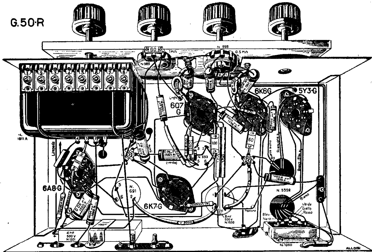
Il piano costruttivo del « G 50 R ».
