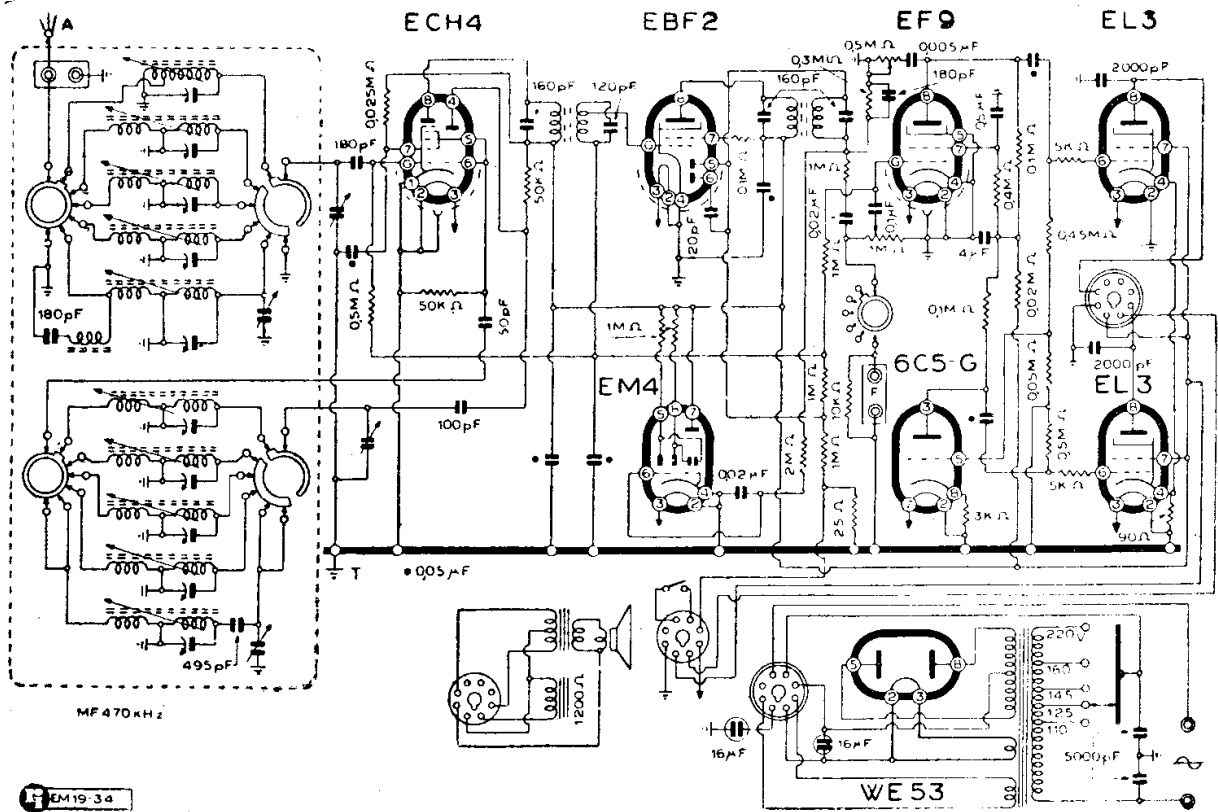
MINERVA - MOD. « 477/1 »
