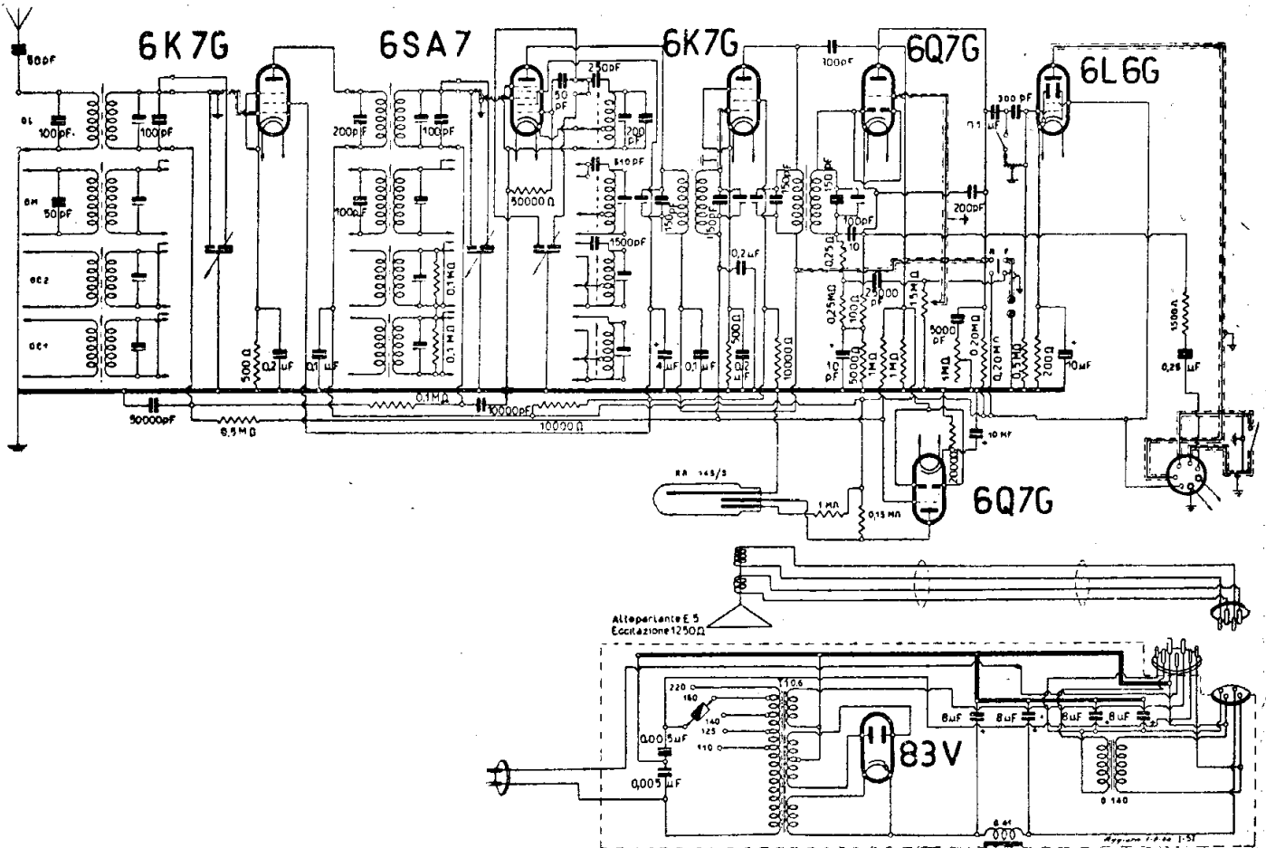
ALLOCCIO, BACCHINI & C. MOD. « 710 »
