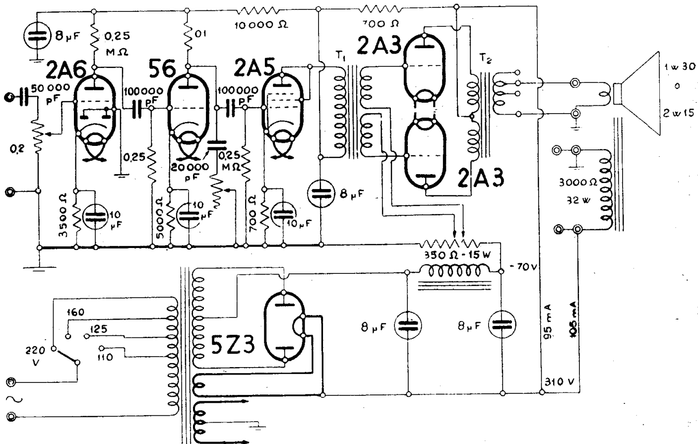
INDUSTRIALE RADIO - AMPLIFICATORE « I R 6 A 20 »
