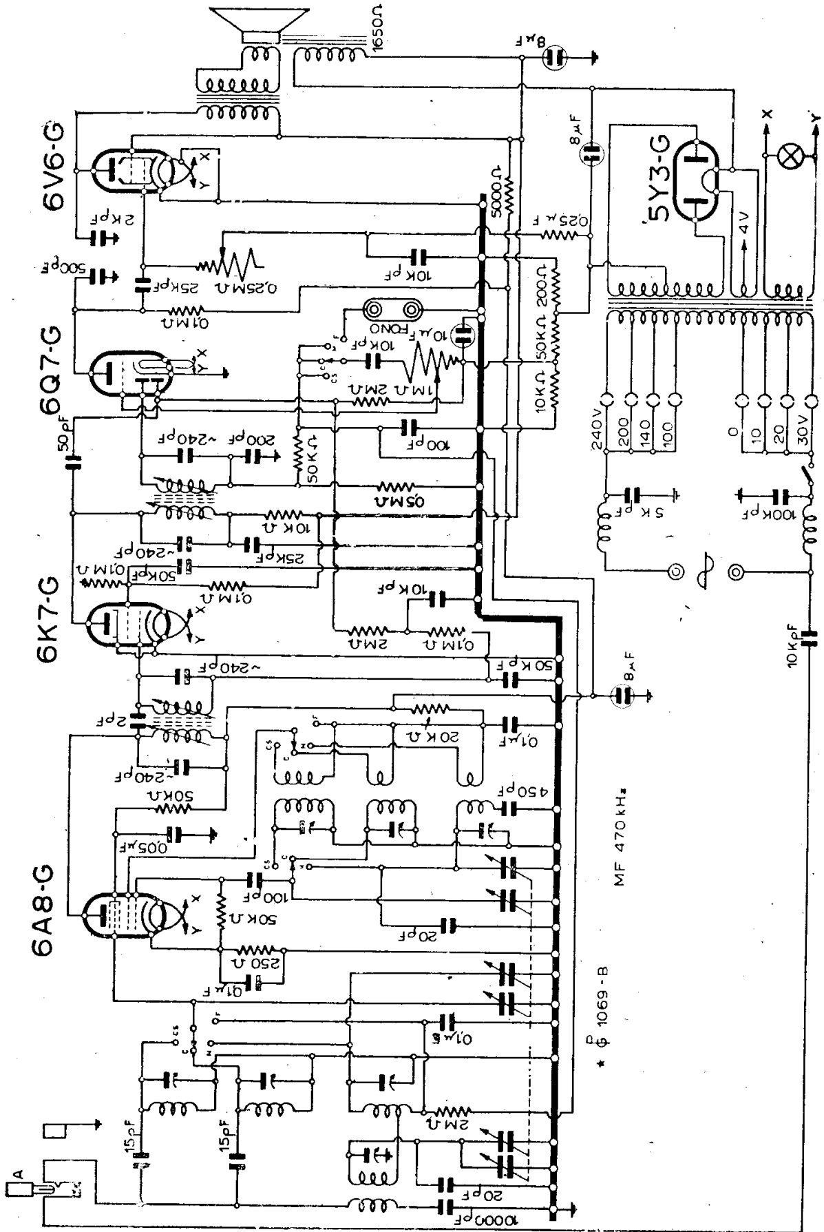
F.I.M.I. - MOD. PHONOLA « 561 B »
