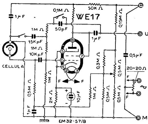
SIEMENS S. A. - PREAMPLIFICATORE MOD. « C 499 »
