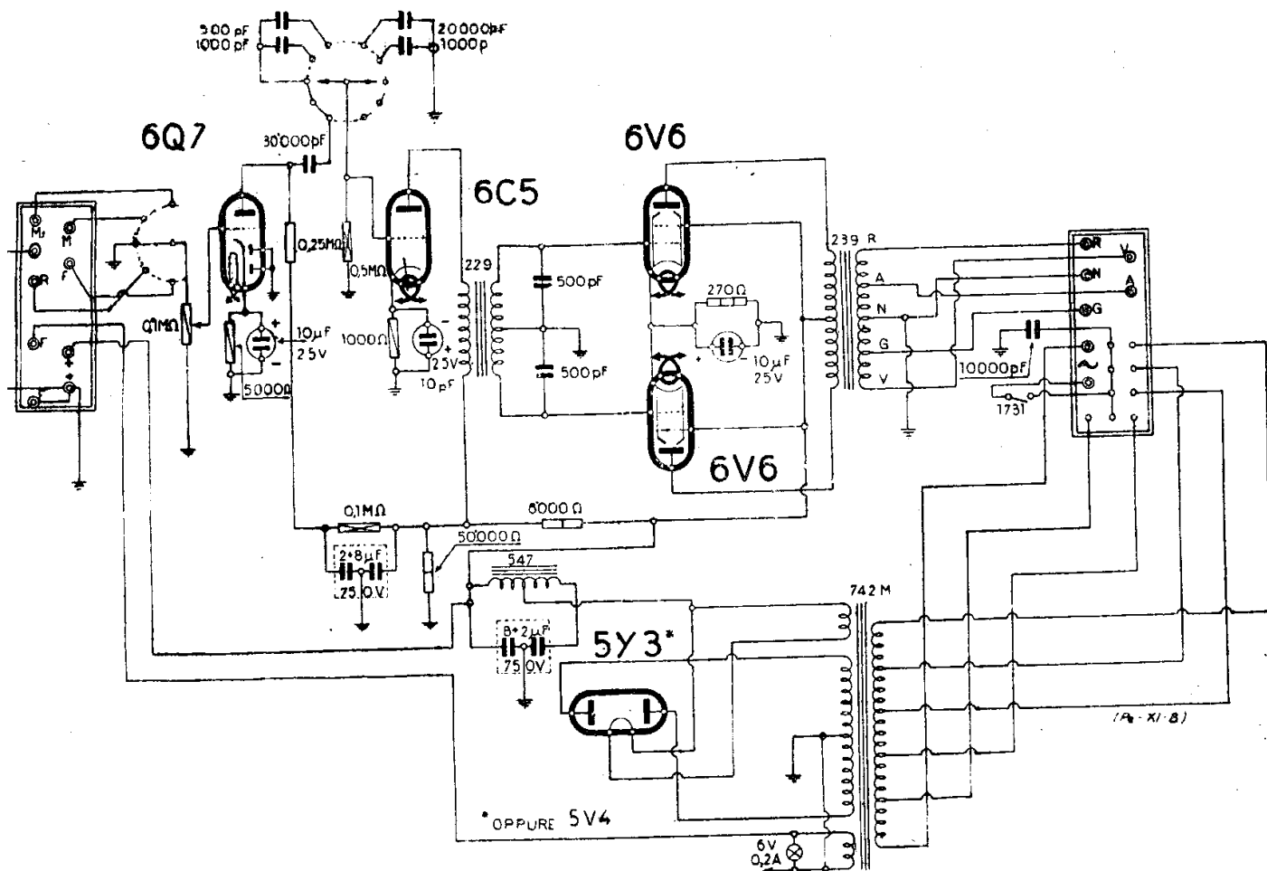
GALLO ING. G. - AMPLIFICATORE CONDOR - MOD. « 15 A5 »
