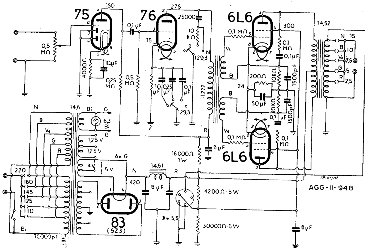
NOVA - AMPLIFICATORE MOD. « 24-30 W » - Nuova Serie
