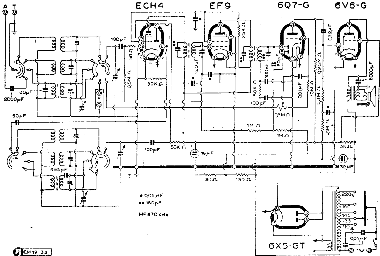
MINERVA - MOD. « 475/5 »
