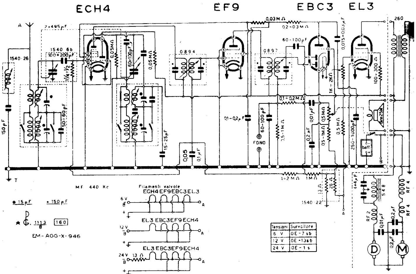
GALLO ING. G. - CONDOR MOD. « GIBLI II° »
