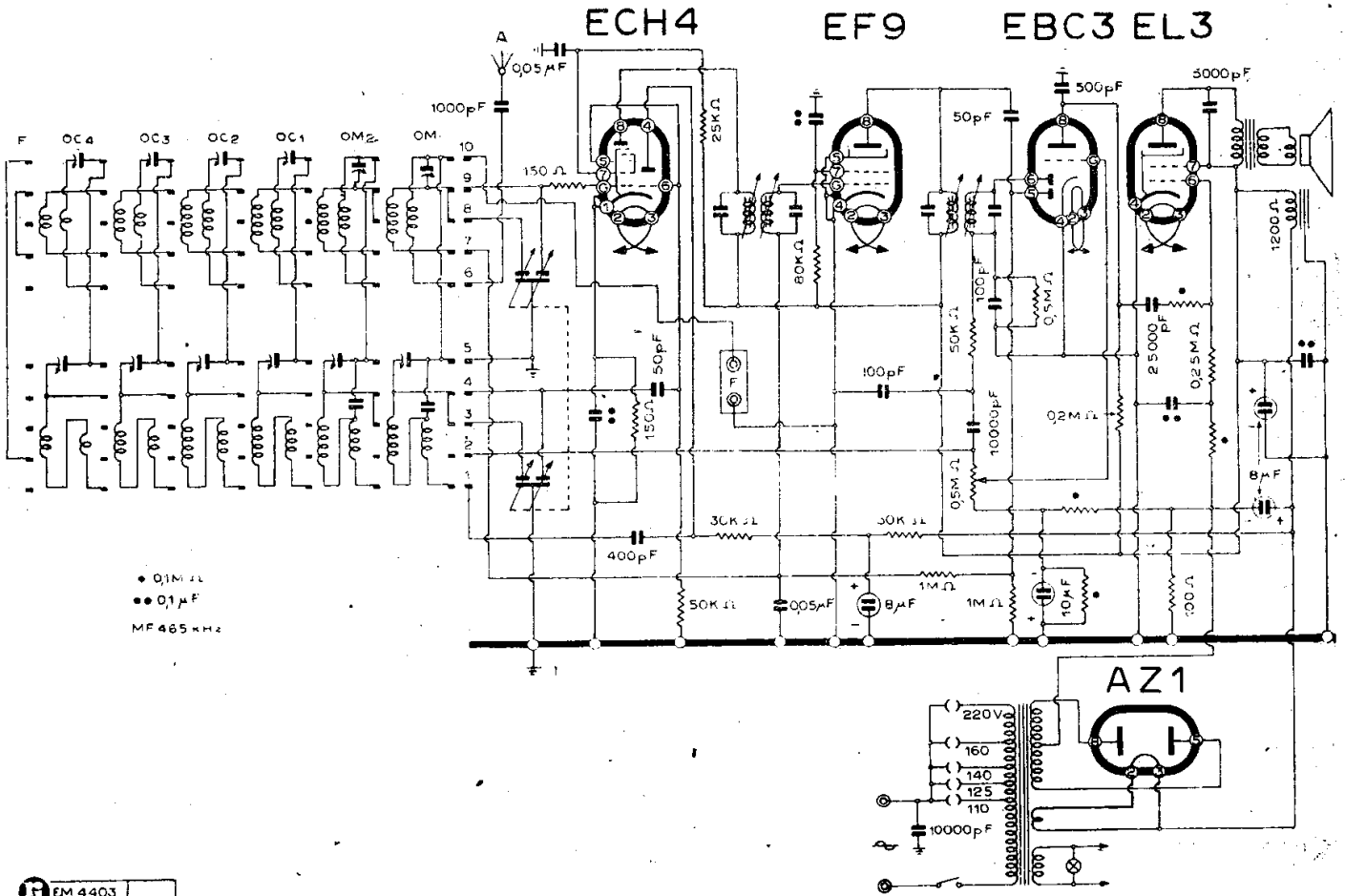
INCAR - MOD. « LV 49 »
