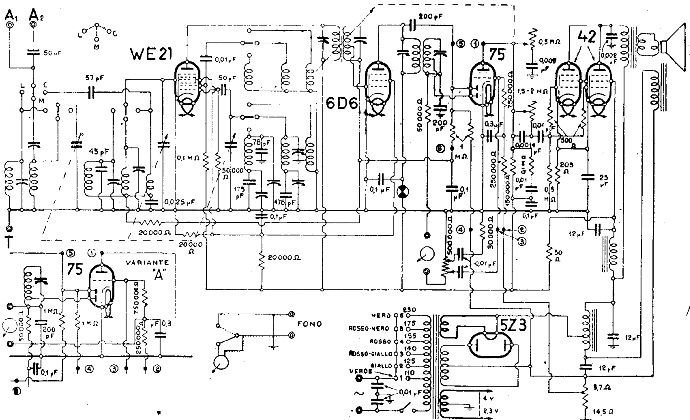
MAGNADYNE - MOD. « SV 15 C »
