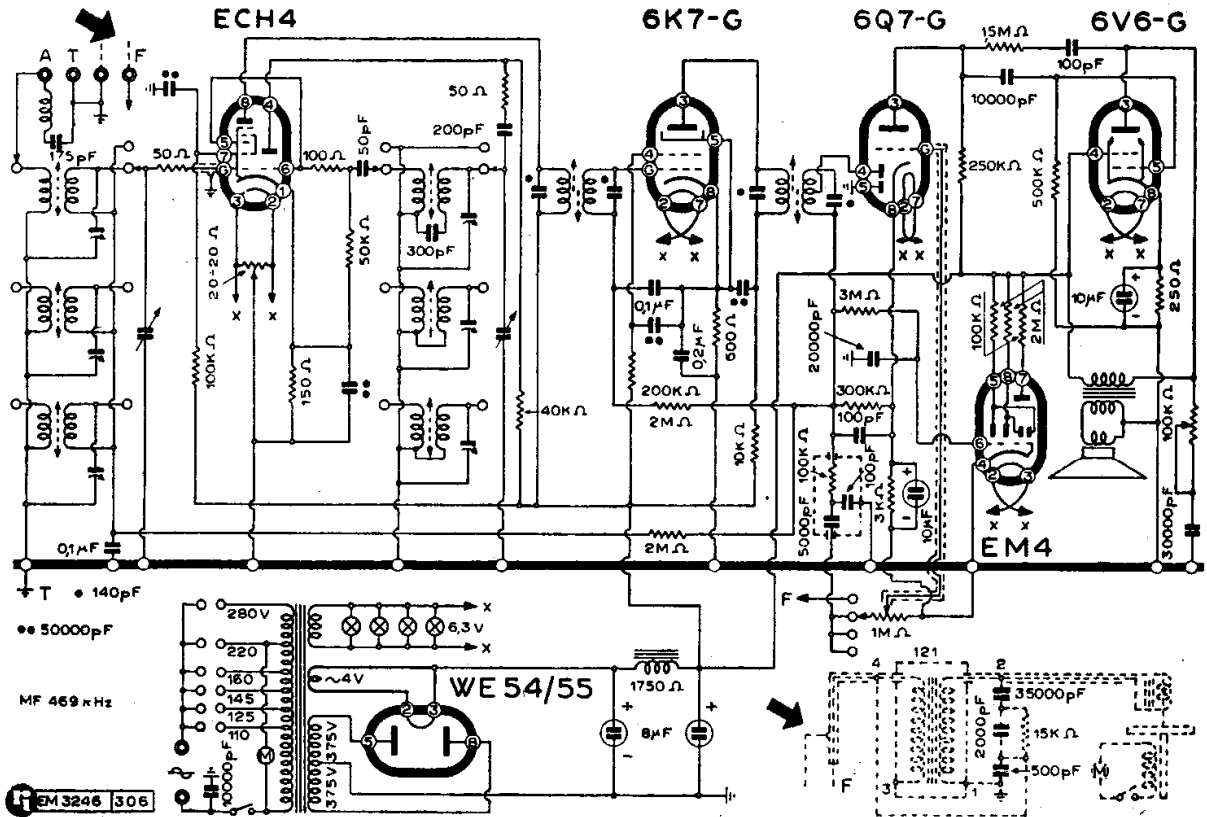
SIEMENS S. A. - MODD. « S 536 » « S 541 RF »
