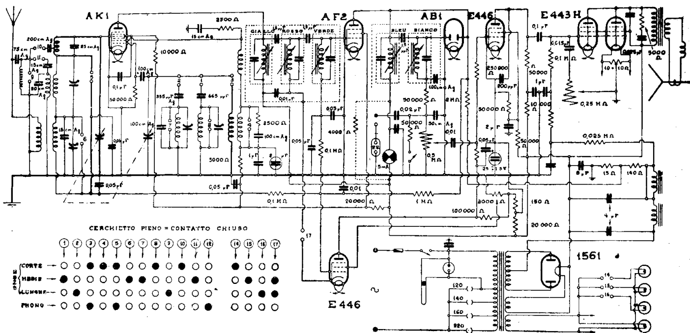
F.I.M.I. - MOD. PHONOLA « 700 »
