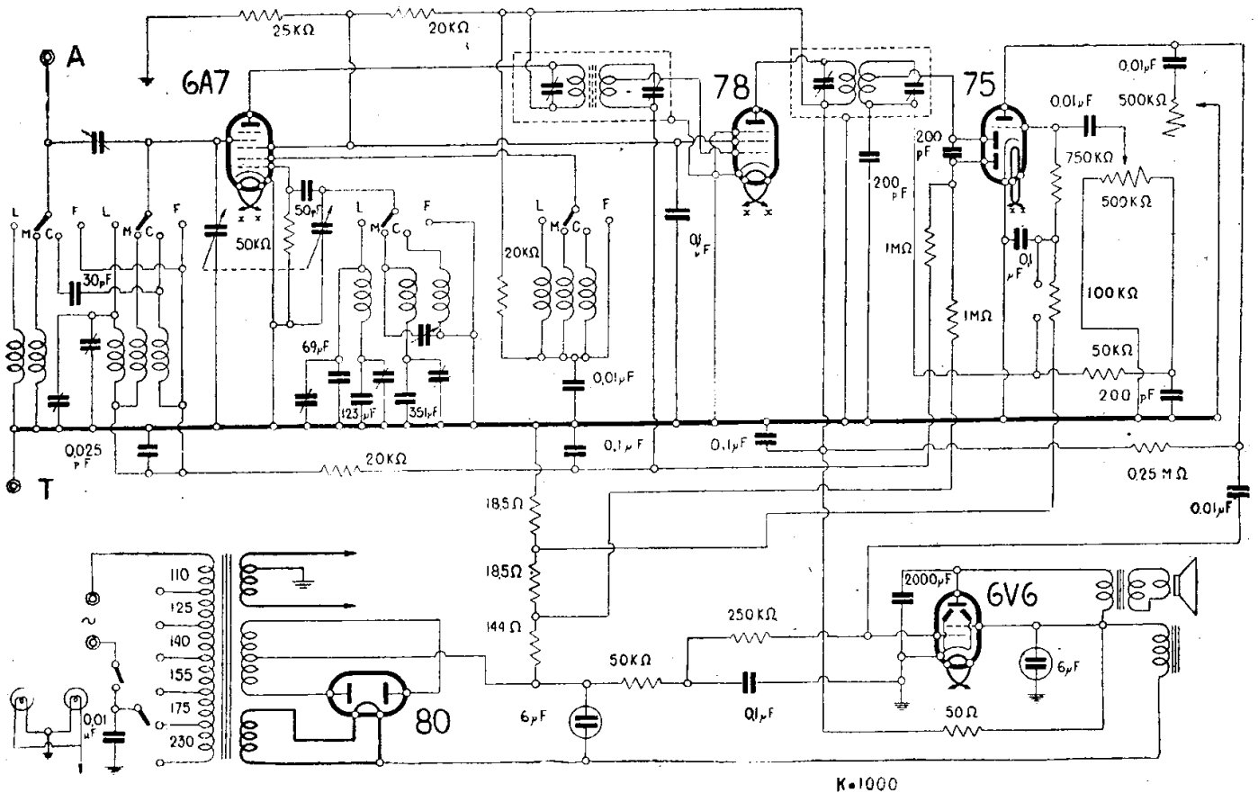
MAGNADYNE - MOD. « S 36 C »
