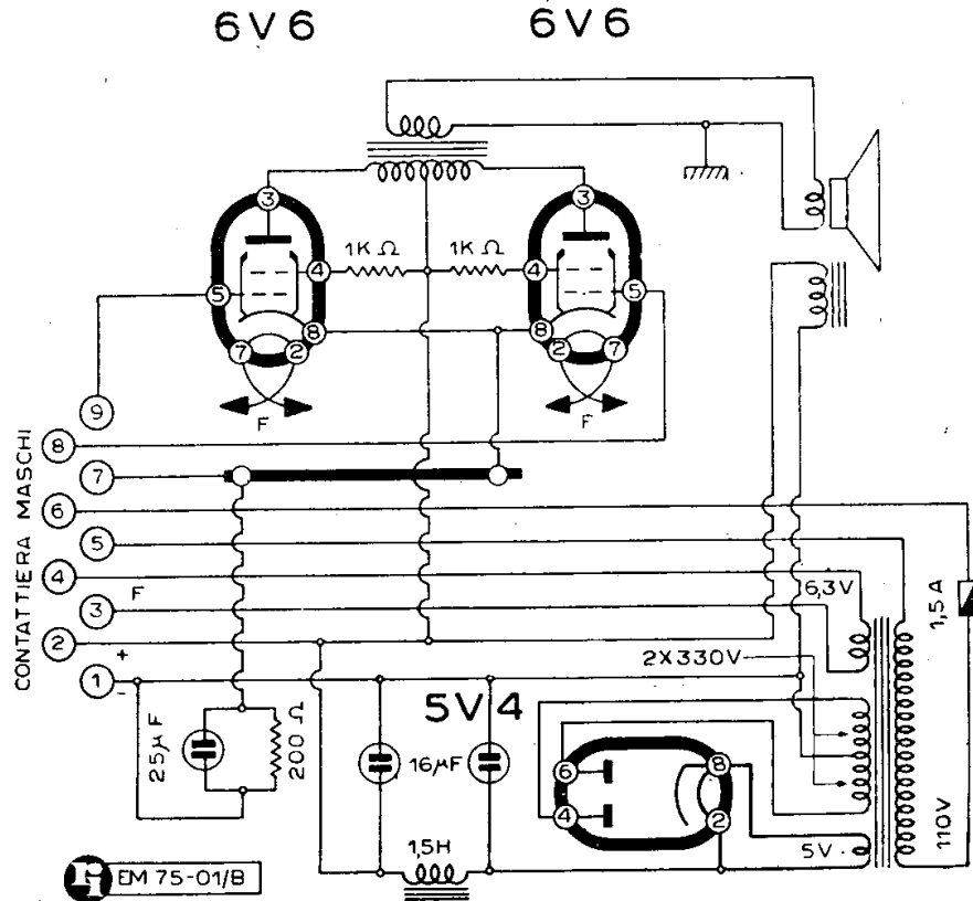
OMABI COMP. COSTR. CINEMATOGRAFICI - AMPLIFICATORE PER PROIETTORE MOD. « 3C/V/47 »
