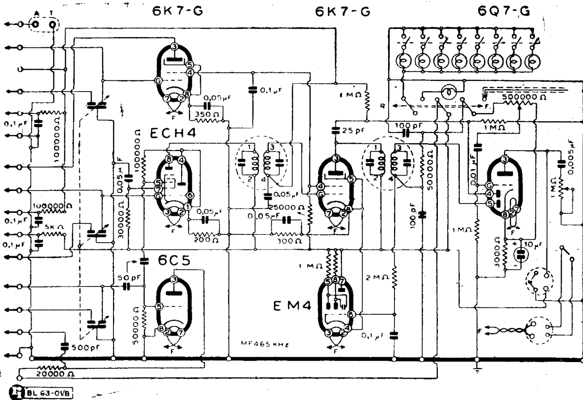
COMP. IT. MARCONI - MODD. « 1183 » « 1184 » PARTI AF-MF-RIV.
