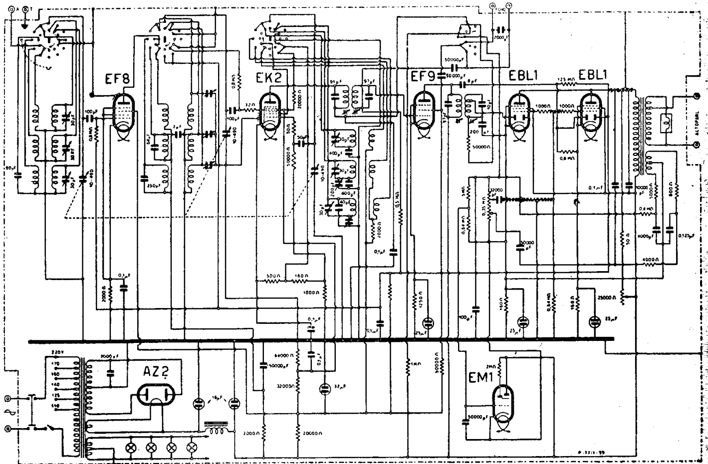
PHILIPS RADIO - MODD. « 755 M » « 788 RF »
