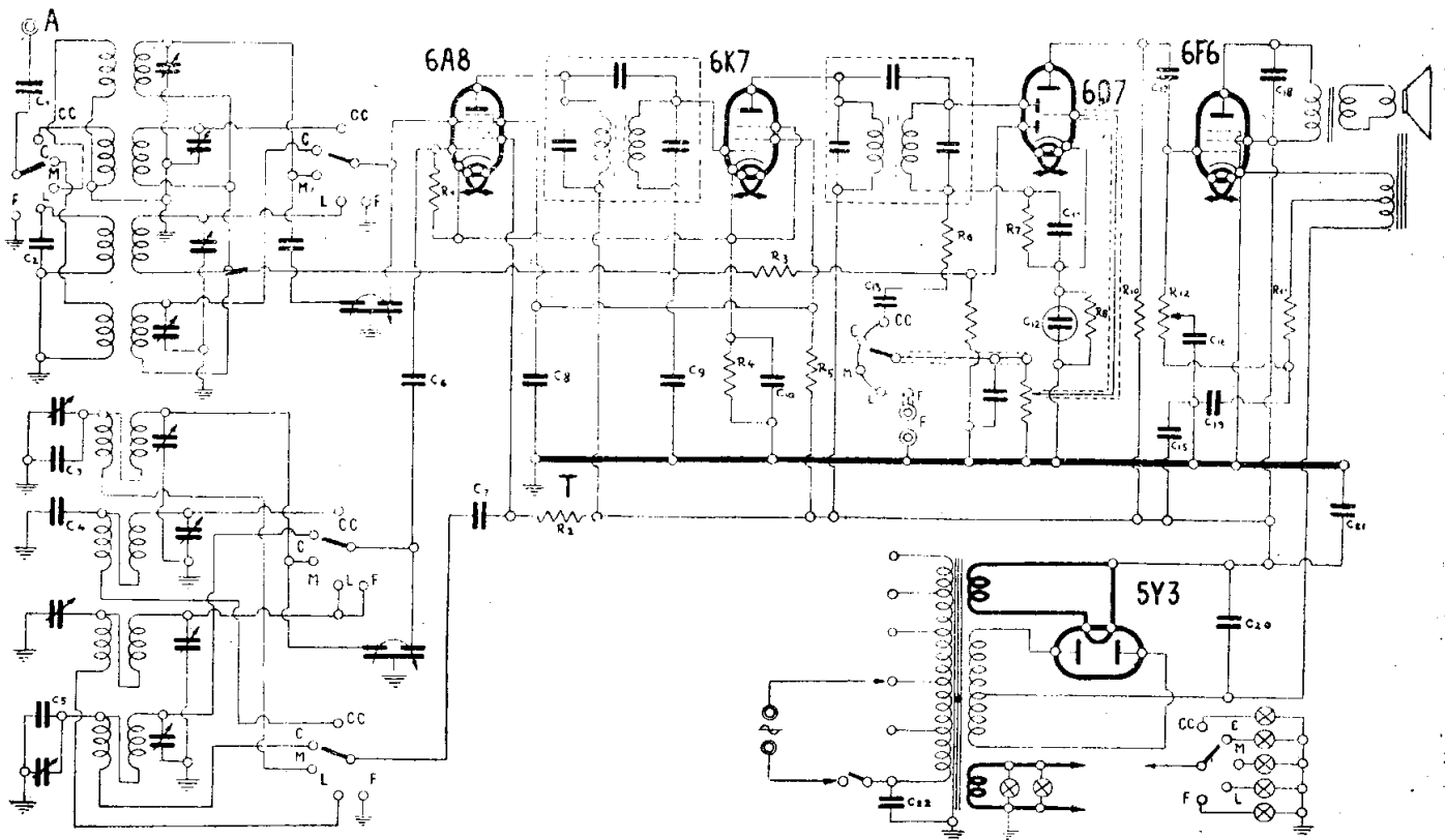
AREL - MOD. «IL MODELLO»
