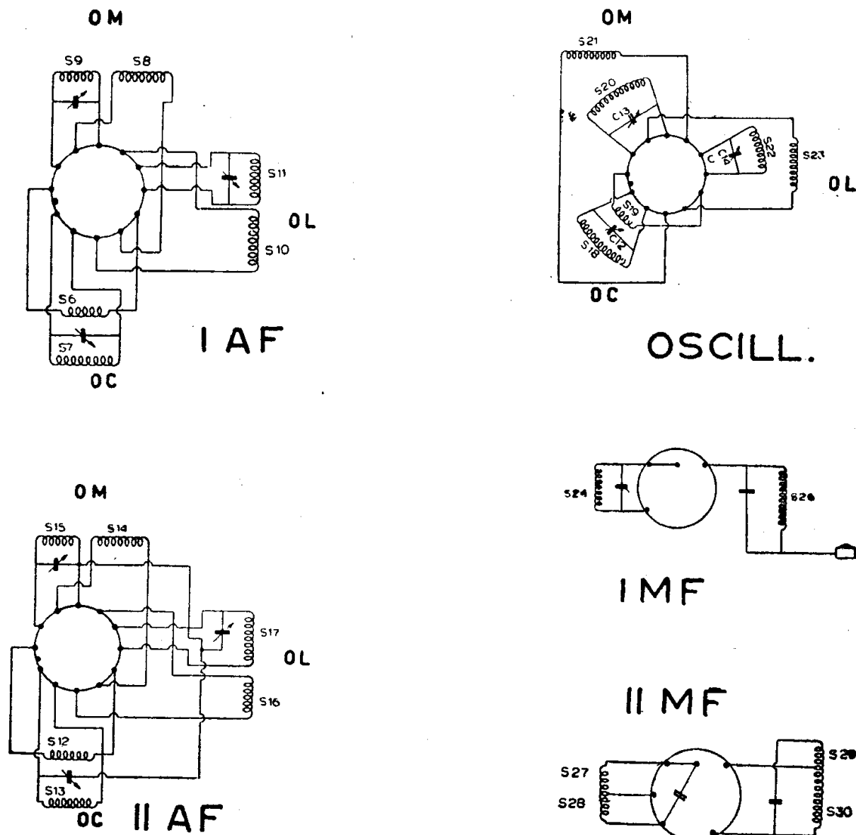
Le bobine e i relativi attacchi dei modelli « 678 » e « 682 ».
