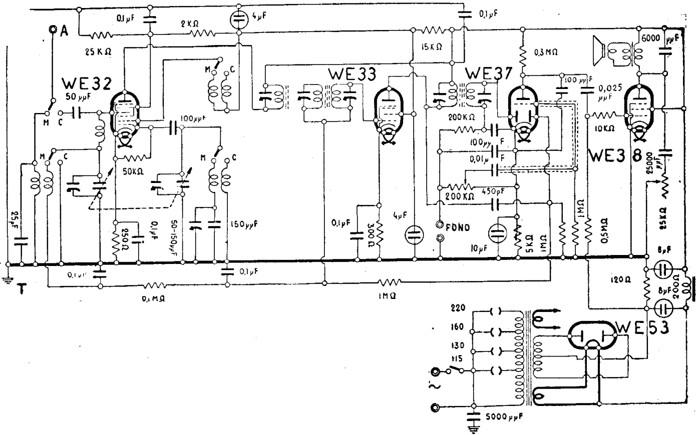
RADIO LAMBDA - MOD. « E 245 »
