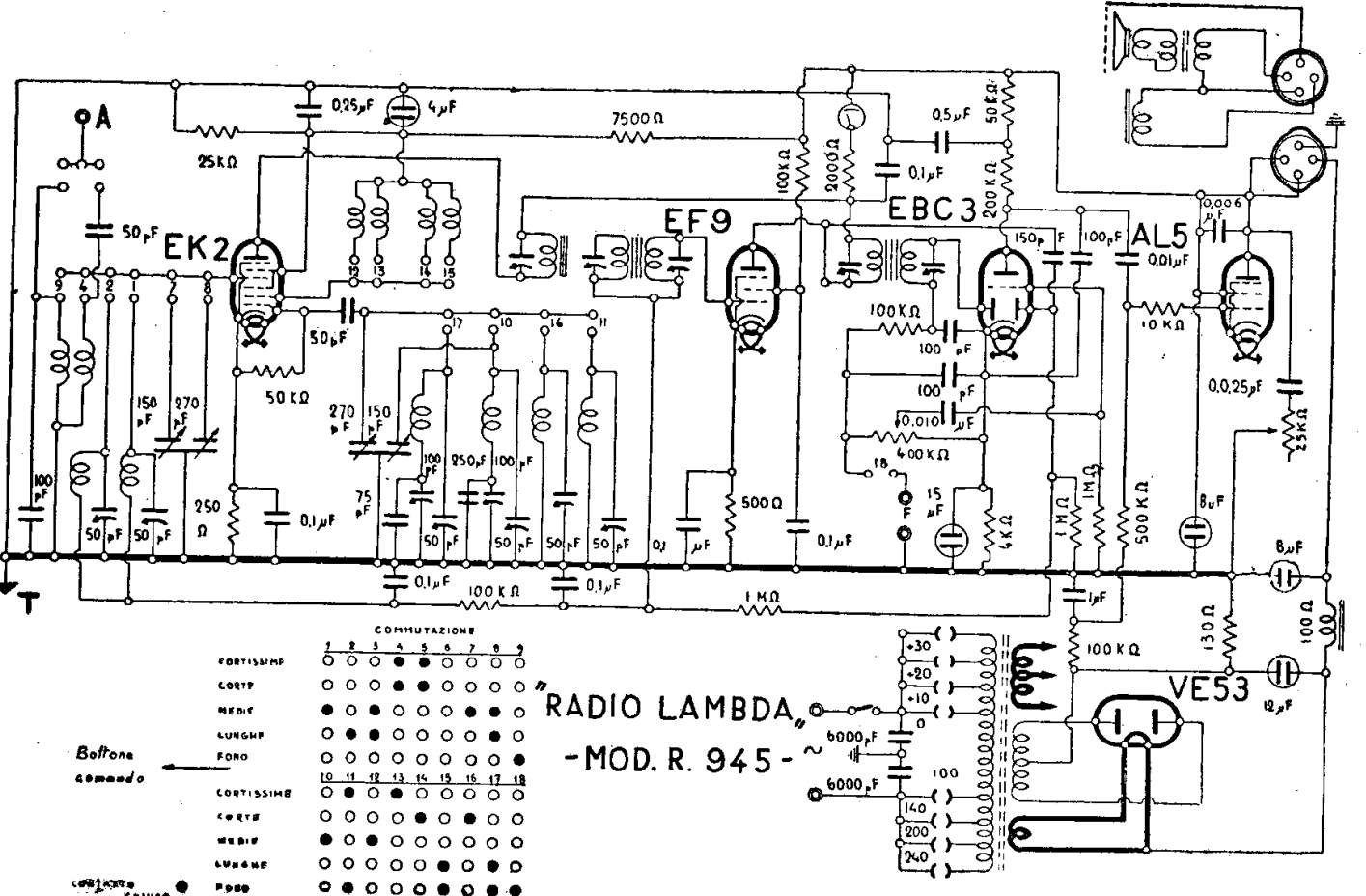
RADIO LAMBDA - MOD. « R 945 »
