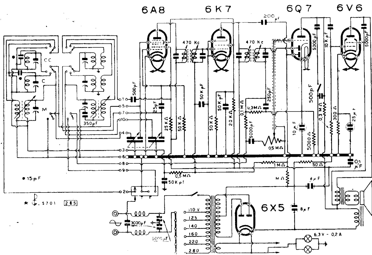
I.R.I.M. - MOD. « 653 »
