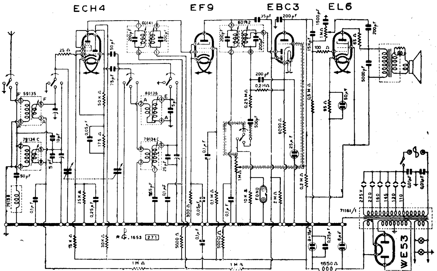
LA VOCE DEL PADRONE - COLUMBIA - MARCONIPHONE MOD. « V. d. P. 580 »
