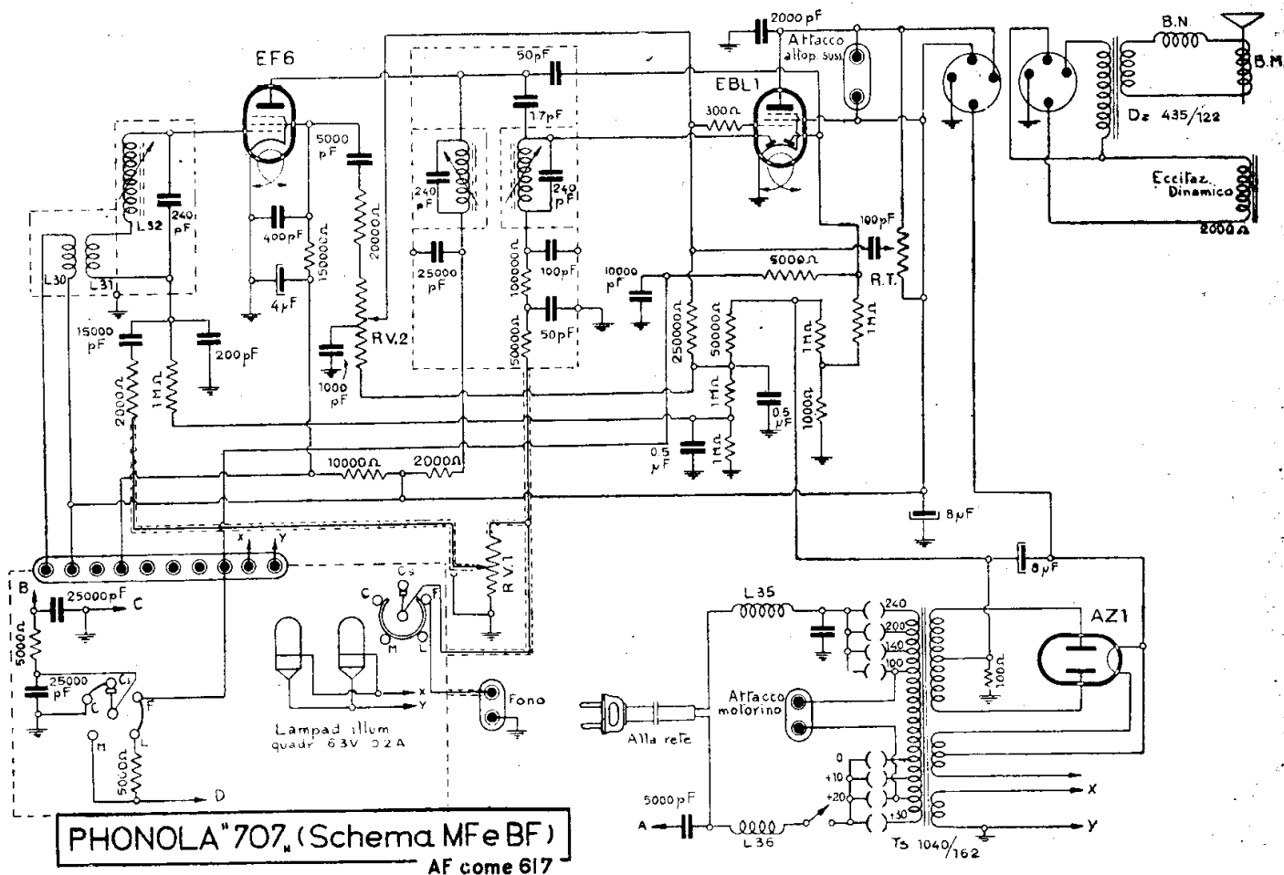
F.I.M.I. - MODD. PHONOLA « 707 » « 708 » « 709 » PARTI MF-BF (AF DEL 617)
