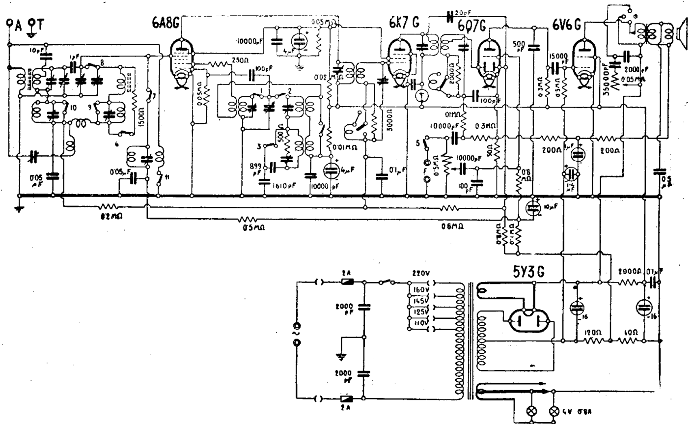
MINERVA . MOD. « 375 - SF »
