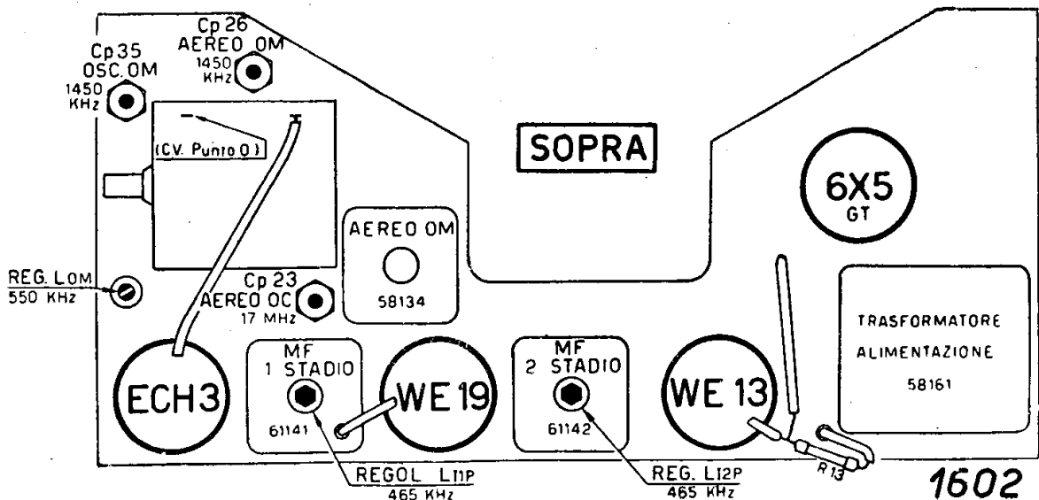
Il telaio del mod. « V.d.P. 458 » visto da sopra.
