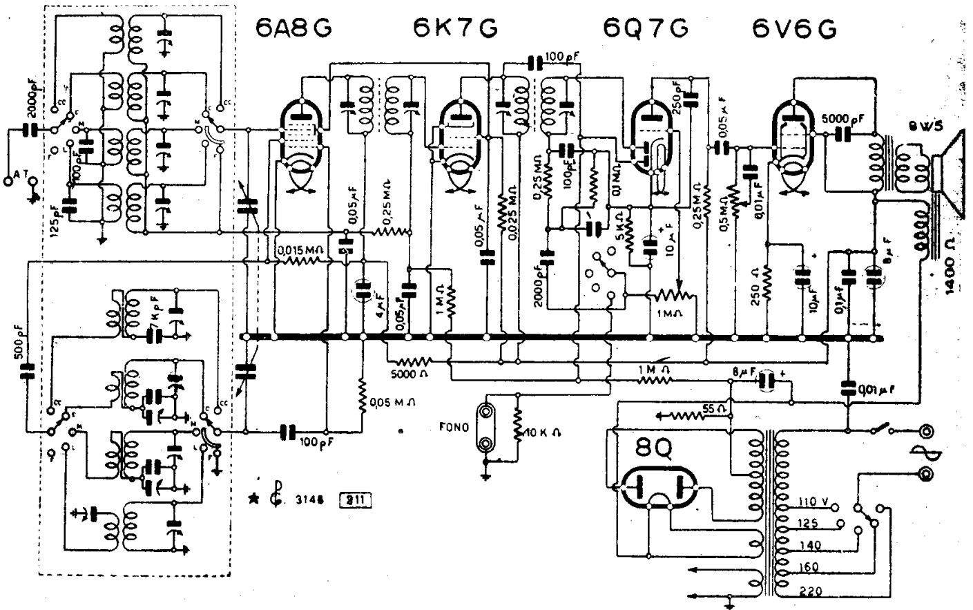
S.I.A.R.E. - MOD. « 411 »
