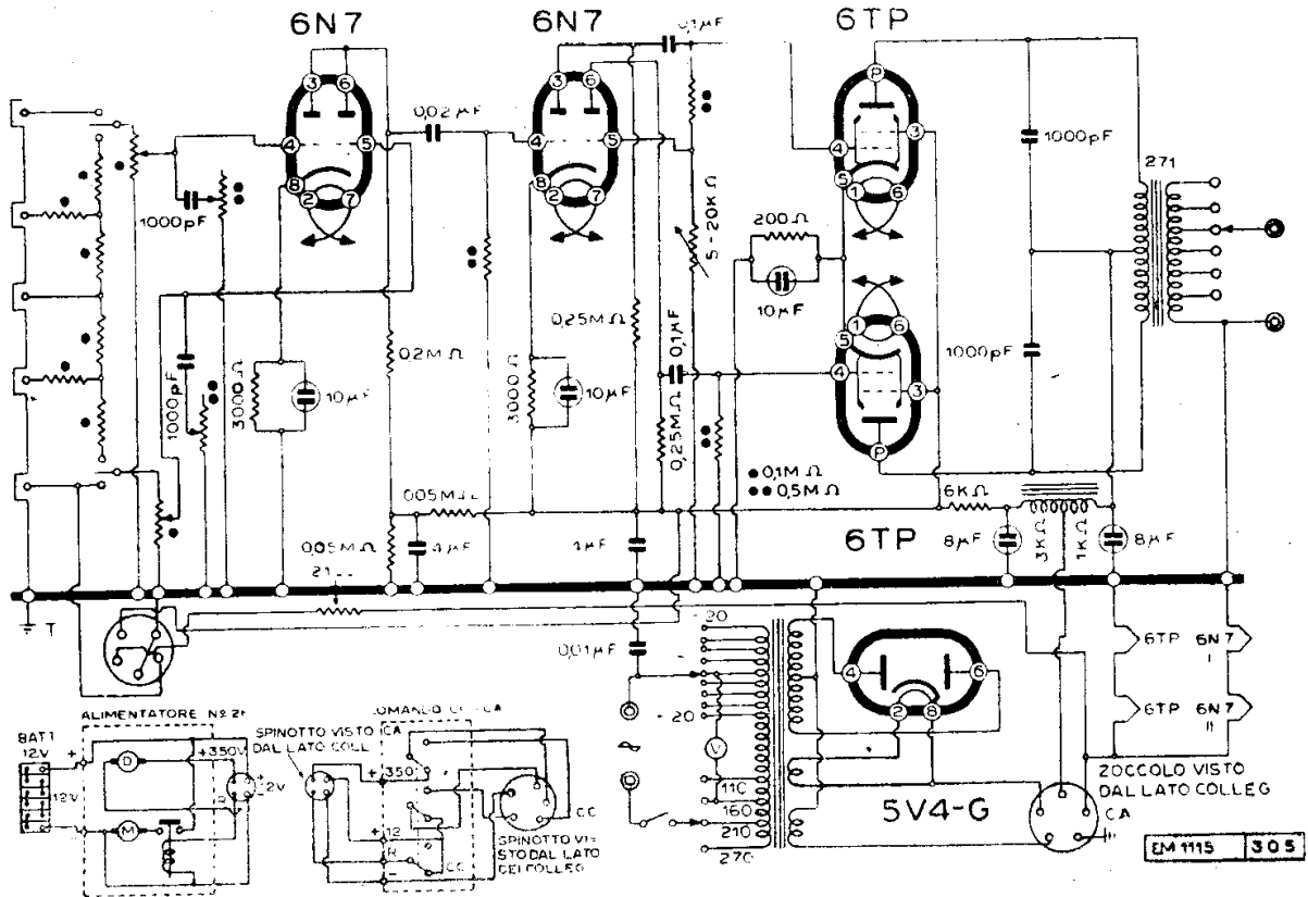
GALLO ING. G. - AMPLIFICATORE CONDOR - MOD. « M 20 ».
