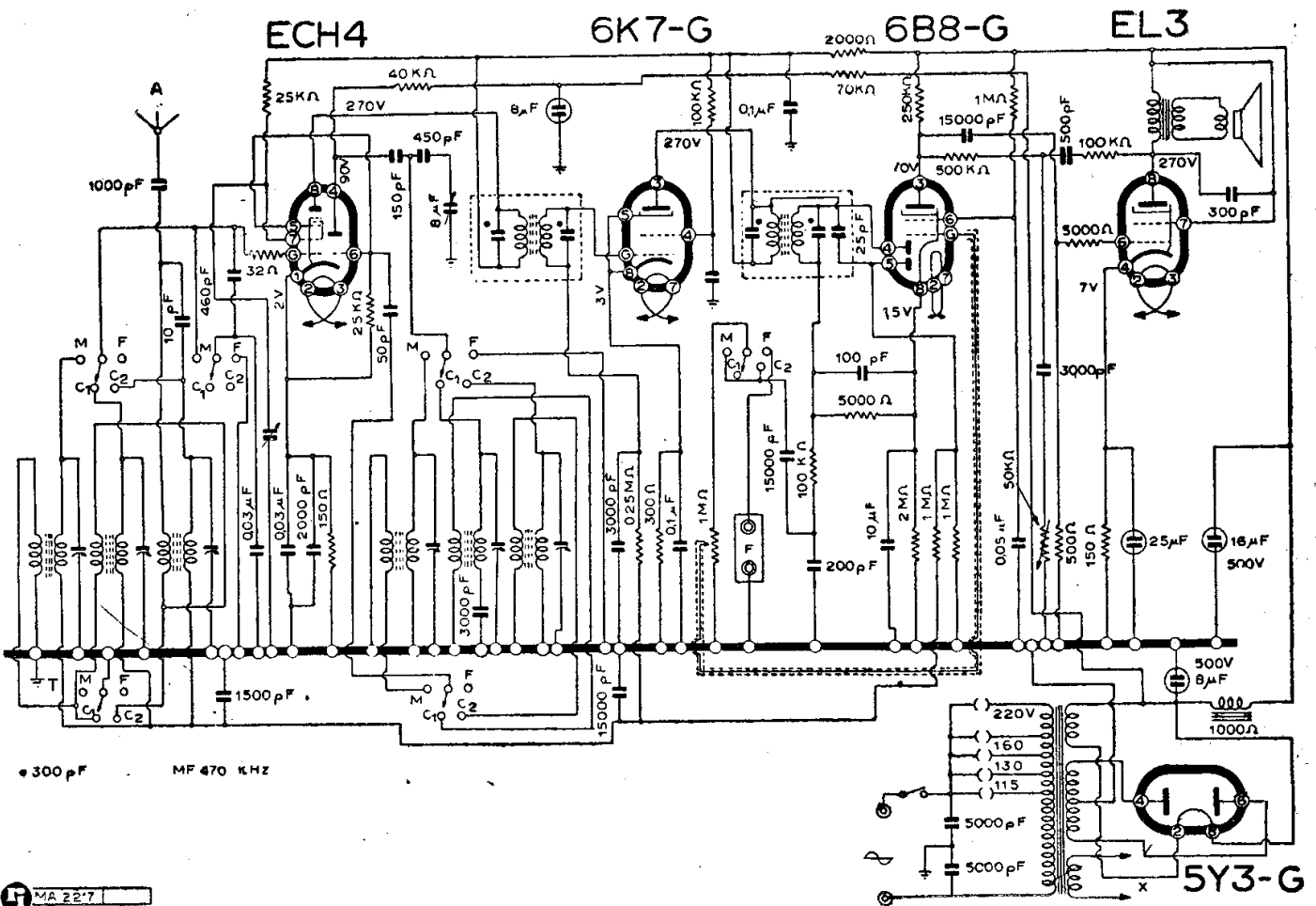
RADIO LAMBDA - MOD. « GL 355-M »
