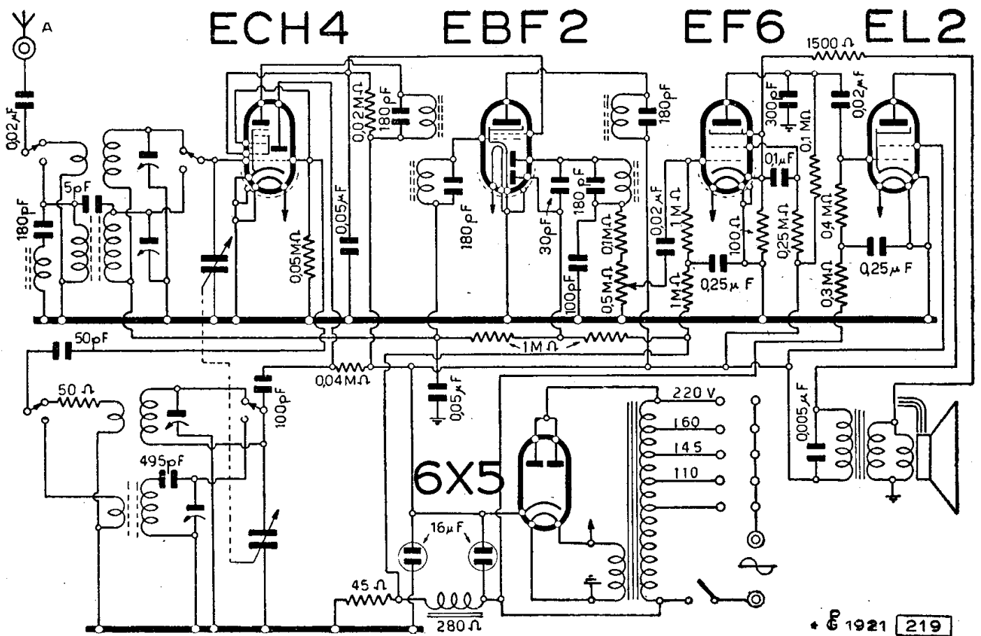
MINERVA - MOD. « 455/1 »
