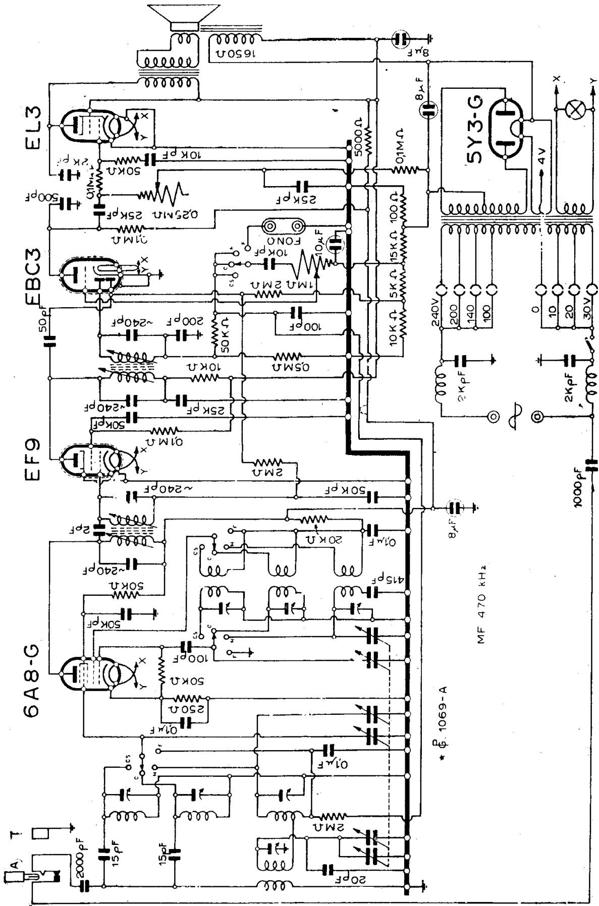
F.I.M.I. - MODD. PHONOLA « 561 A » - « 562 A »
