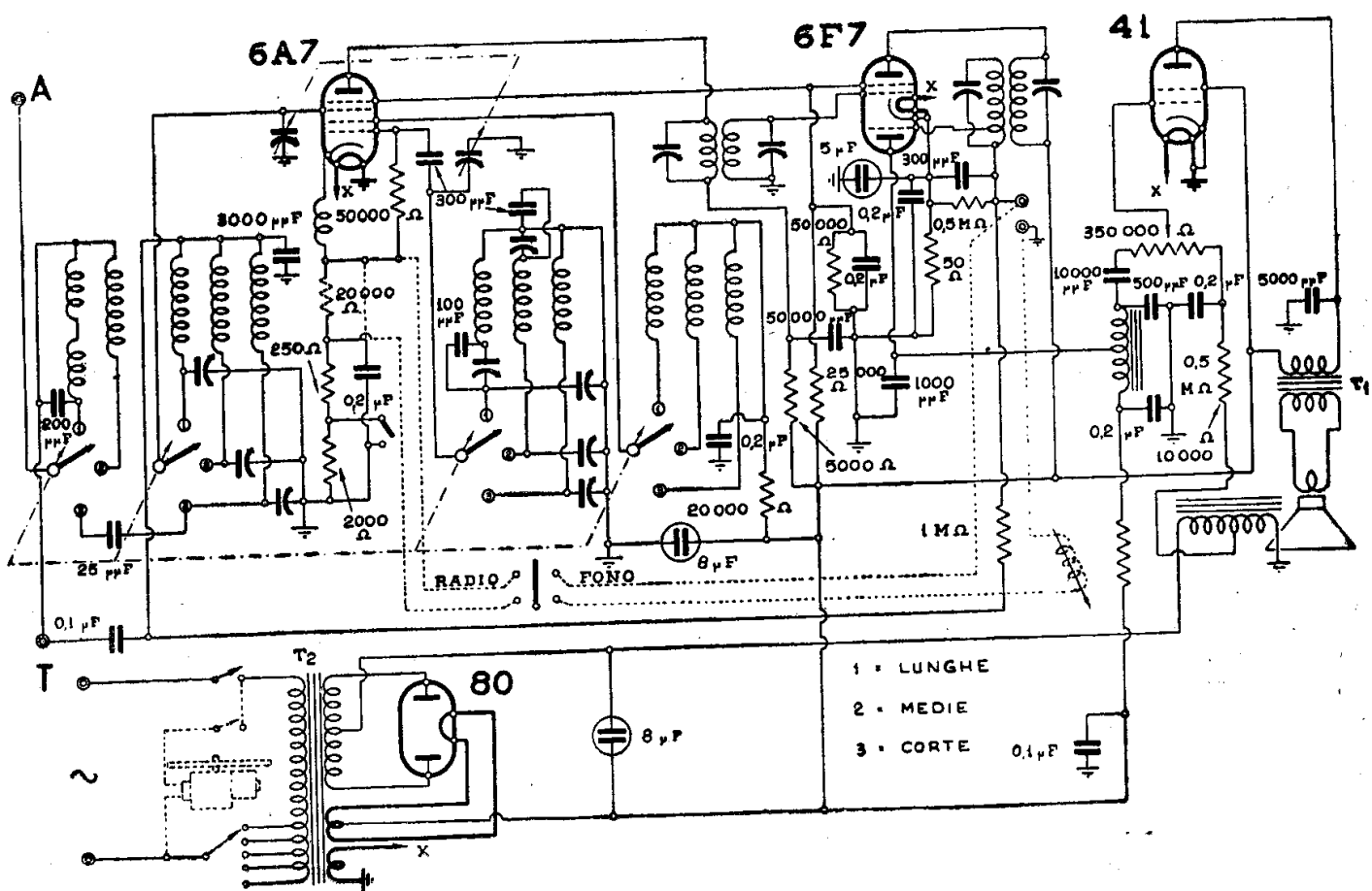
S.A.F.A.R. - MOD. « 43 »
